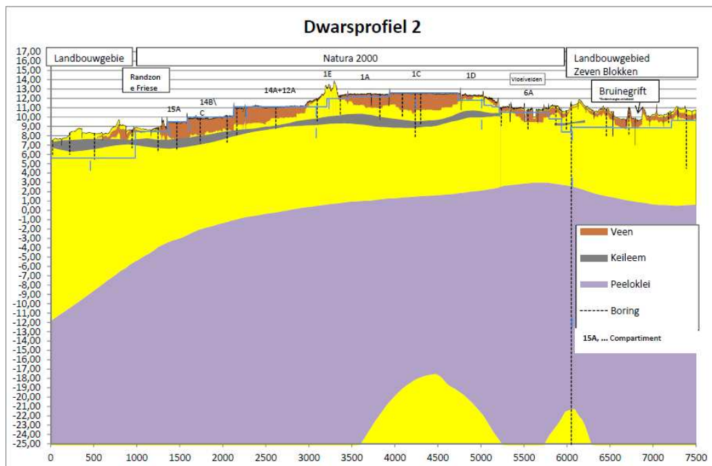
Figuur 3-3 De bodemopbouw in een west-oost-raai.
