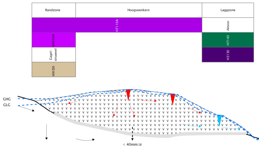
5 Figuur 3-1 Schematische doorsnede van de werking van een hoogveengebied (Gradiëntdocument: Everts, et al.). In het Fochteloërveen is een afgeleide situatie aanwezig met nauwelijks nog een acrotelm (bovenste intacte veenlaag) en over het algemeen (veel) meer wegzijging dan 40 mm per jaar (In: Rijpkema et al., 2013) Daarnaast ontbreekt een natuurlijke rand- en laggzone.
