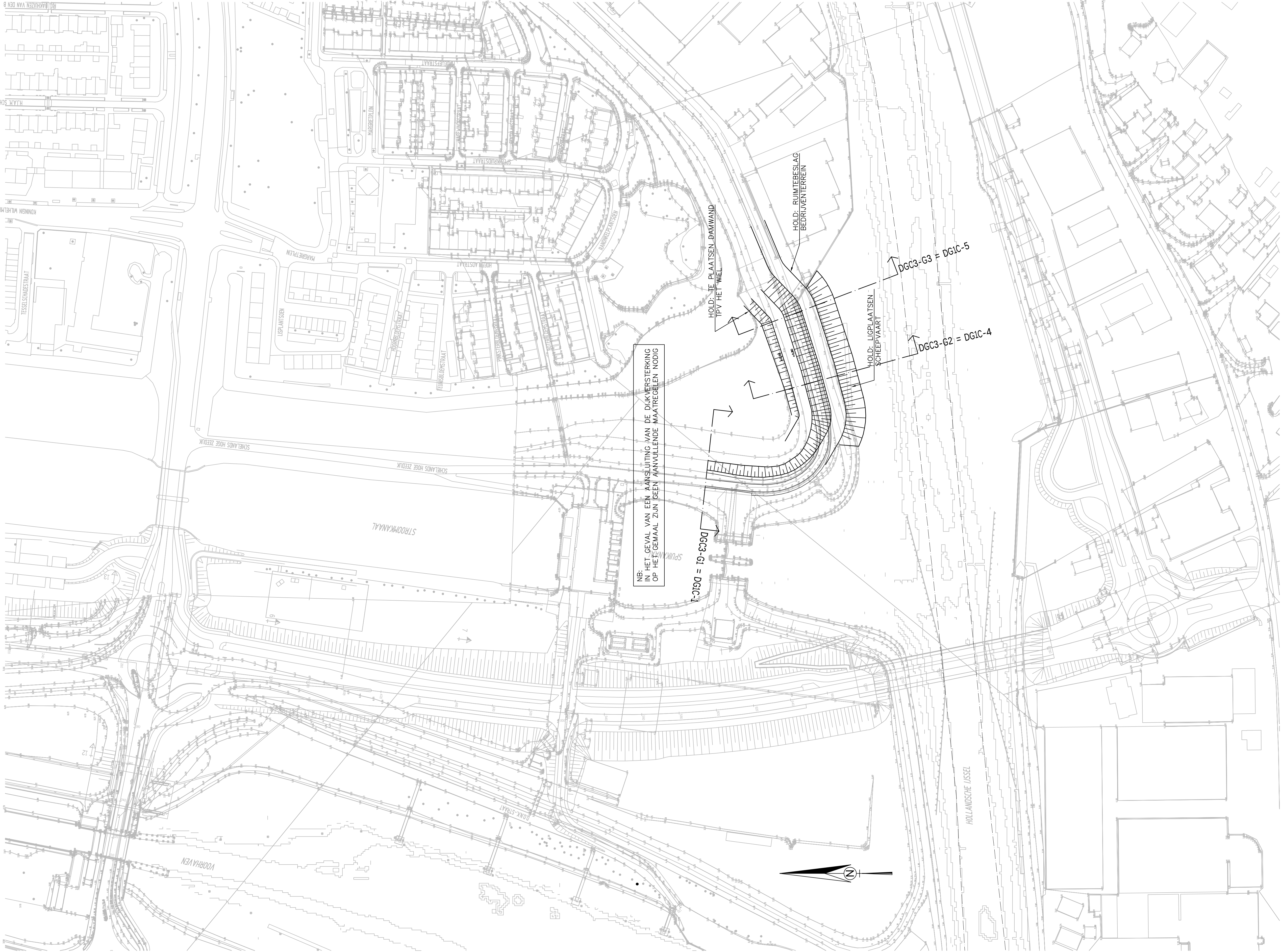
BOVENAANZICHT VARIANT C3 SCHAAL 1:1000
