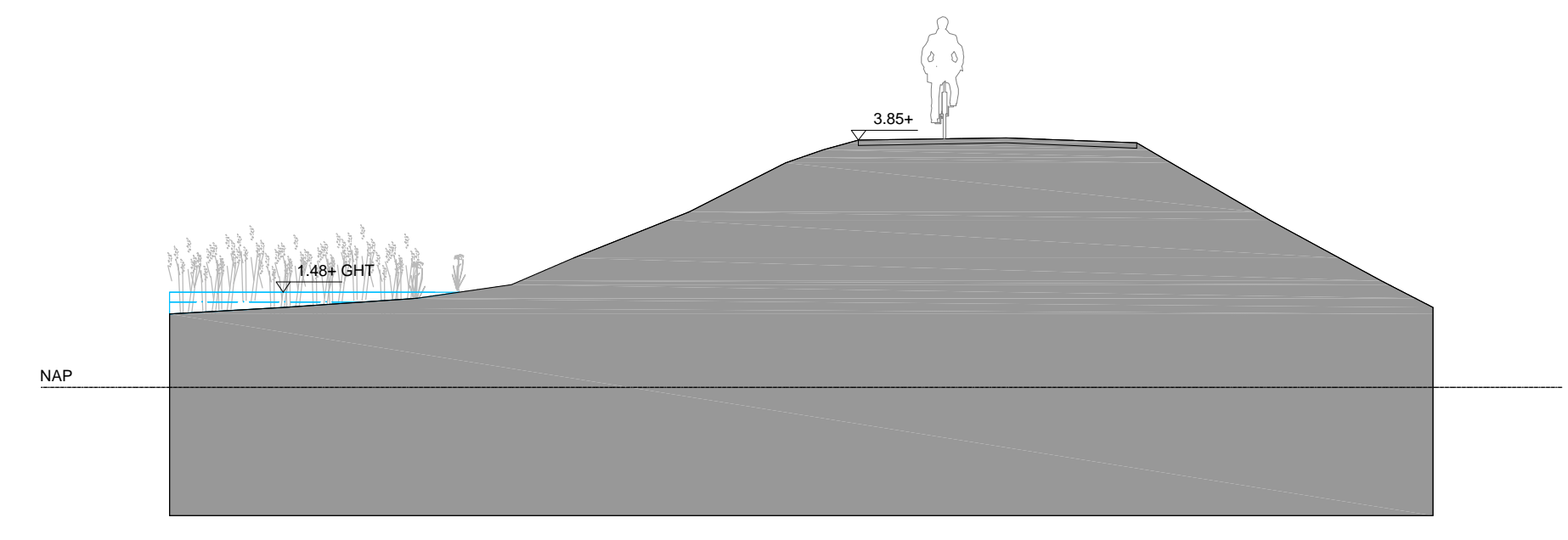
Doorsnede G-G', schaal 1:100
