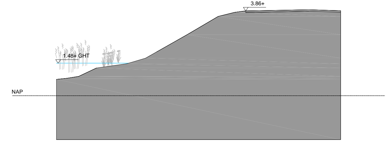
Doorsnede F-F, schaal 1:100
