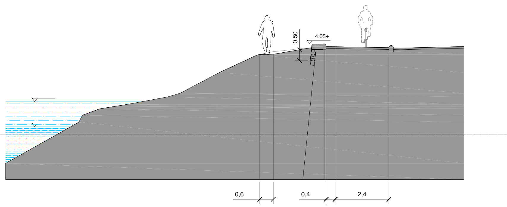
Doorsnede E-E' beëindiging van de muur ten oosten van de Haastrechtsebrug, schaal 1:100
