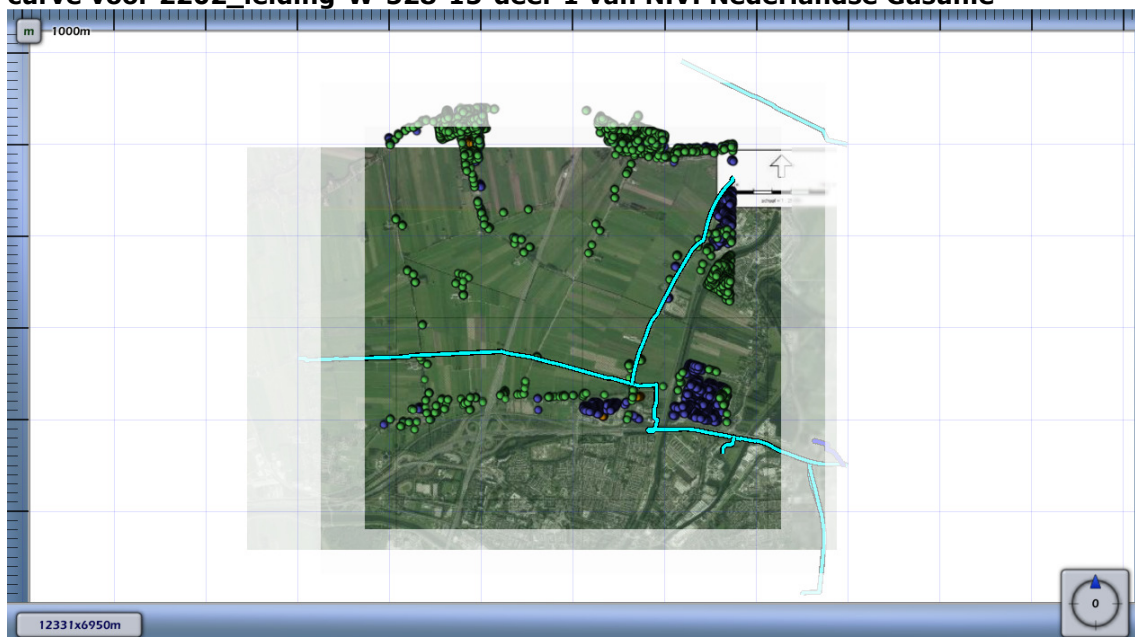
Figuur 4.6 Kilometer leiding behorende bij de maximale overschrijding van de FN-curve voor 2202_leiding-W-528-15-deel-1 van N.V. Nederlandse Gasunie
