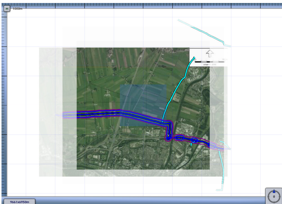
3.2 Figuur 3.2 Plaatsgebonden risico voor 2202_leiding-W-528-01-deel-1 van N.V. Nederlandse Gasunie
