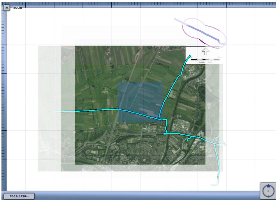
3.2 Figuur 3.2 Plaatsgebonden risico voor 2202_leiding-W-528-01-deel-1 van N.V. Nederlandse Gasunie
