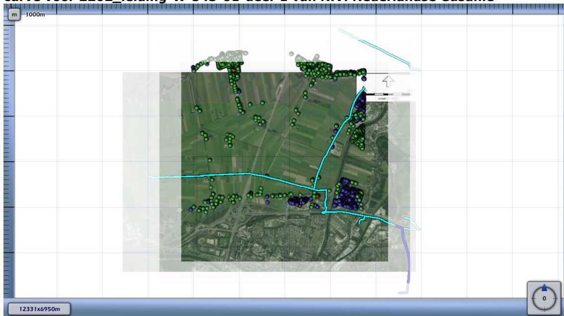
Figuur 4.7 Kilometer leiding behorende bij de maximale overschrijding van de FN-curve voor 2202_leiding-W-543-01-deel-1 van N.V. Nederlandse Gasunie
