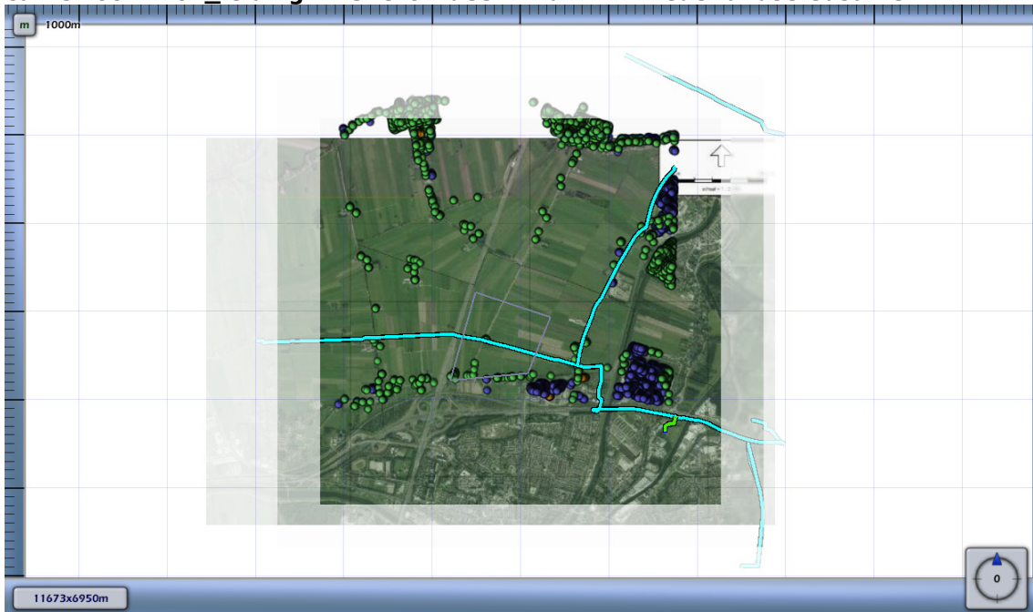
Figuur 4.5 Kilometer leiding behorende bij de maximale overschrijding van de FN-curve voor 2202_leiding-W-528-07-deel-1 van N.V. Nederlandse Gasunie
