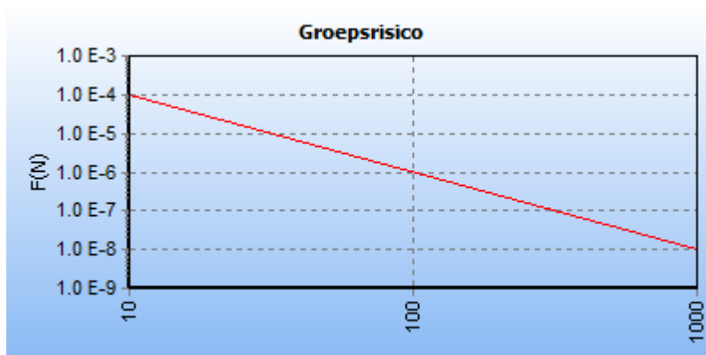
Figuur 2.6: fN -curve buisleiding W-528-01-deel-1 vóór planrealisatie
