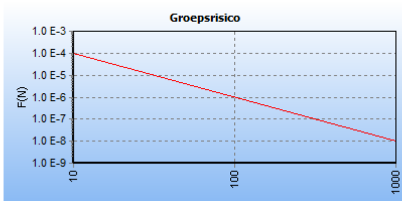
5.5 Figuur 5.5 FN curve voor 2202_leiding-W-528-07-deel-1 van N.V. Nederlandse Gasunie voor de kilometer tussen stationing 0.00 en stationing 260.00
