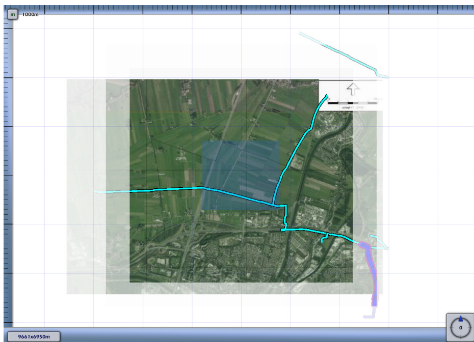
3.8 Figuur 3.8 Plaatsgebonden risico voor 2202_leiding-W-543-02-deel-1 van N.V. Nederlandse Gasunie
