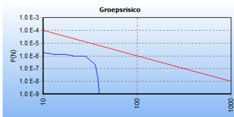
Figuur 2.7: fN-curve buisleiding W-528-01-deel-1 ná planrealisatie
