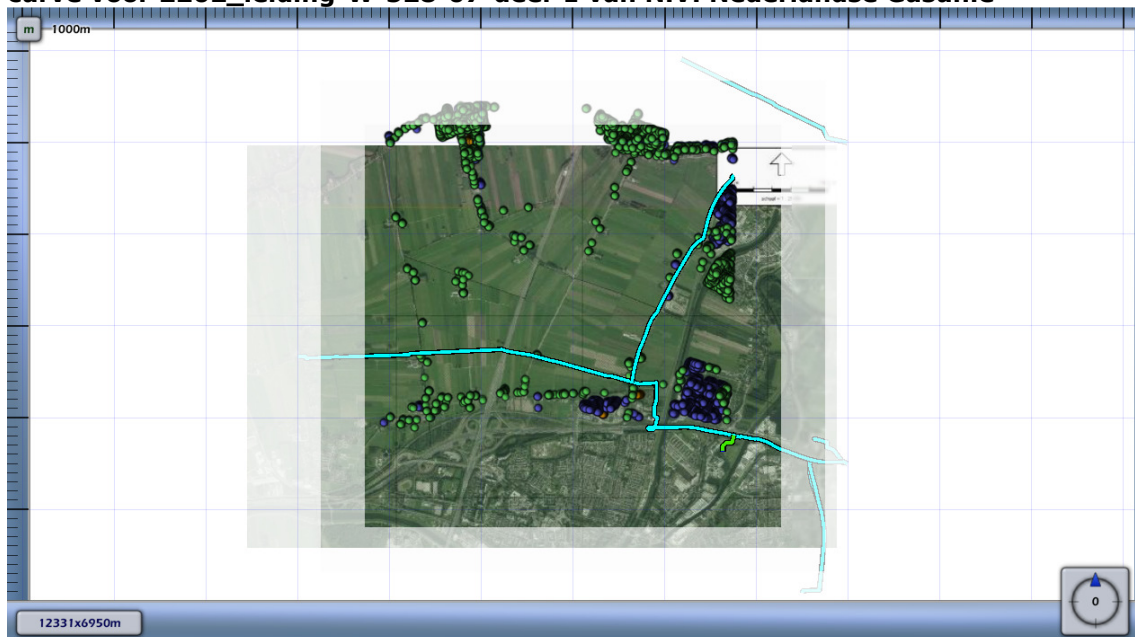
Figuur 4.5 Kilometer leiding behorende bij de maximale overschrijding van de FN-curve voor 2202_leiding-W-528-07-deel-1 van N.V. Nederlandse Gasunie
