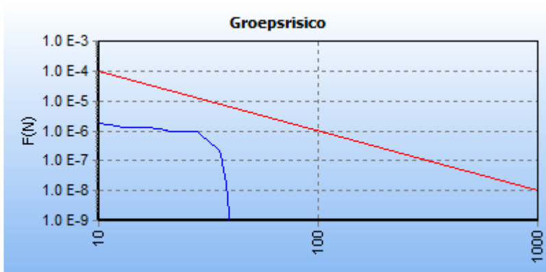
5.2 Figuur 5.2 FN curve voor 2202_leiding-W-528-01-deel-1 van N.V. Nederlandse Gasunie voor de kilometer tussen stationing 9730.00 en stationing 10730.00
