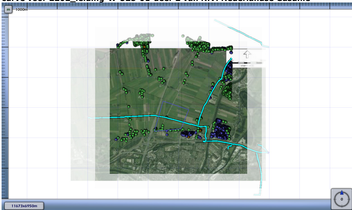
Figuur 4.3 Kilometer leiding behorende bij de maximale overschrijding van de FN-curve voor 2202_leiding-W-528-01-deel-2 van N.V. Nederlandse Gasunie
