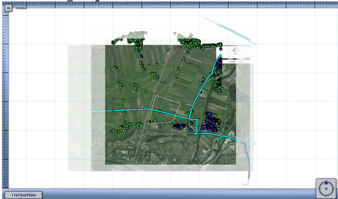
Figuur 4.7 Kilometer leiding behorende bij de maximale overschrijding van de FN-curve voor 2202_leiding-W-543-01-deel-1 van N.V. Nederlandse Gasunie
