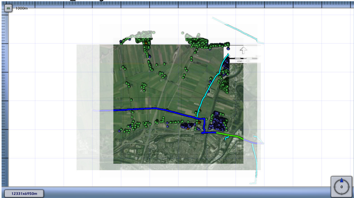
Figuur 4.2 Kilometer leiding behorende bij de maximale overschrijding van de FN-curve voor 2202_leiding-W-528-01-deel-1 van N.V. Nederlandse Gasunie
