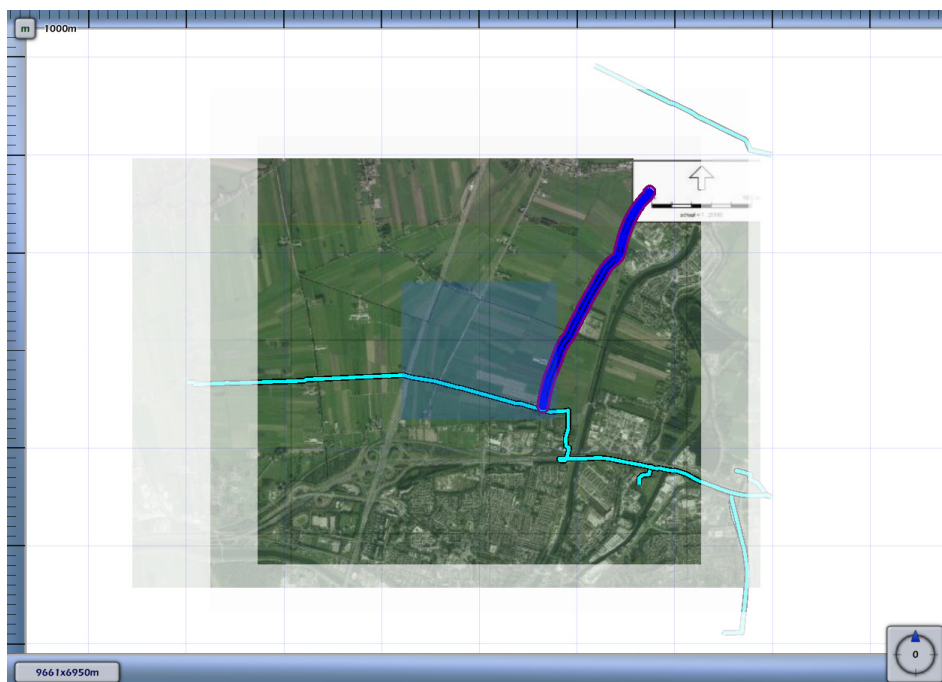
3.4 Figuur 3.4 Plaatsgebonden risico voor 2202_leiding-W-528-03-deel-1 van N.V. Nederlandse Gasunie
