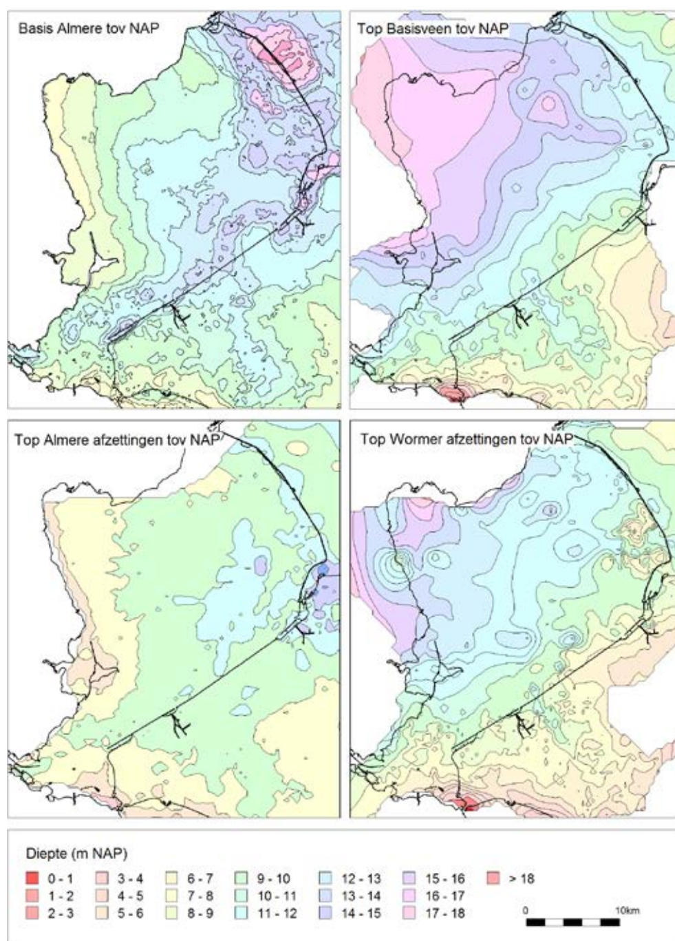
Afbeelding 19. Overzicht van de verschillende geologische modellen
