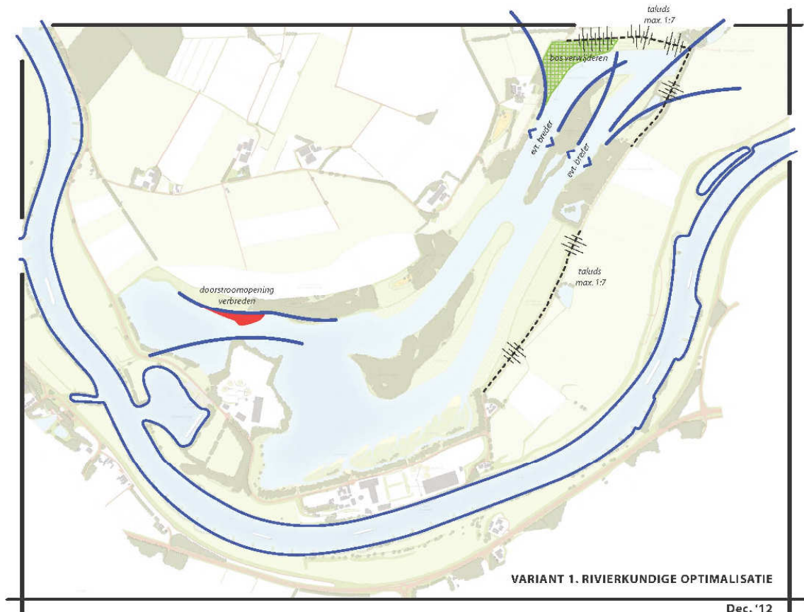
Figuur 4.6 Ontwerpprincipe Variant 1 en inrichtingsschets Variant 1
