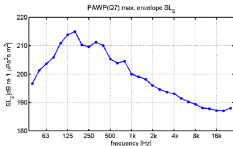
Figuur 20: Geschatte bovengrens voor het energie bronniveau spectrum (1/3-octave) voor het heigelluid, gebaseerd op de meetresultaten van Q7 (zie Bijlage 2).
