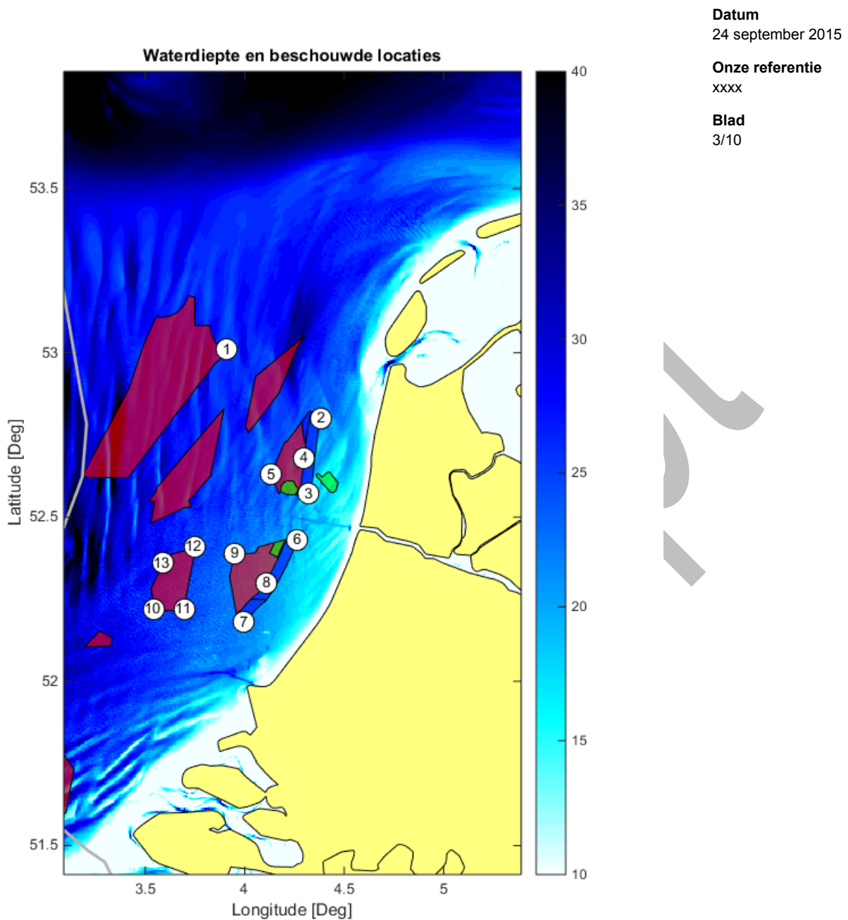
Figuur 2: Bathymetrikaart van het gebied met daarin aangegeven de contouren van de zoekgebieden en de 13 geselecteerde heilocaties waarvoor de verspreiding van het heigeluid is berekend.
