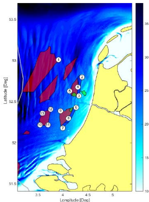
Figuur 21: Bathymetriekaart van het gebied met daarin aangegeven de contouren van de zoekgebieden en de 13 geselecteerde heilocaties waarvoor de verspreiding van het heigelluid is berekend
