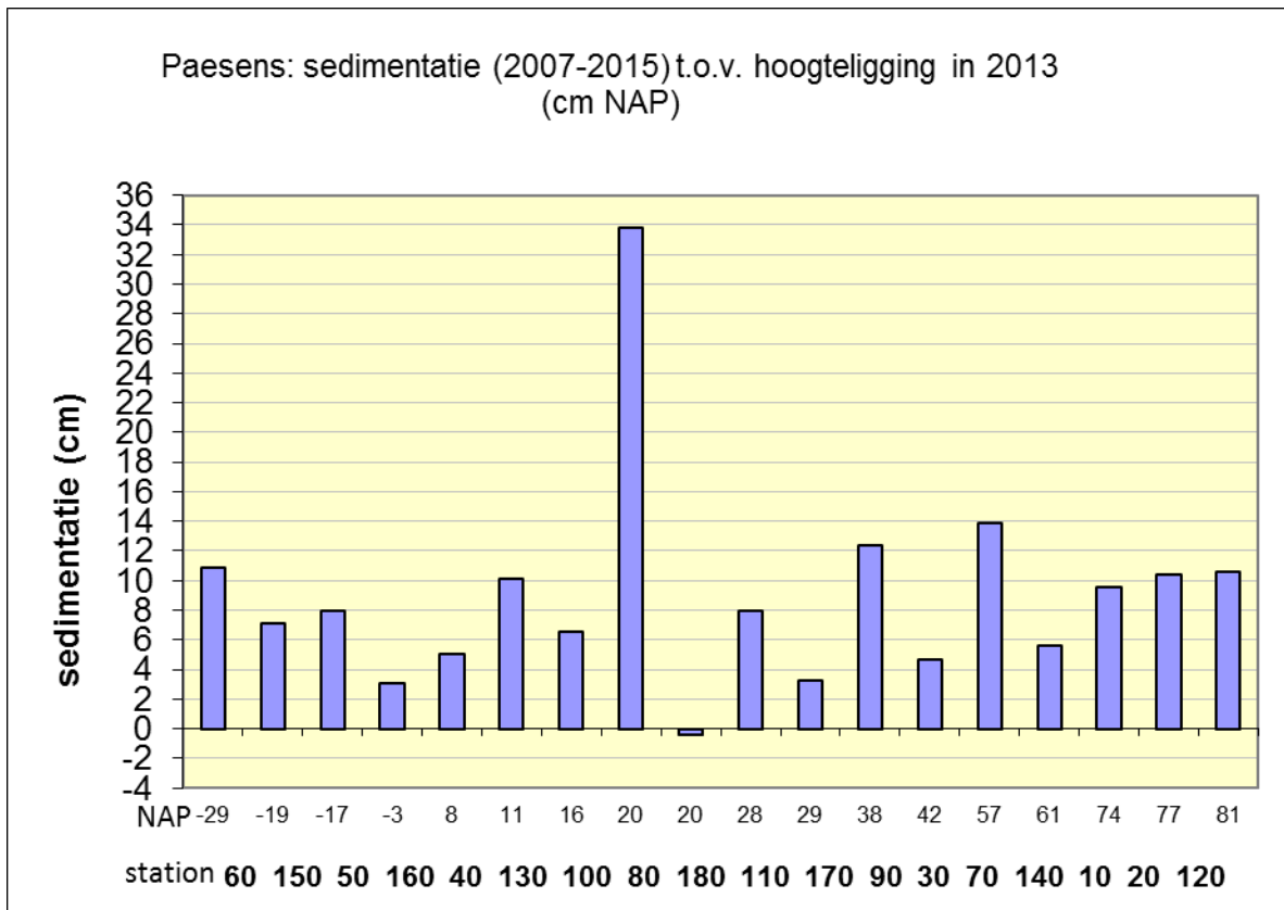
Figuur 29. Sedimentatie P10 – P180 in relatie tot de hoogteligging.
