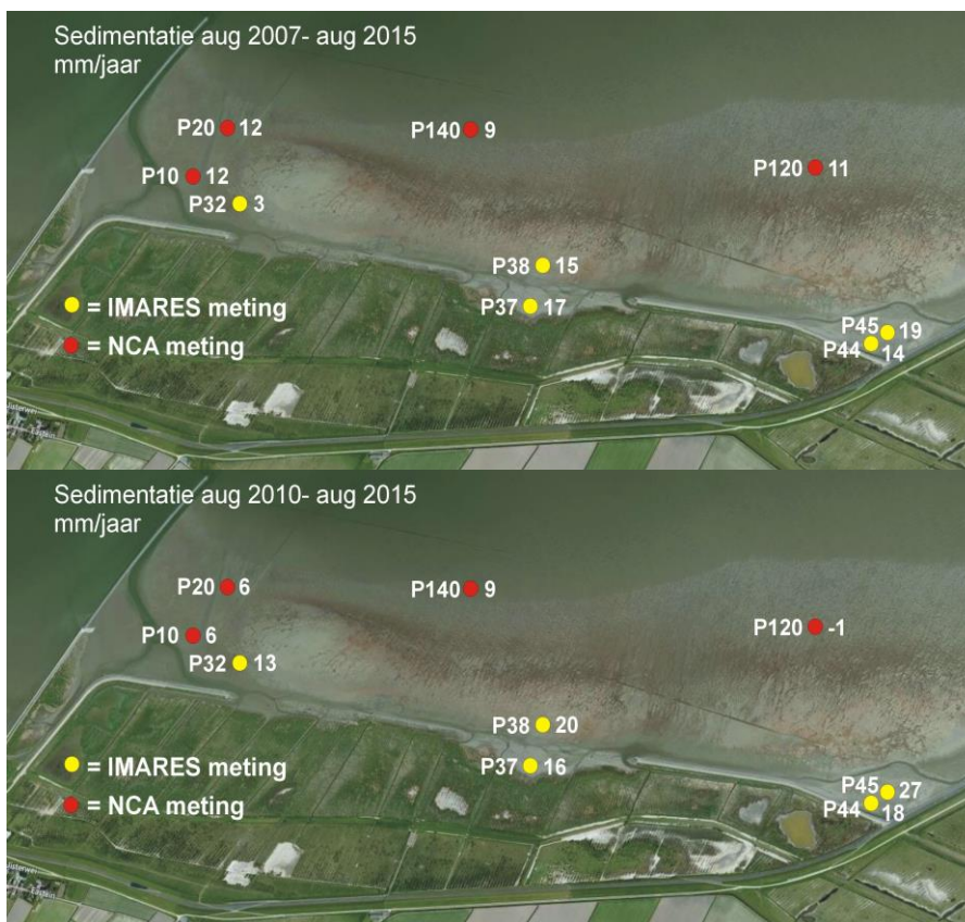
Figuur 35. Kaartbeeld met sedimentatie vergelijking van de meting van NCA en IMARES. Boven over periode aug2007-aug2015. Onder over periode aug2010-aug2015. Rechts van de gekleurde stip waarmee de locatie van het meetstation wordt aangeduid staat de sedimentatie in mm/jaar.
