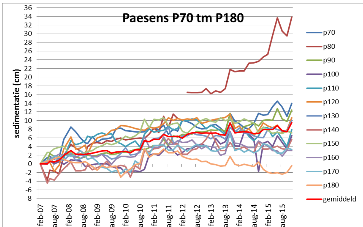
Figuur 14. Gemiddelde meetlijnen van de meetstations P70 tm P180 in het onderzoeksgebied bij Paesens. Tevens is het gemiddelde (rode lijn) van deze 12 meetlijnen genomen als weergave van de sedimentatie van het gebied waarin de meetstations liggen.
