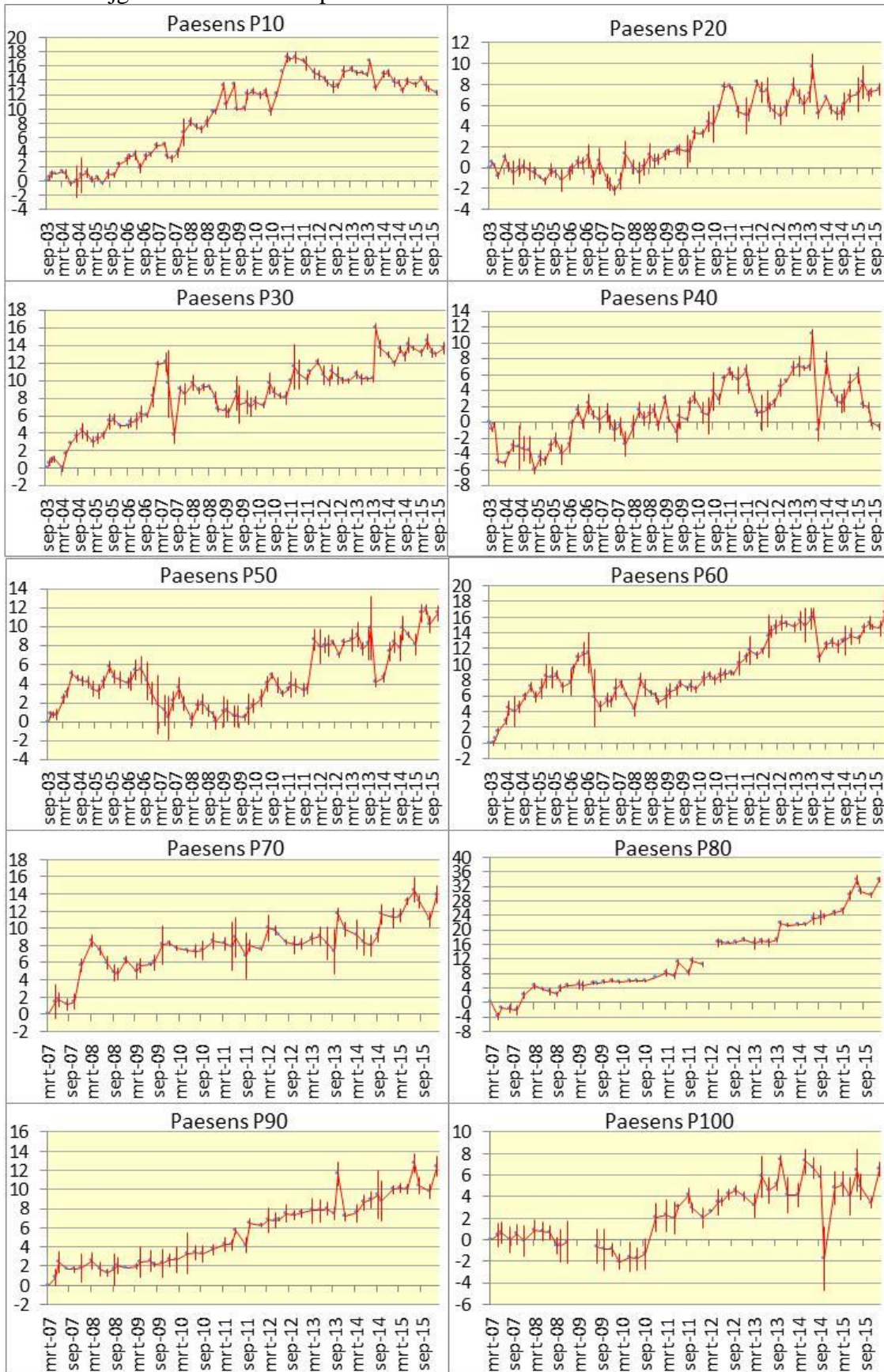
Bijlage A. Grafieken gemiddelde sedimentatie en SD van alle meetstations onderzoeksgebied Paesens bijgewerkt tm 2015. Op Y-as sedimentatie in cm.
