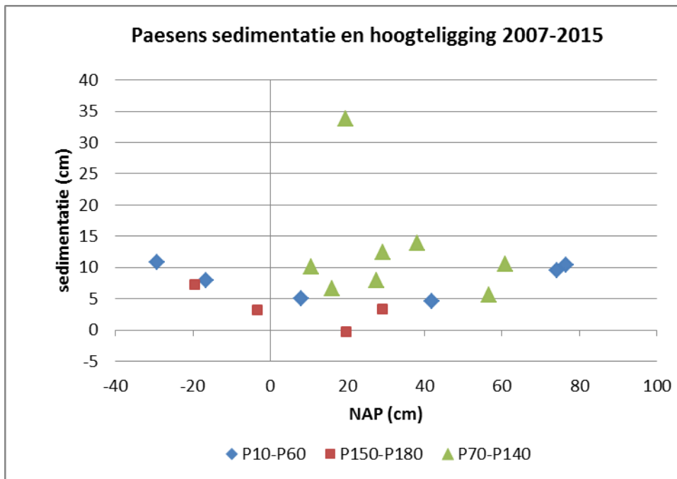
Figuur 30. Hoogteligging en sedimentatie van meetstations bij Paesens in de periode 2007-2015.
