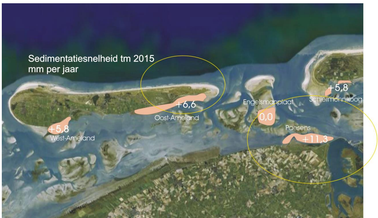
Figuur 24. Sedimentatiesnelheid per onderzoeksgebied in mm/jaar. De reeksen waarop het gemiddelde is gebaseerd variëren in lengte van 8 tot 14 jaar maar ze zijn allemaal bijgewerkt tm 2015.
