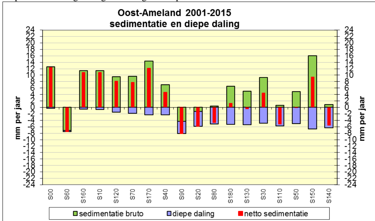
Figuur 31. Snelheid van sedimentatie en diepe bodemdaling in mm/jaar per meetstation (zie tabel 1). Diepe daling berekend over feb 2001-feb 2014. De sedimentatie aan het oppervlak is berekend tm 2015.
