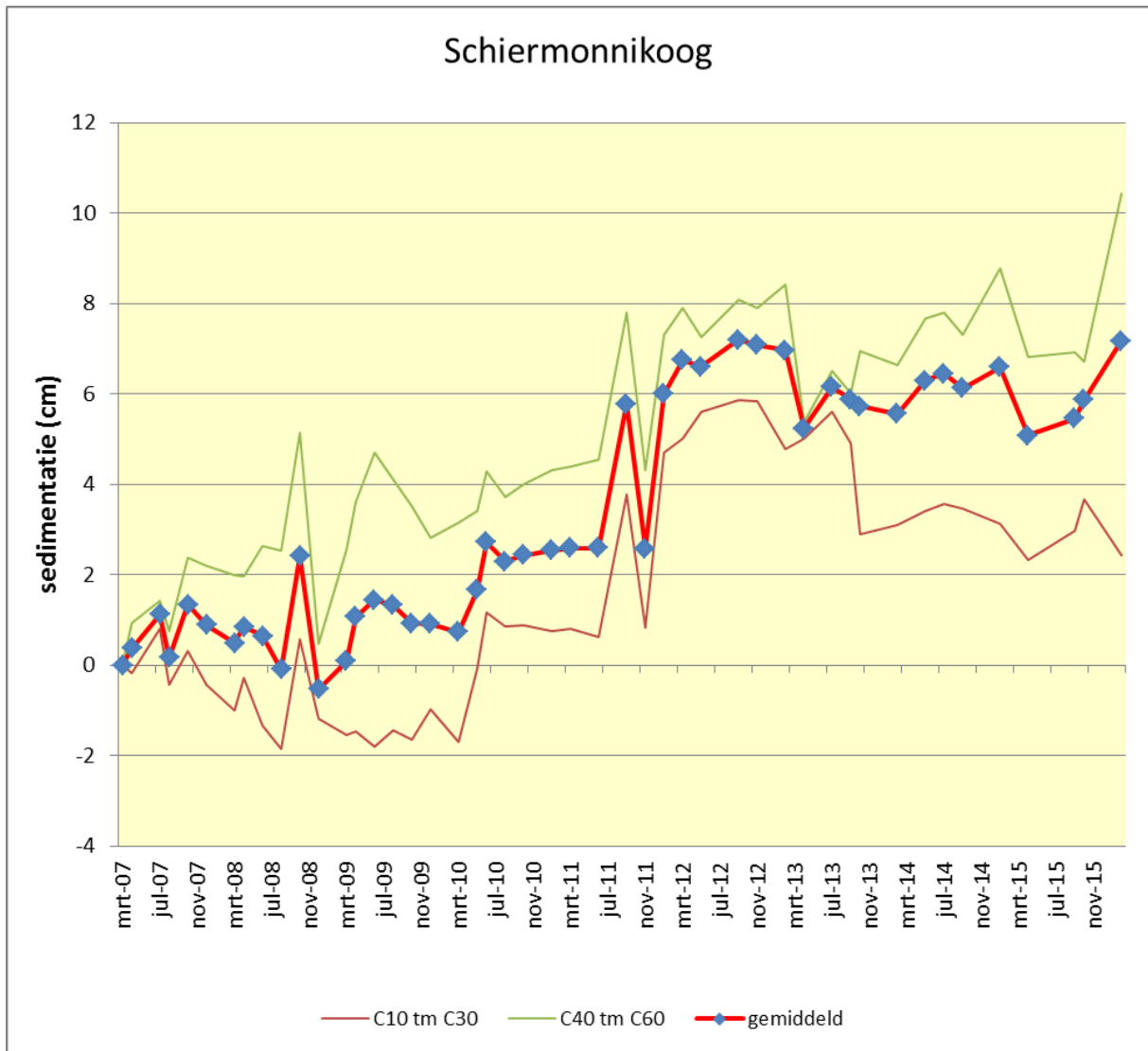
Figuur 19. Gemiddelde van de gebieden C10 – C30 en C70 (oost) en C40 – C60 (west) en het overall gemiddelde van de meetstations C10 tm C70 in het onderzoeksgebied Schiermonnikoog.
