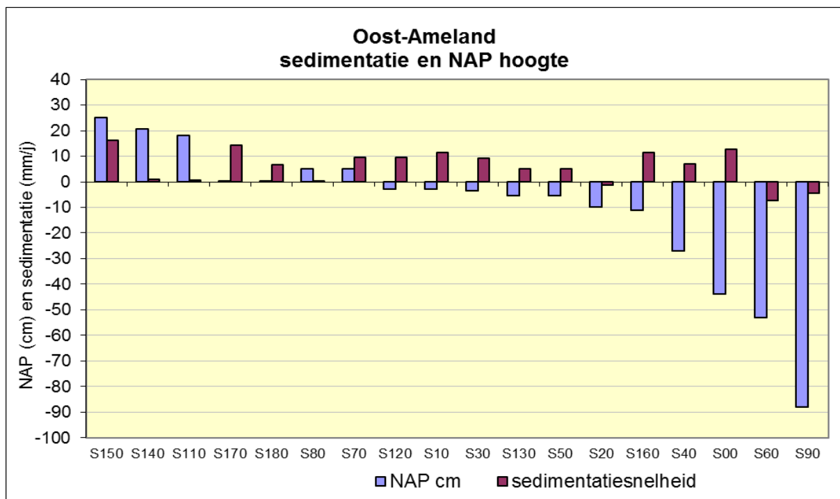
Figuur 27. Wadsedimentatie ten opzichte van hoogteligging van de meetstations bij Oost-Ameland. Sedimentatiesnelheid in mm per jaar over de totale meetperiode. Meetperiode van de meetstations varieert van 8 tot 14 jaar tussen 2000 en 2014 (zie tabel 2). Meetdatum sedimentatie is in december 2014. Een uitzondering is S100, dit station is door geulvorming in 2009 verloren gegaan.
