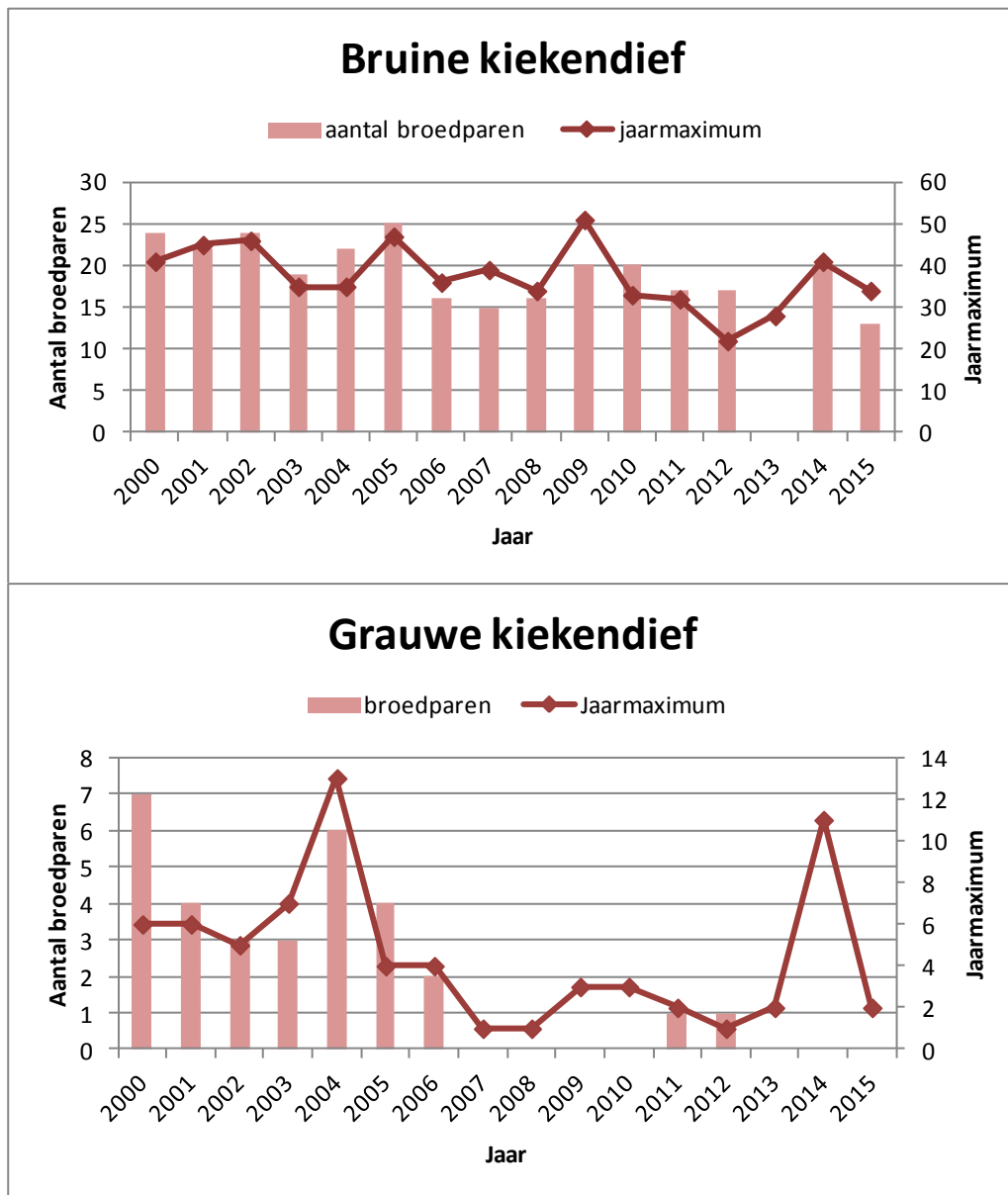
Figuur 5.1 Aantal broedparen en jaarmaximum tijdens de maandelijkse vogeltellingen van Bruine en Gruuwe kiekendief in het Lauwersmeer in de periode 2000-2015. Een jaar loopt van januari -december. In 2013 zijn de broedparen niet geteld. Bron voor het aantal broedvogels: Kleefstra & de Boer 2016.
