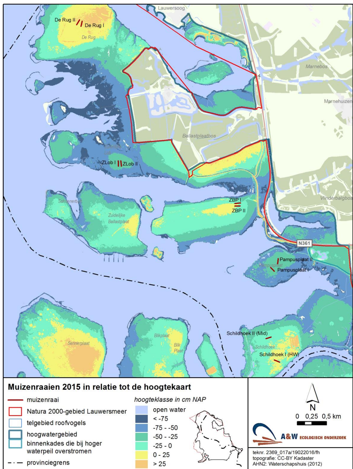
Figuur 4.1 Overzicht van bemonsterde muizenraaien in het Lauwersmeer in relatie tot de hoogtekaart in oktober 2015.
