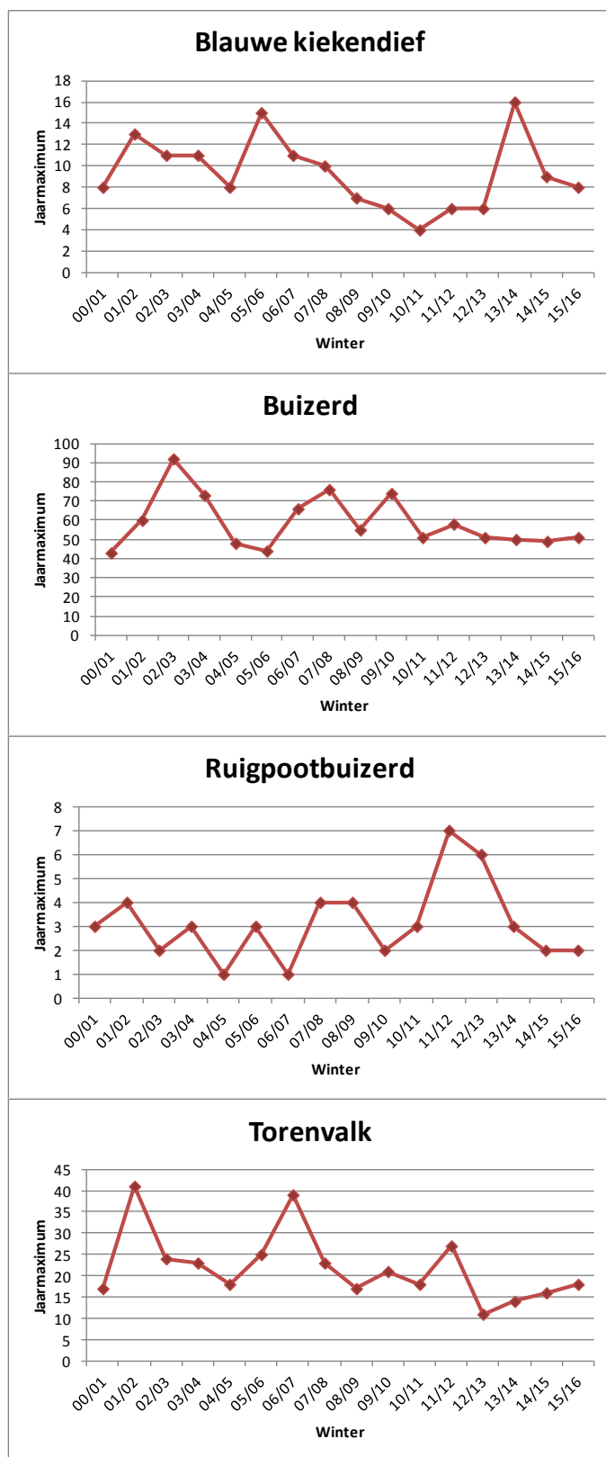
Figuur 5.2 Jaarmaximum van Blauwe kiekendief, Buizerd, Ruigpootbuizerd en Torenvalk tijdens de maandelijkse vogeltellingen in het Lauwersmeer in de periode 2000/2001-2015/2016. Een jaar loopt van juli - juni, in 2015/2016 van juli - februari.
