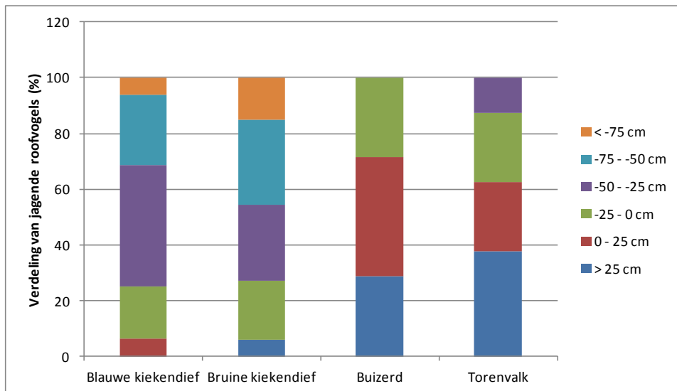
Figuur 5.6 Het voorkomen van jagende muizenetende roofvogels in relatie tot bodemhoogte binnen het hoogwatergebied in het Lauwersmeer in 2015. Gebieden die omgeven worden door binnenkades, die deels een gestuurd waterpeil hebben en pas bij een hoger waterpeil overstroomd, zijn hierbij niet meegerekend.
