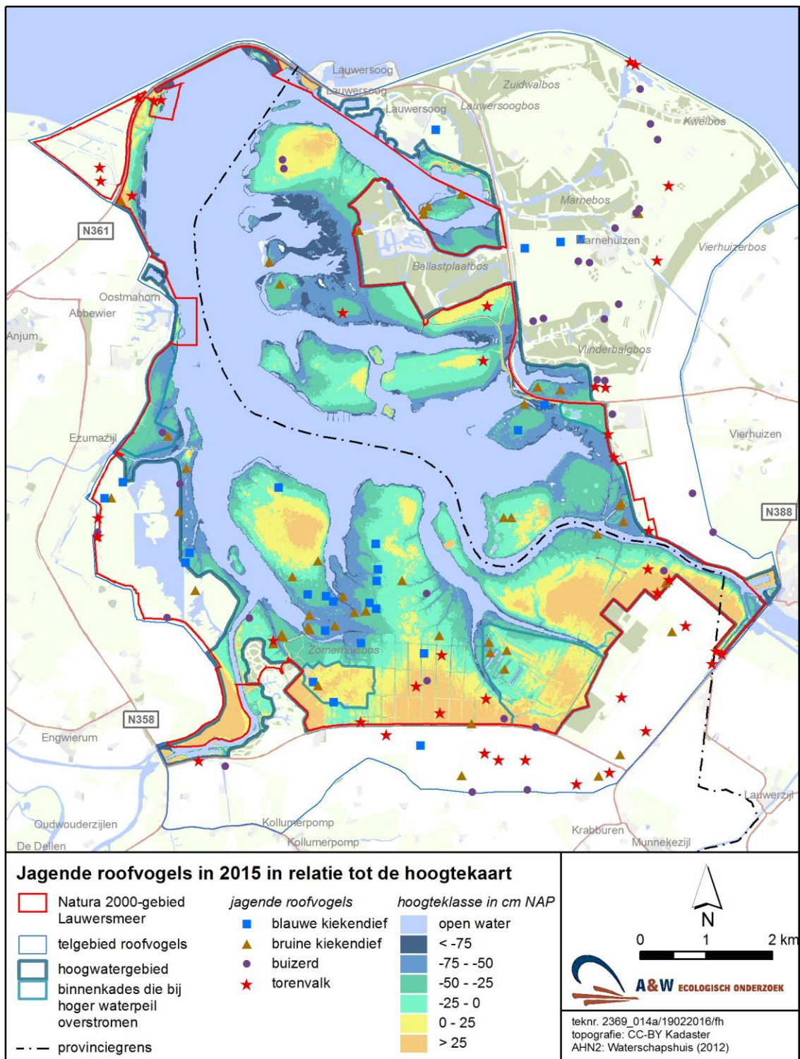
Figuur 5.5 De verspreiding van jagende muizenetende roofvogels in het Lauwersmeer in 2015 in relatie tot bodemhoogte. De hoogtekkaart is alleen weergegeven voor het hoogwatergebied.
