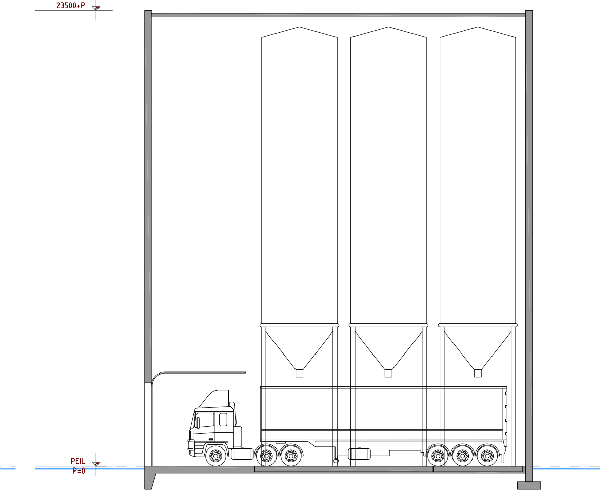
Doorsnede D-D Schaal 1:200
