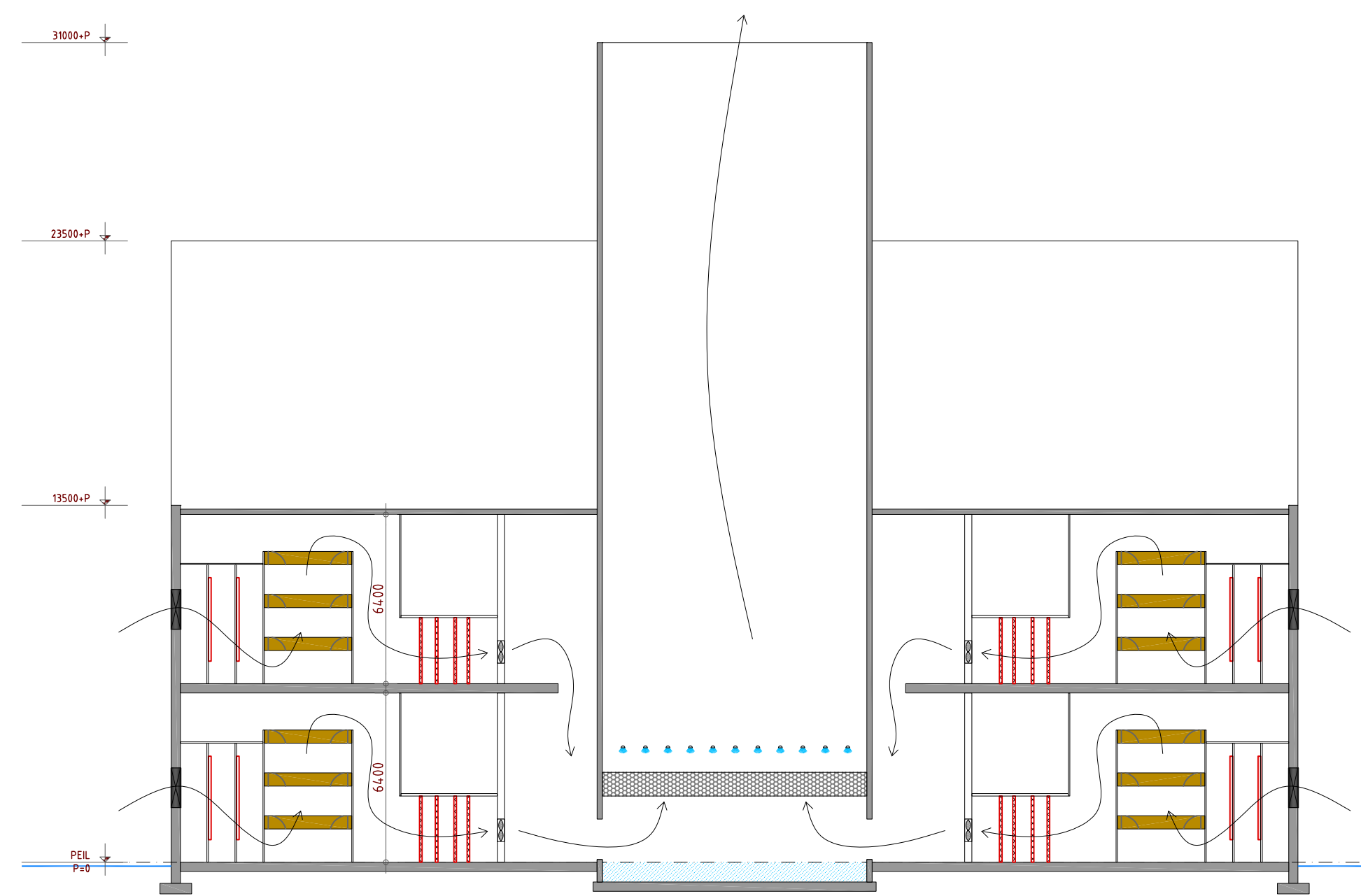
Doorsnede A-A Schaal 1:200
