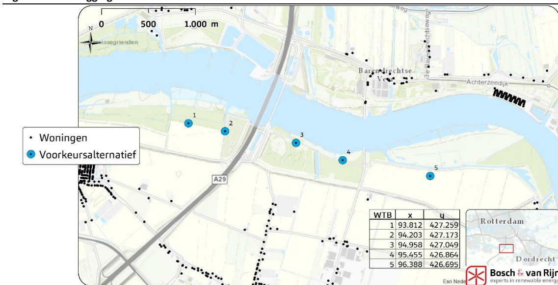
Figuur 3 Ligging van de windturbines van het voorkeursalternatief.
