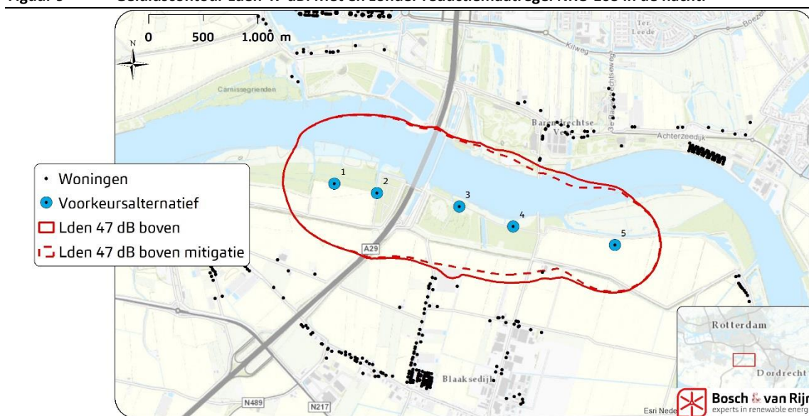
Figuur 9 Geluidscontour Lden 47 dB. Met en zonder reductiemaatregel NRO 103 in de nacht.
