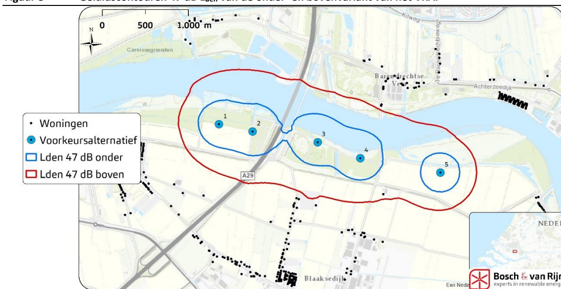
Figuur 8 Geluidscontouren 47 dB Lden van de onder- en bovenvariant van het VKA.
