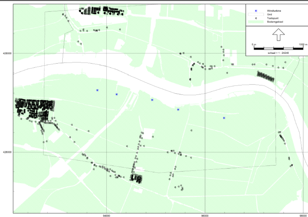
Figuur 10 Basis van het rekenmodel: windturbines, woningen, bodemgebieden en een rekgid.
