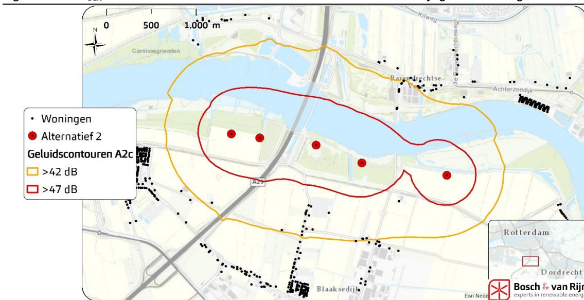
Figuur 6 L_{DEN} 47 en 42 dB-contour van de Alternatief A2c ter illustratie. Zie Bijlage D voor overige contouren.
