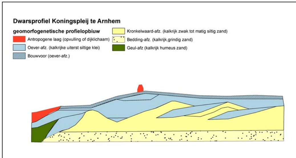
Figuur 3.3 Een globaal dwarsprofiel van de jonge kronkelwaard Koningspleij bij Arnhem. Het hoogste punt (dijkje) bevindt zich op 11,60 m +NAP, het laagste punt (geul) op 6,25 m +NAP. Het bodemprofiel is gebaseerd op 9 boringen met onderlinge afstanden van 50 m (450 m lang) en boordiepten van drie meter. De grindrijke beddingafzettingen bevinden zich in het zuiden dieper dan 3 m en zijn niet aangeboord. Op het figuur zijn deze onderste geulafzettingen wel ingetekend. Alle getoonde bodemlagen behoren tot de Formatie van Echteld. Ze stammen uit de periode eind late middeleeuwen tot aan de laatste bedijking (1400 tot 1775 na Chr.).
