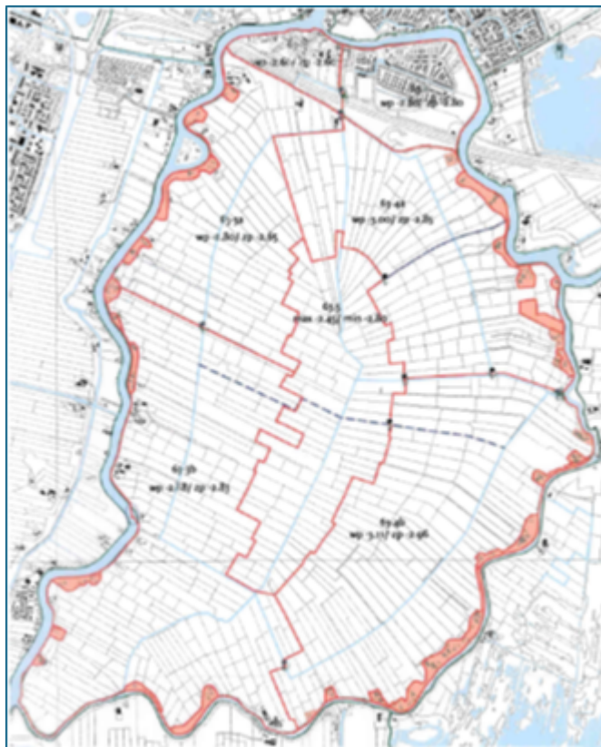
Afbeelding 5.4 Peilgebieden en hoogwatervoorzieningen (bron: startnotitie Ronde Hoep, 2016)
