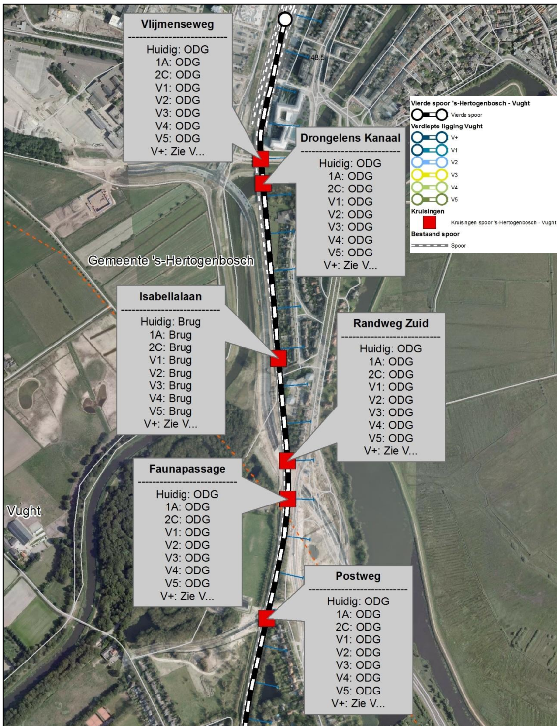
Afbeelding 7: Uitvoeringen kruisingen Vught Noord
