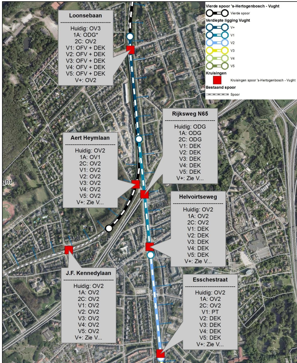
Afbeelding 8: Uitvoeringen kruisingen Vught Midden
