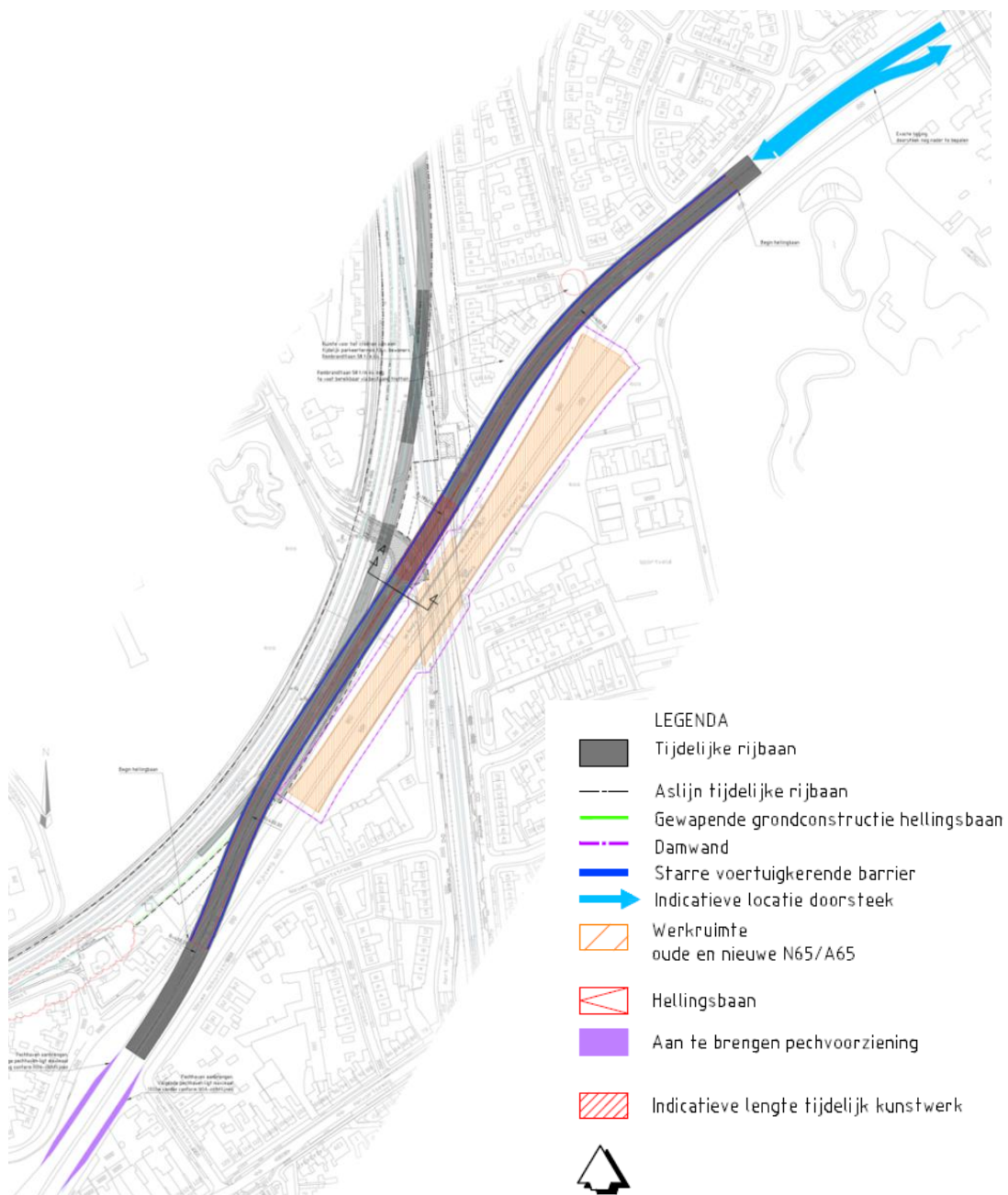
Afbeelding 12: Bovenaanzicht tijdelijke kruising A65/N65
