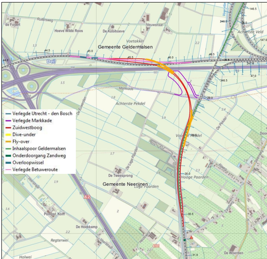
Afbeelding 21: Situatieschets variant V2 Hoog
