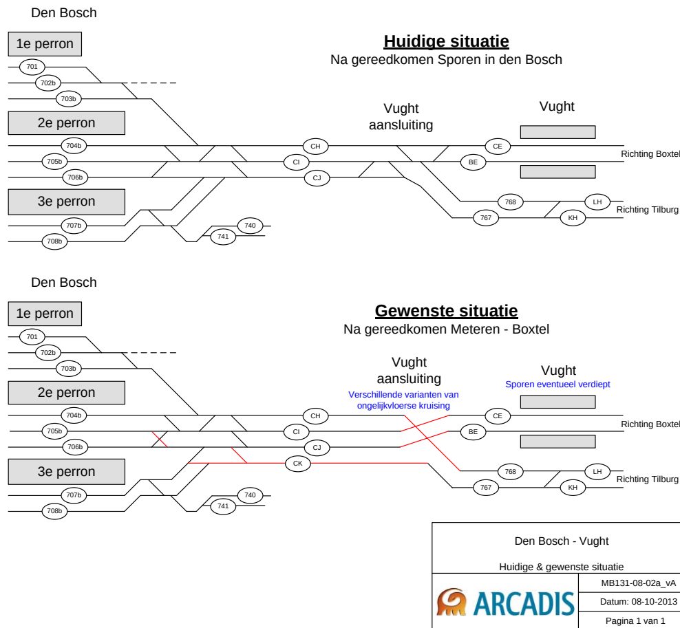
Abbeelding 2: Schematische weergave sporen in huidige situatie (na gereedkomen Sporen in Den Bosch) en in de projectsituatie
