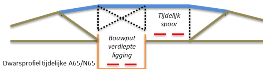
Afbeelding 13: Dwarsprofiel tijdelijke kruising A65/N65
