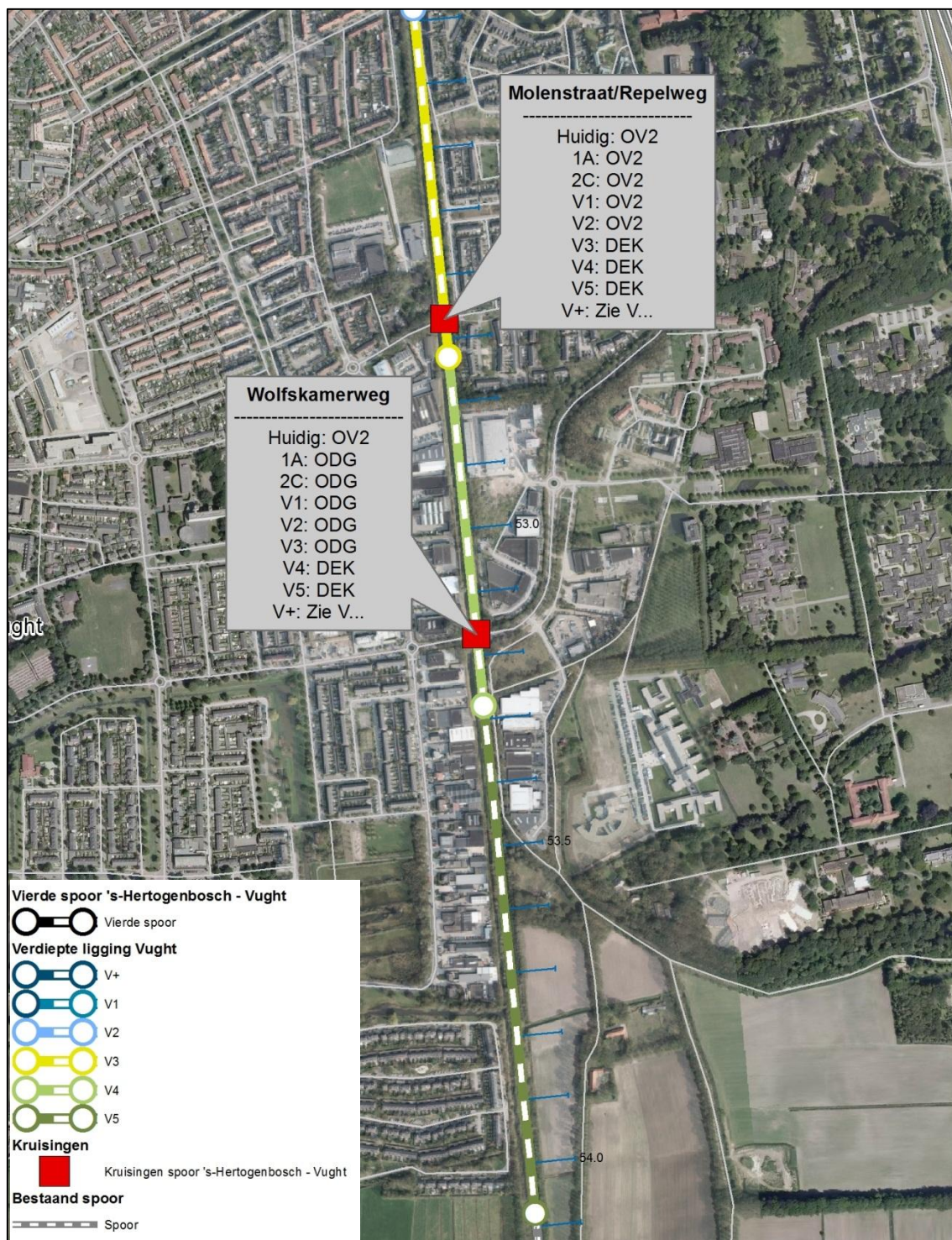
Afbeelding 9: Uitvoeringen kruisingen Vught Zuid
