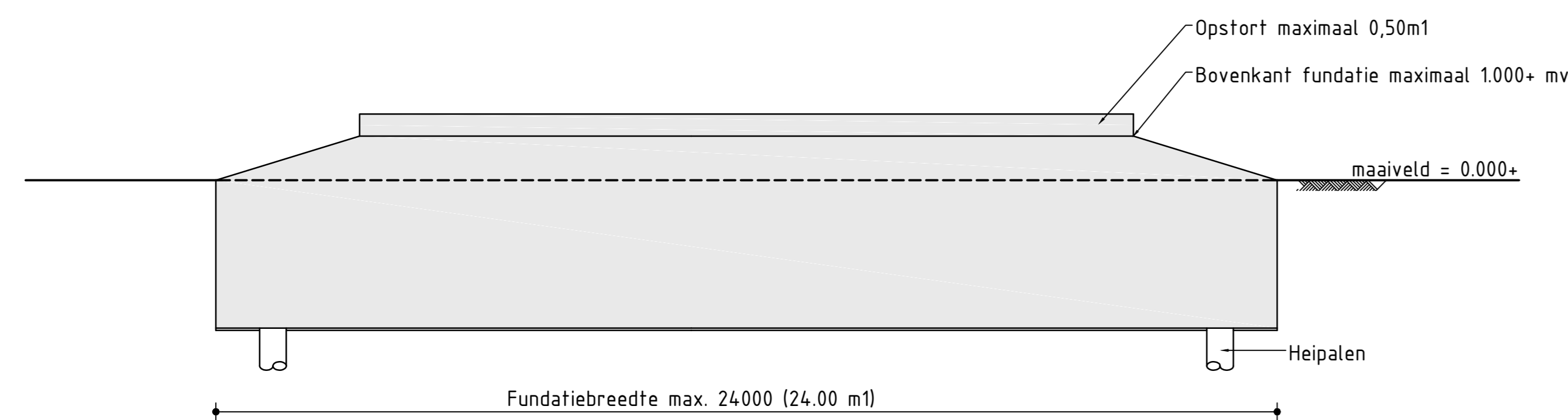
Principe Detail fundatie Schaal 1 : 100
