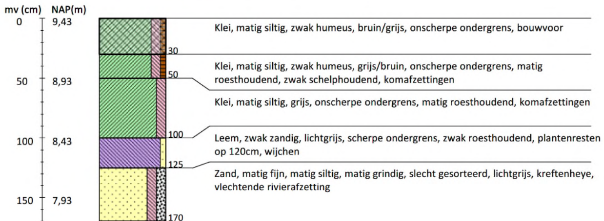
Boring 29 RD-coördinaten: 200959/440905
