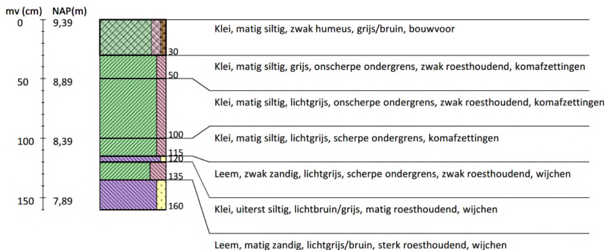
Boring 31 RD-coördinaten: 200847/440916
