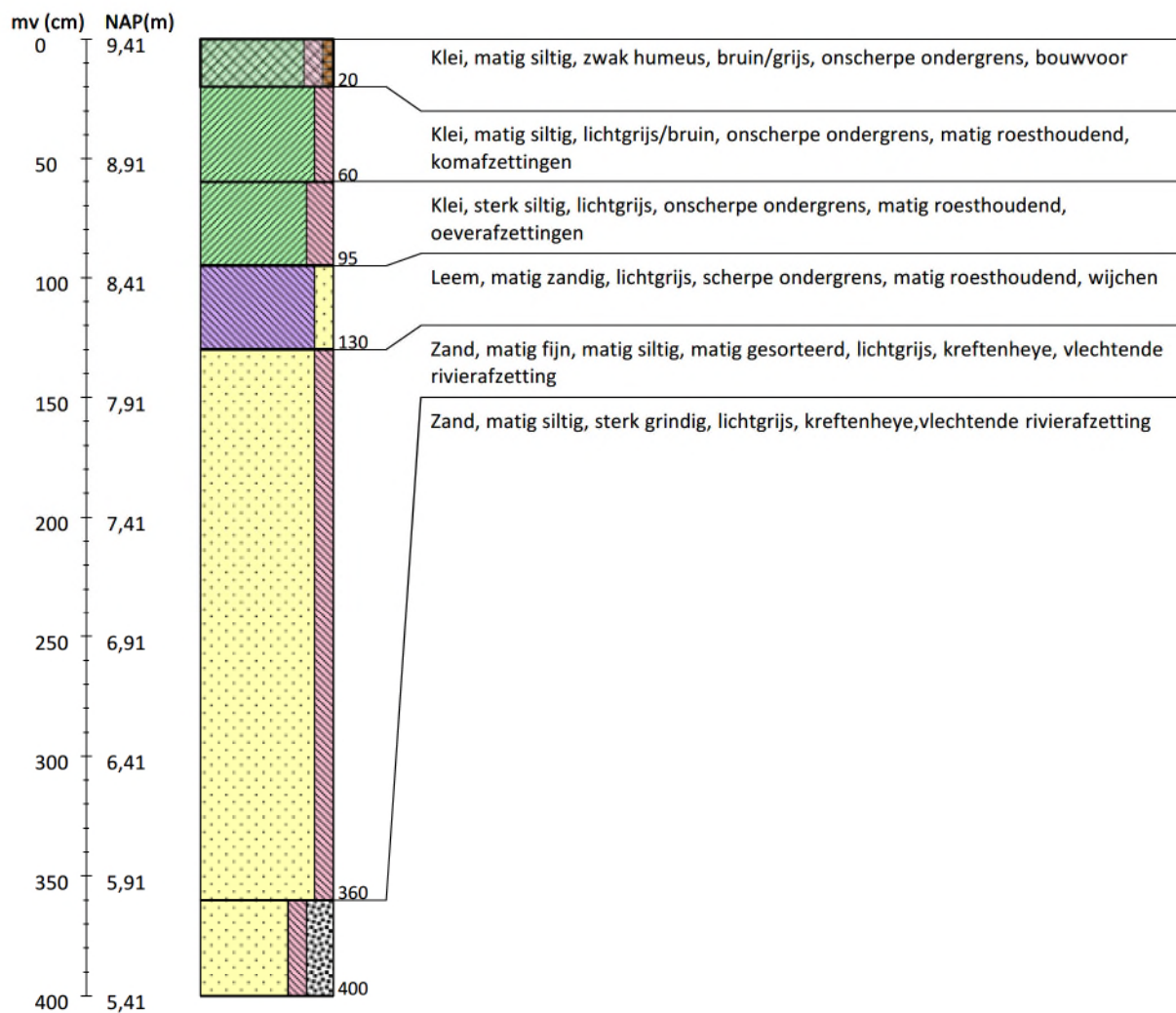
Boring 50 RD-coördinaten: 201113/440843
