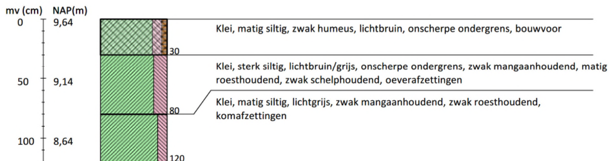
Boring 15 RD-coördinaten: 200495/440125
