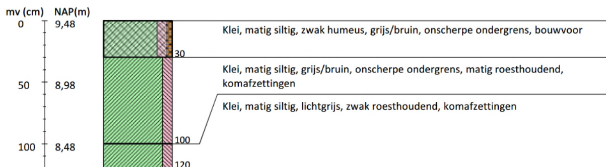
Boring 26 RD-coördinaten: 200568/440552
