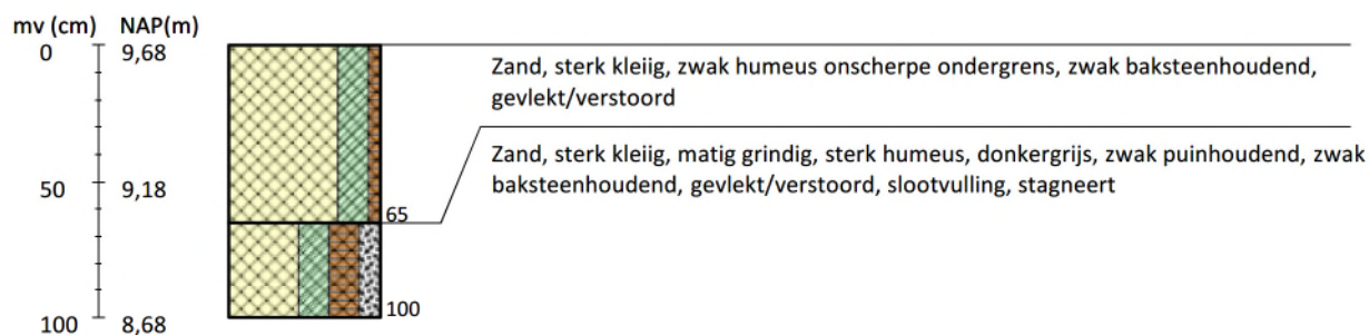
Boring 34 RD-coördinaten: 200725/440919
