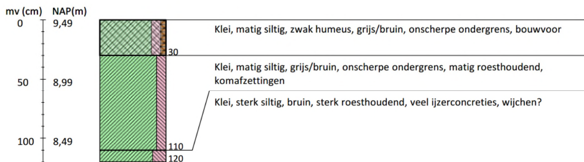
Boring 25 RD-coördinaten: 200587/440514
