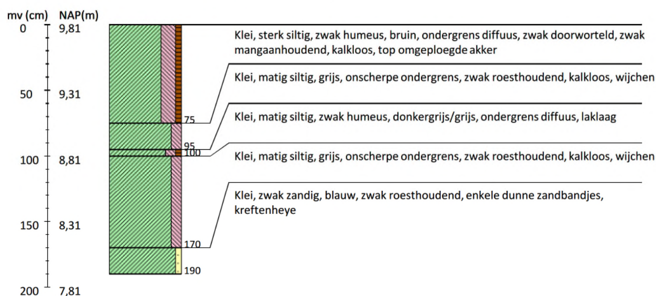
Boring 64 RD-coördinaten: 200097/439395
