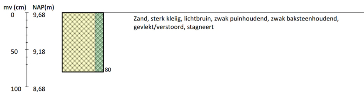
Boring 36 RD-coördinaten: 200657/440898
