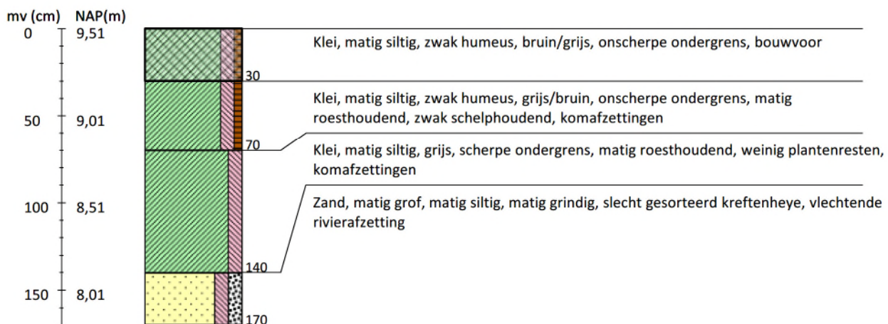
Boring 30 RD-coördinaten: 200903/440911
