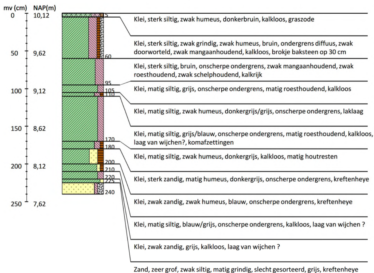
Boring 55 RD-coördinaten: 200005/439047
