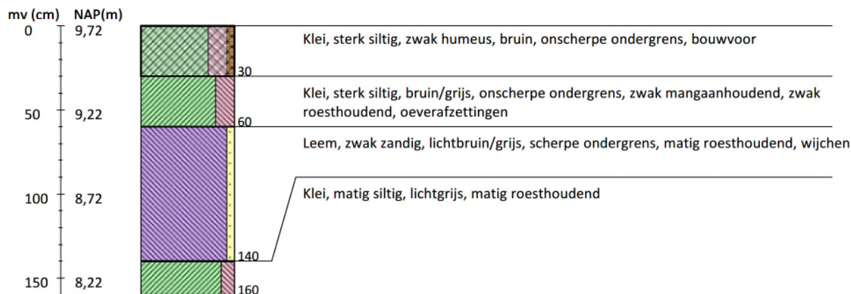
Boring 9 RD-coördinaten: 200366/439912
