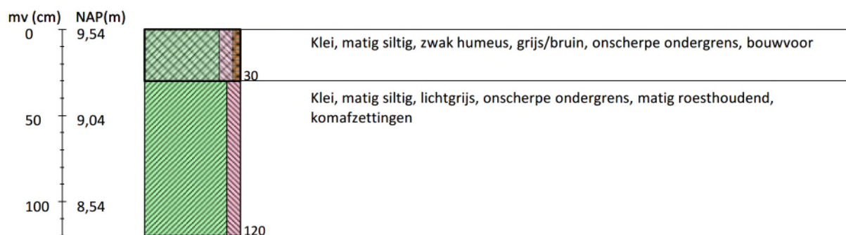
Boring 24 RD-coördinaten: 200608/440479
