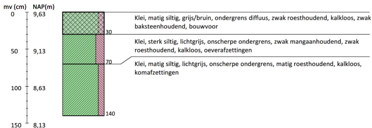
Boring 2 RD-coördinaten: 200283/439781
