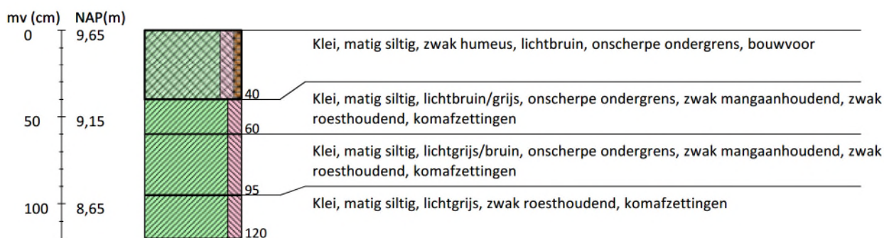
Boring 18 RD-coördinaten: 200565/440238
