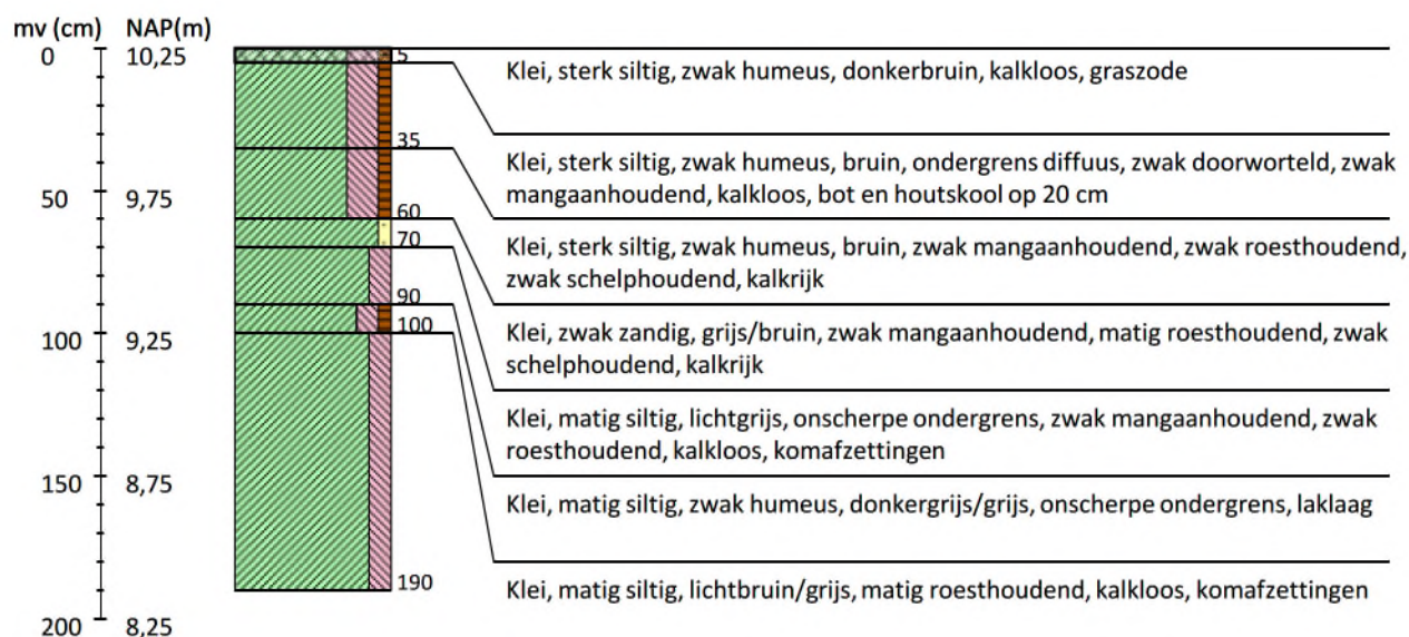
Boring 54 RD-coördinaten: 199987/439025
