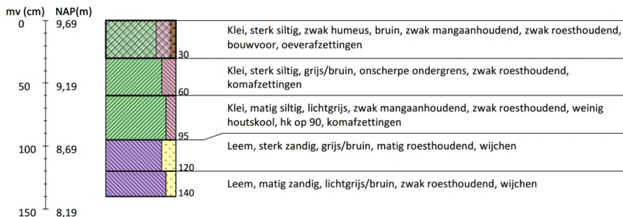
Boring 11 RD-coördinaten: 200408/439983
