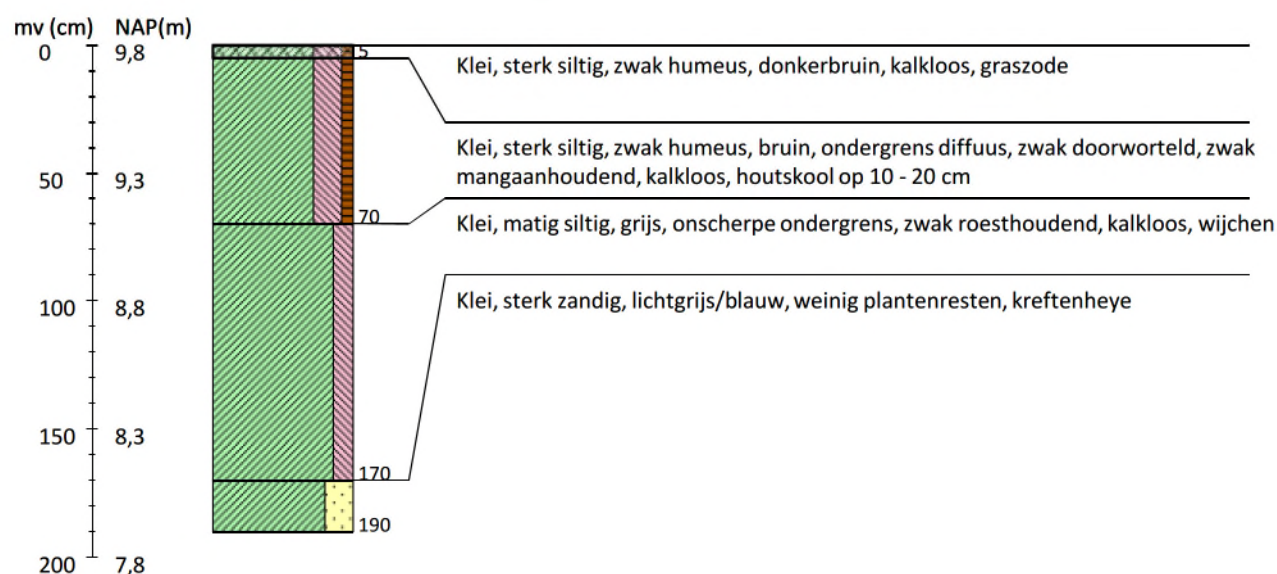
Boring 63 RD-coördinaten: 200088/439355
