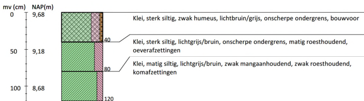
Boring 17 RD-coördinaten: 200544/440203
