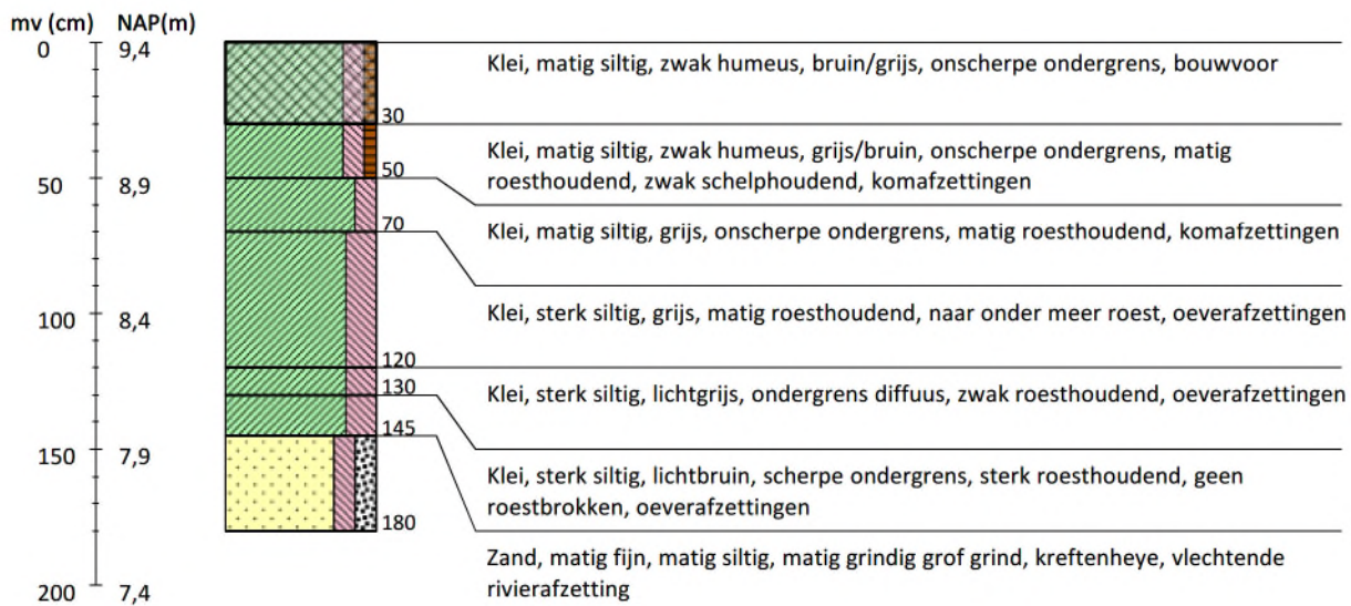
Boring 28 RD-coördinaten: 201001/440890
