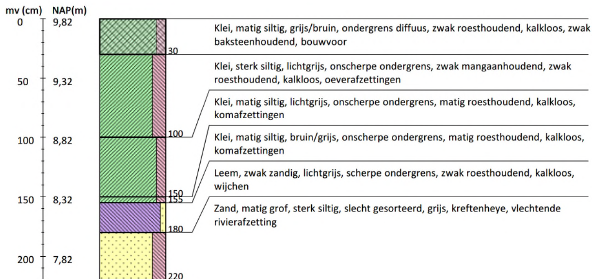
Boring 1 RD-coördinaten: 200309/439813
