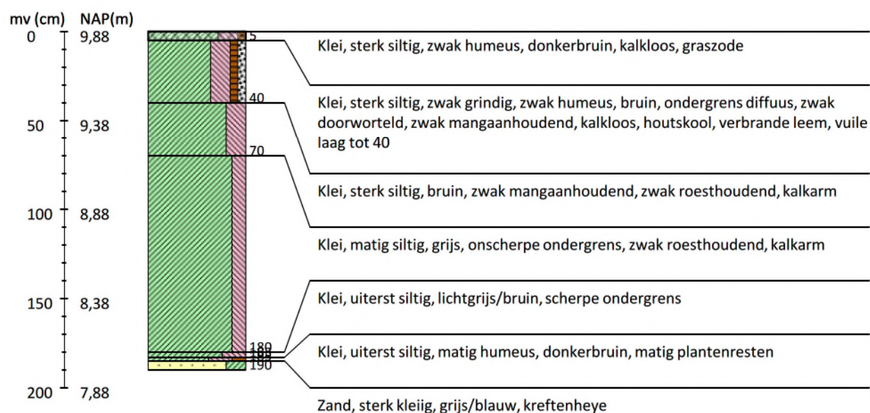
Boring 61 RD-coördinaten: 200067/439277
