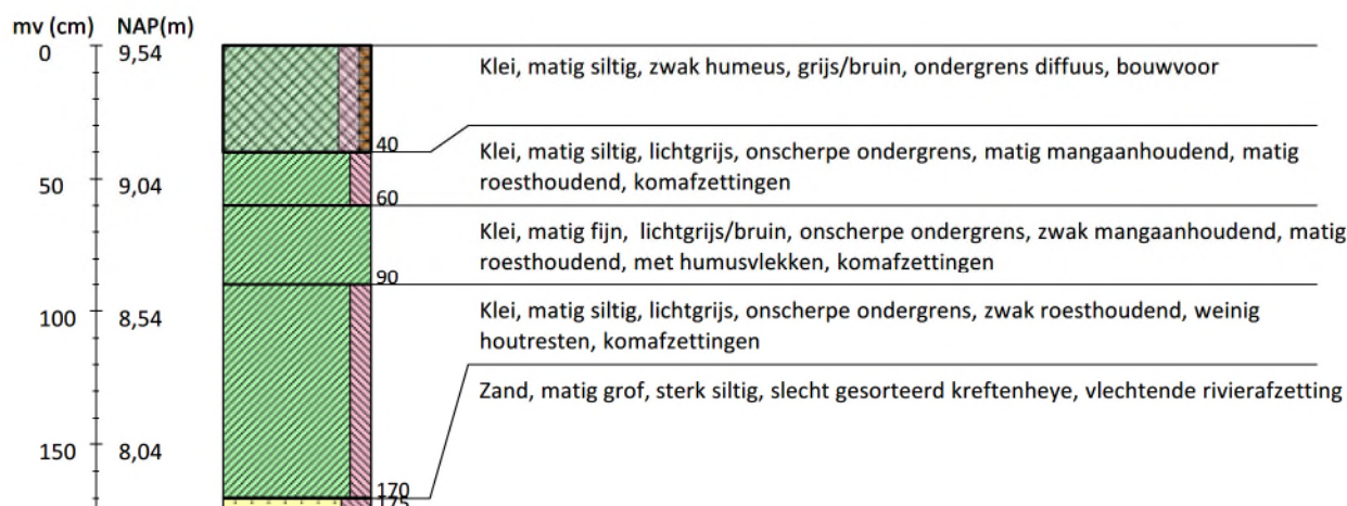
Boring 22 RD-coördinaten: 200654/440401
