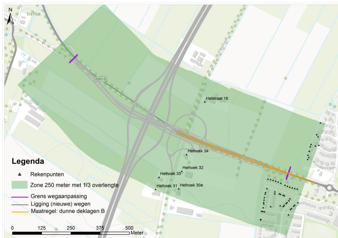
Figuur 5-1: Wegaanpassing Oostsingel, N801
