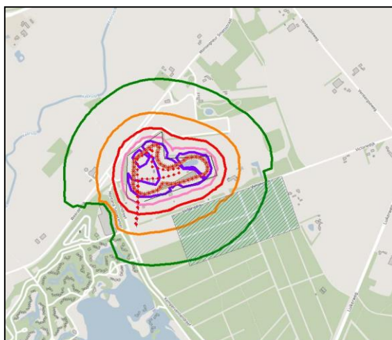
Geluidcontouren AK-situatie 1
