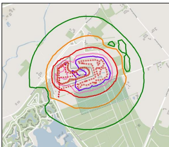
Geluidcontouren AK-situatie
