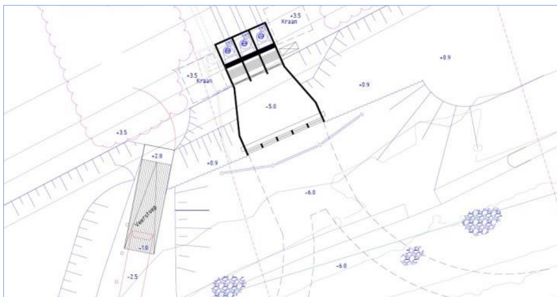
Afbeelding 13: Overzichtstekening innamewerk en omgeving (concept)
