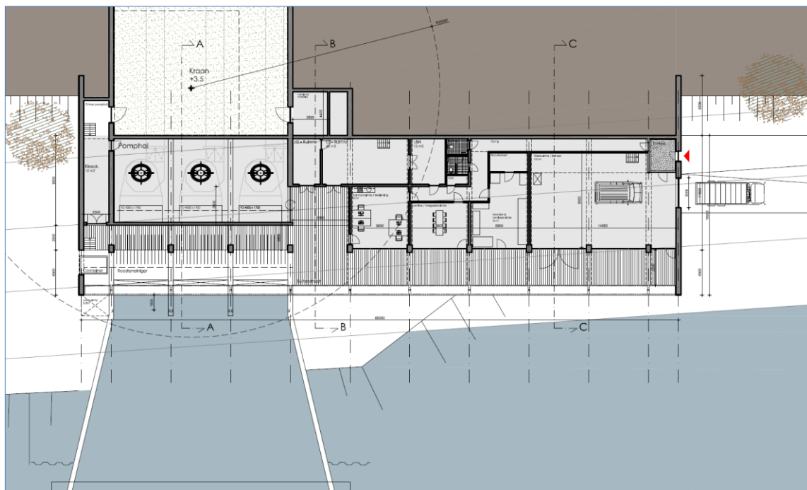
Afbeelding 15: Impressie plattegrond innamegebouw
