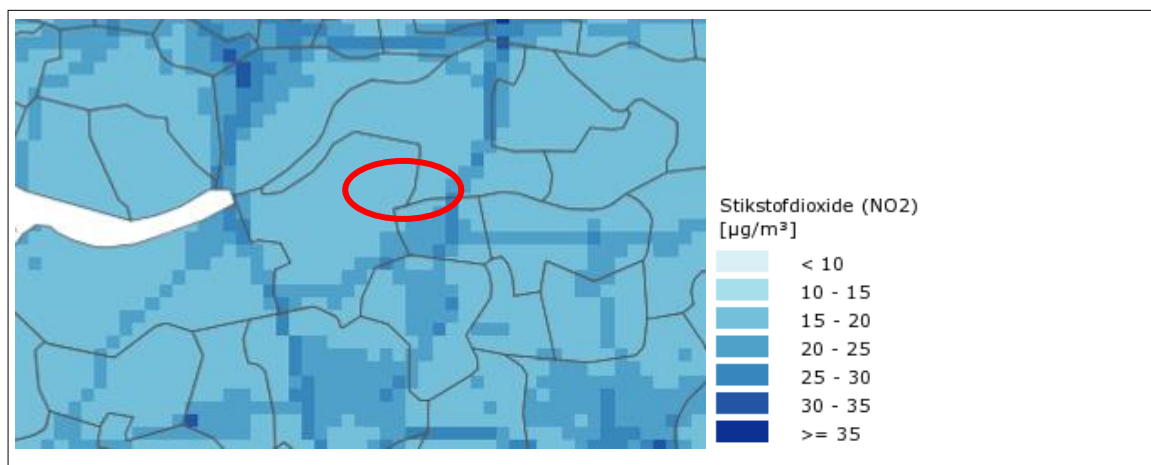
Afbeelding 30: Jaargemiddelde concentratie stikstofdioxide 2016 (Bron: http://geodata.rivm.nl/gcn/ RIVM)
