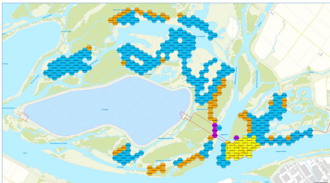
Afbeelding 35: Stikstofdepositie en ontwikkelingsruimte basisvariant+ (2019)
