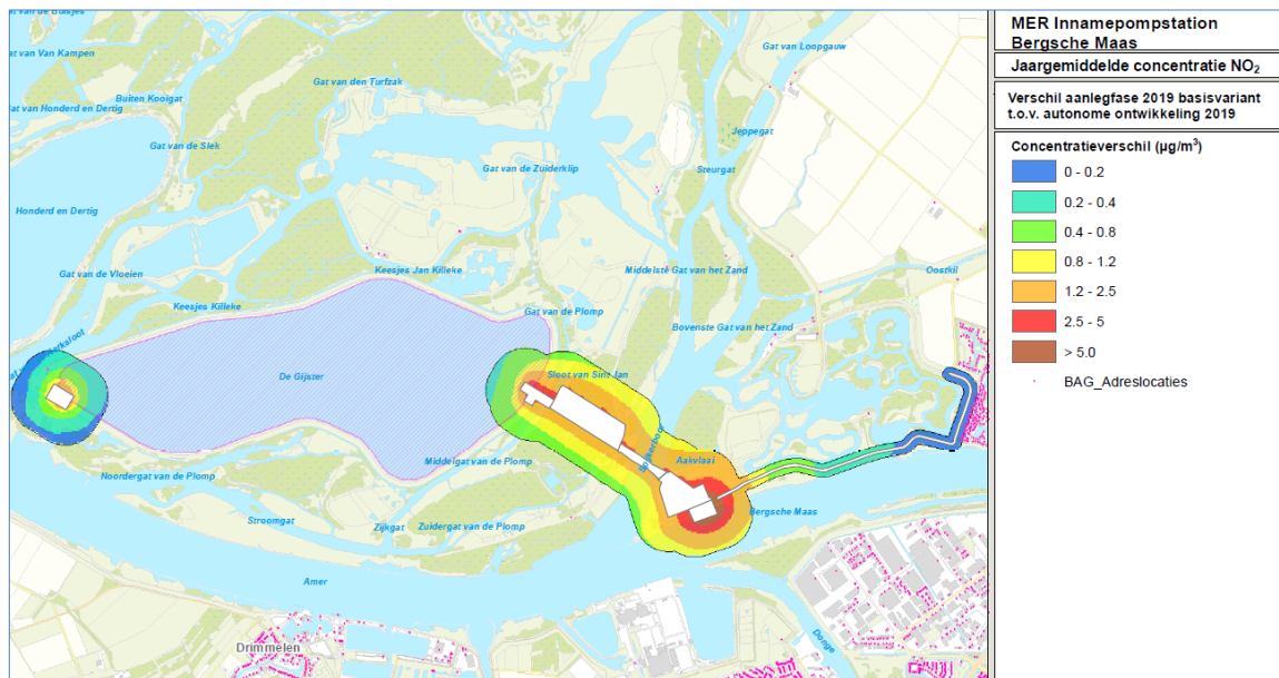
Afbeelding 33: Verschil jaargemiddelde concentratie NO 2 basisvariant (2019) t.o.v. autonome ontwikkeling
