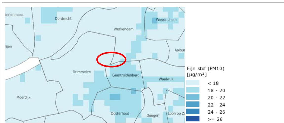
Afbeelding 31: Jaargemiddelde concentratie PM 10 2016 (Bron: http://geodata.rivm.nl/gcn/ RIVM)
