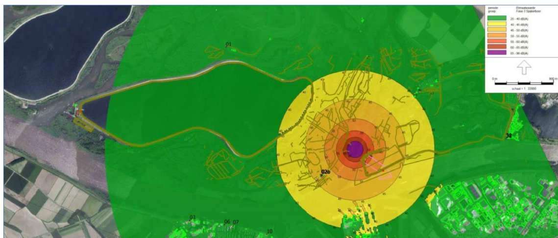
Afbeelding 27: Geluidcontouren werkzaamheden Spijkerboor
