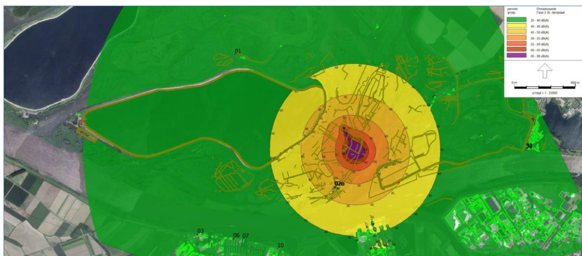
Afbeelding 26: Geluidcontouren werkzaamheden St. Jansplaat
