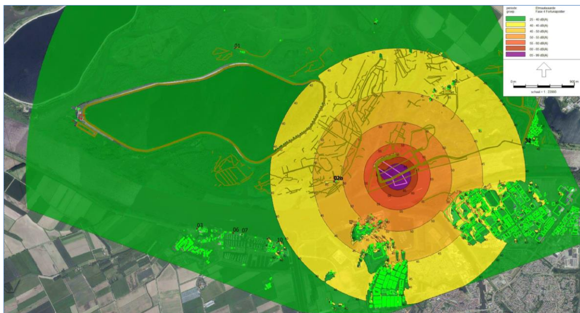
Afbeelding 28: Geluidcontouren werkzaamheden Fortunapolder
