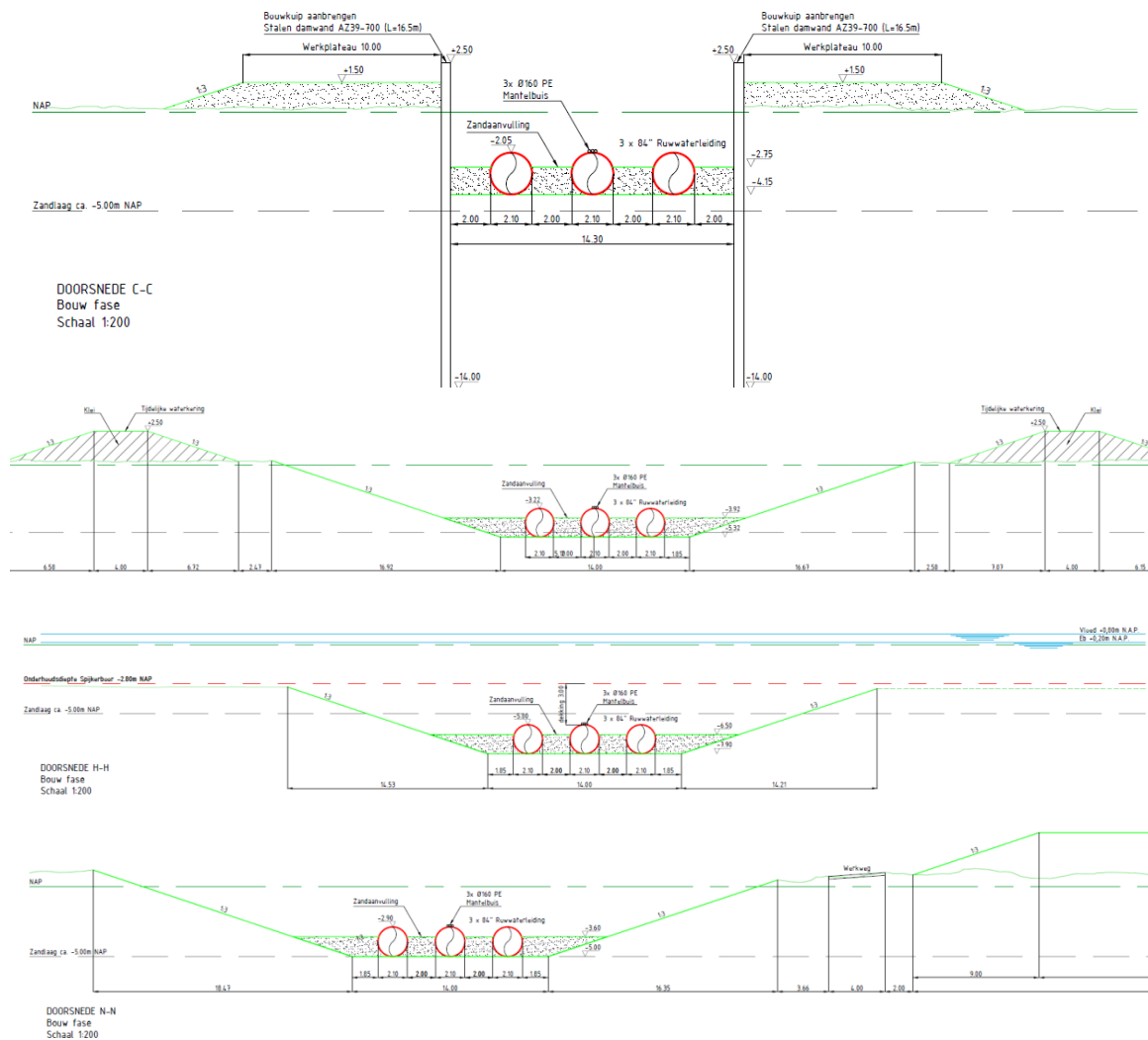
Afbeelding 14: Dwarsprofielen van de sleuf in de Fortunapolder (1 e en 2 e ), in het Spijkerboor (3 e ) op de St. Jansplaat (4 e ).
