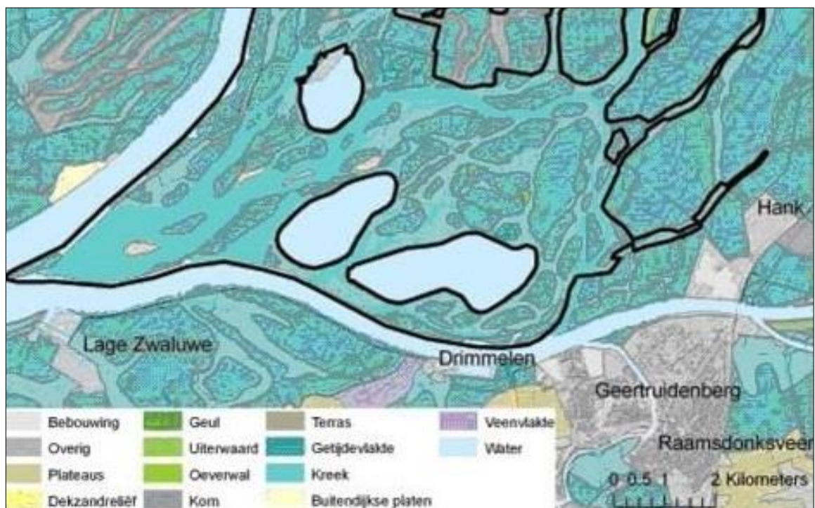
Afbeelding 18: Uitsnede geomorfologische kaart Biesbosch (Alterra, geomorfologische kaart Nederland)
