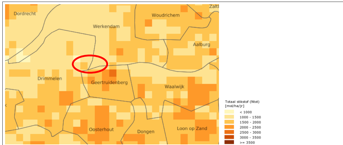
Afbeelding 32: Jaarlijkse bijdrage totaal stikstof 2016 (Bron: http://geodata.rivm.nl/gcn/RIVM )
