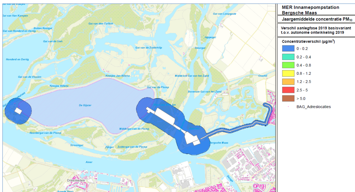
Afbeelding 34: Verschil jaargemiddelde concentratie PM 10 basisvariant (2019) t.o.v. autonome ontwikkeling
