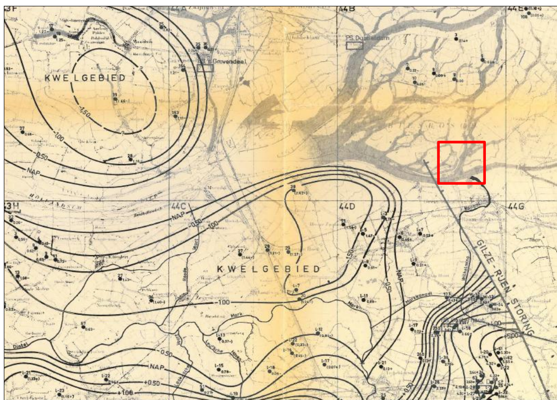
Afbeelding 22: Isohypsen van het grondwater in het eerste watervoerend pakket met onderzoeksgebied rood omkaderd (Grondwaterkaart van Nederland; Inventarisatierapport West-Brabant, kaartbladen 43 en 44 W, TNO, 1976)
