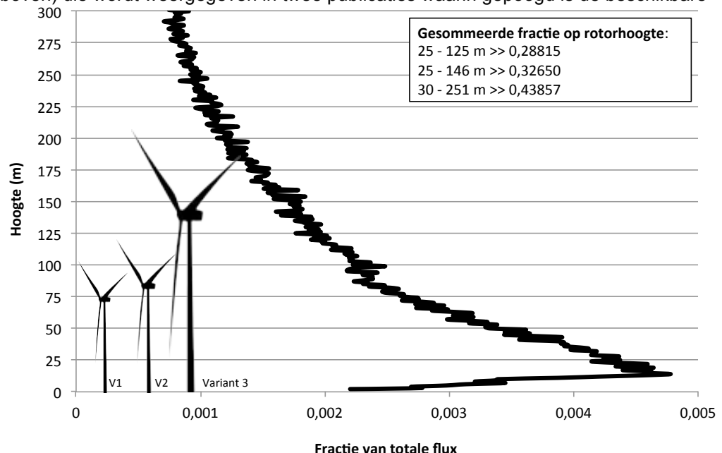
Figuur 2.20 Hoogteprofiel van zangvogeltrek tijdens oktonachten in OWEZ en daarmee aangegeven de cumulatieve fracties op rotorhoogte voor de verschillende alternatieven in windenergiegebied Borssele.
