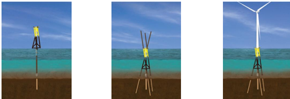
Figuur 1.10 Drie stadia in de installatie van een Twisted Jacket
