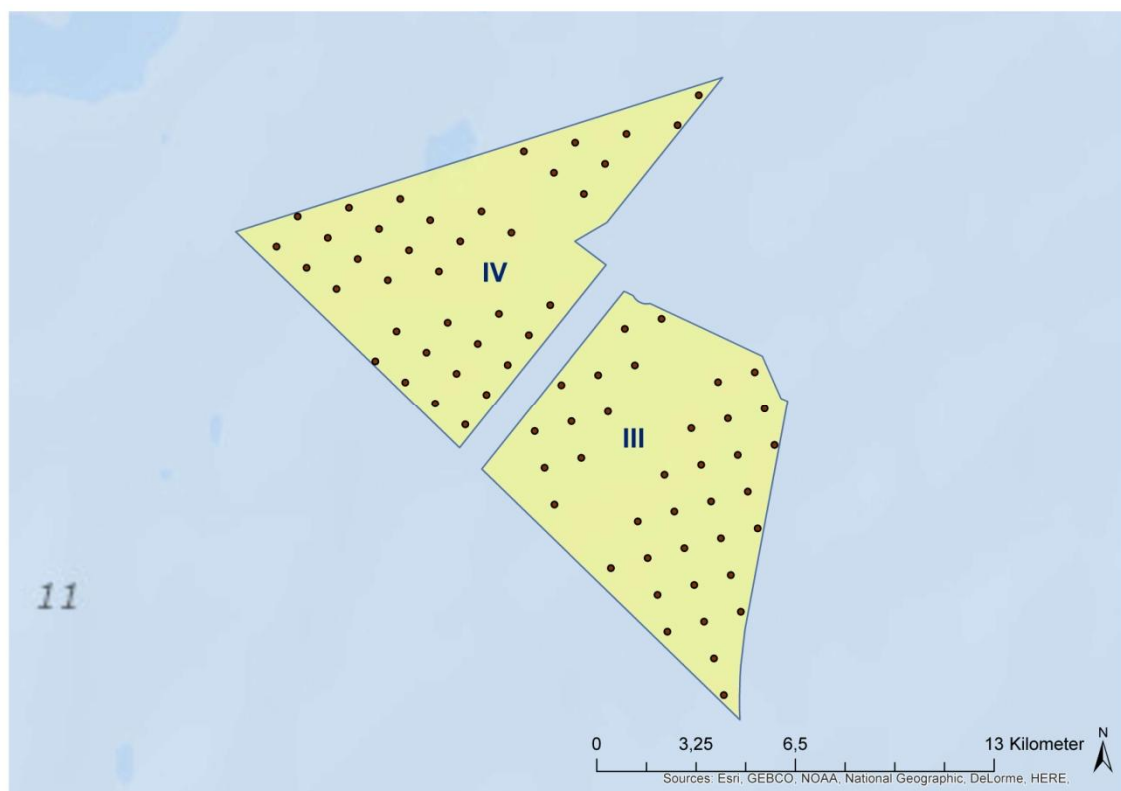
Figuur 1.3 Opstelling met 38 turbines van 10 MW
