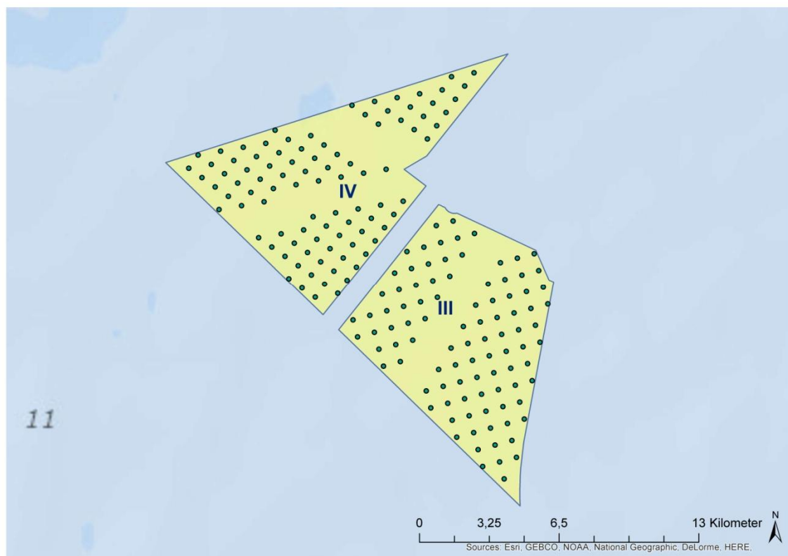
Figuur 1.2 Opstelling met 95 turbines van 4 MW
