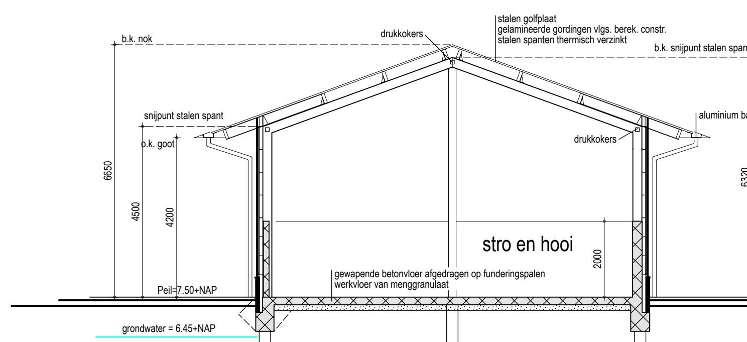
doorsnede gebouw Q
