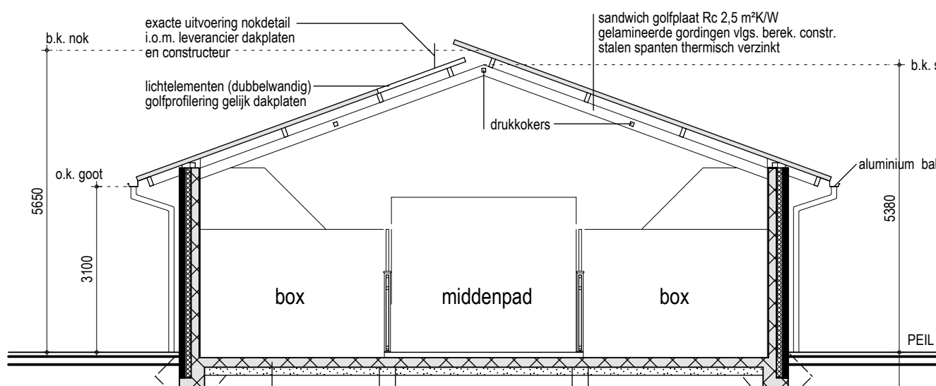
doorsnede gebouw G
