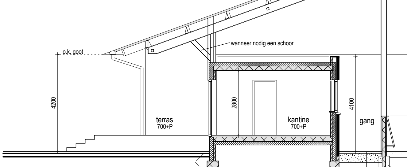
doorsnede gebouw J
