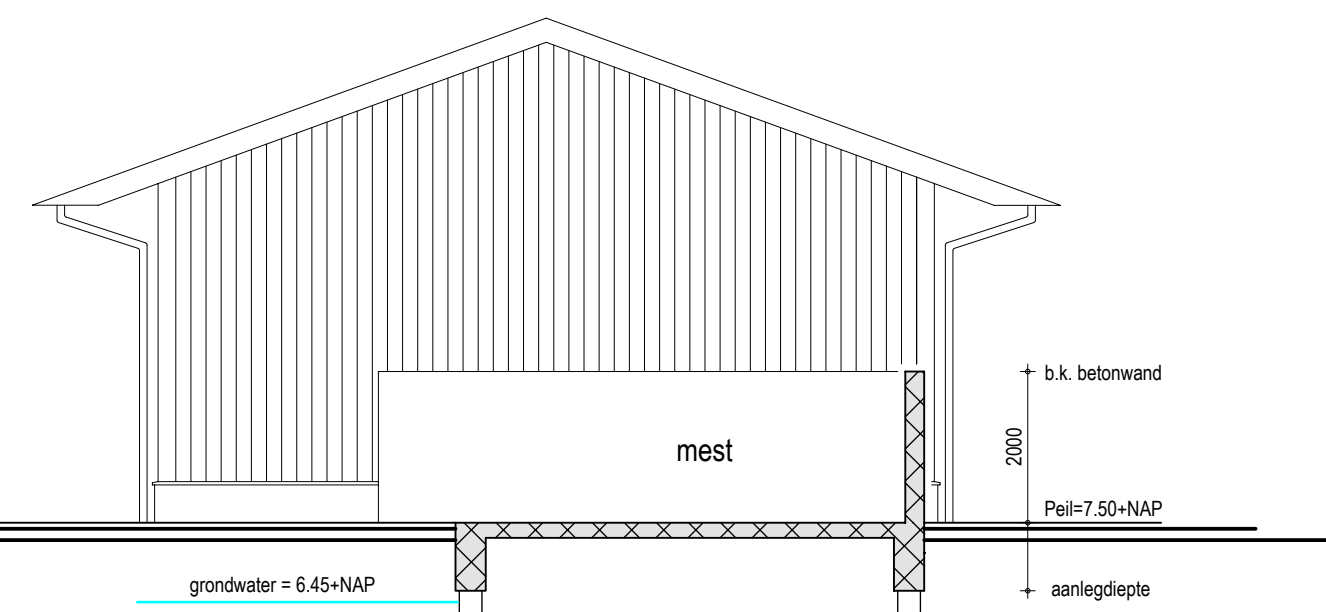
doorsnede MP mestplaat
