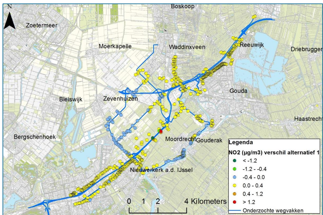
Figuur 4-9 Verschilconcentratie NO 2 alternatief 1 versus referentiesituatie
