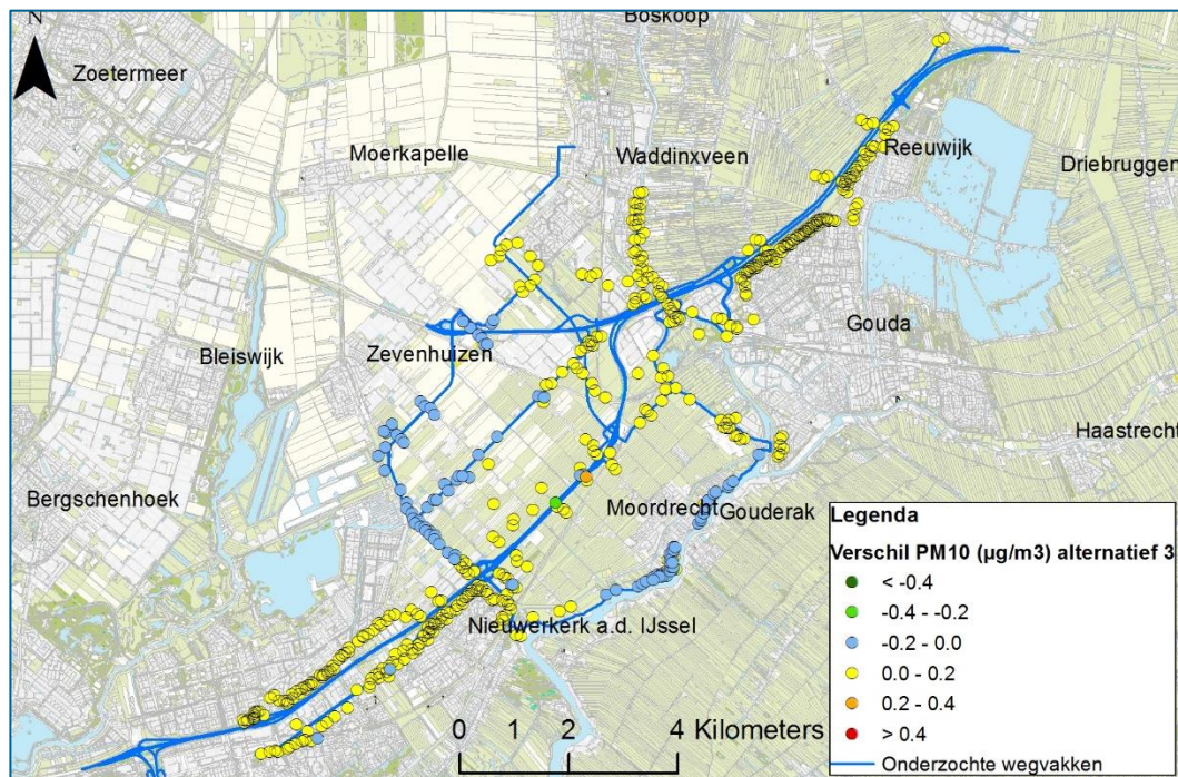
Figuur 4-12 Verschilconcentratie \text{PM}_{10} alternatief 3 versus referentiesituatie
