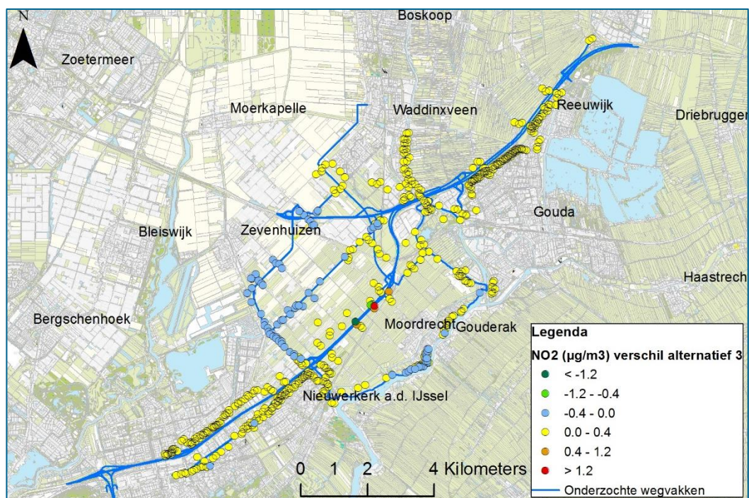
Figuur 4-11 Verschilconcentratie \text{NO}_2 alternatief 3 versus referentiesituatie
