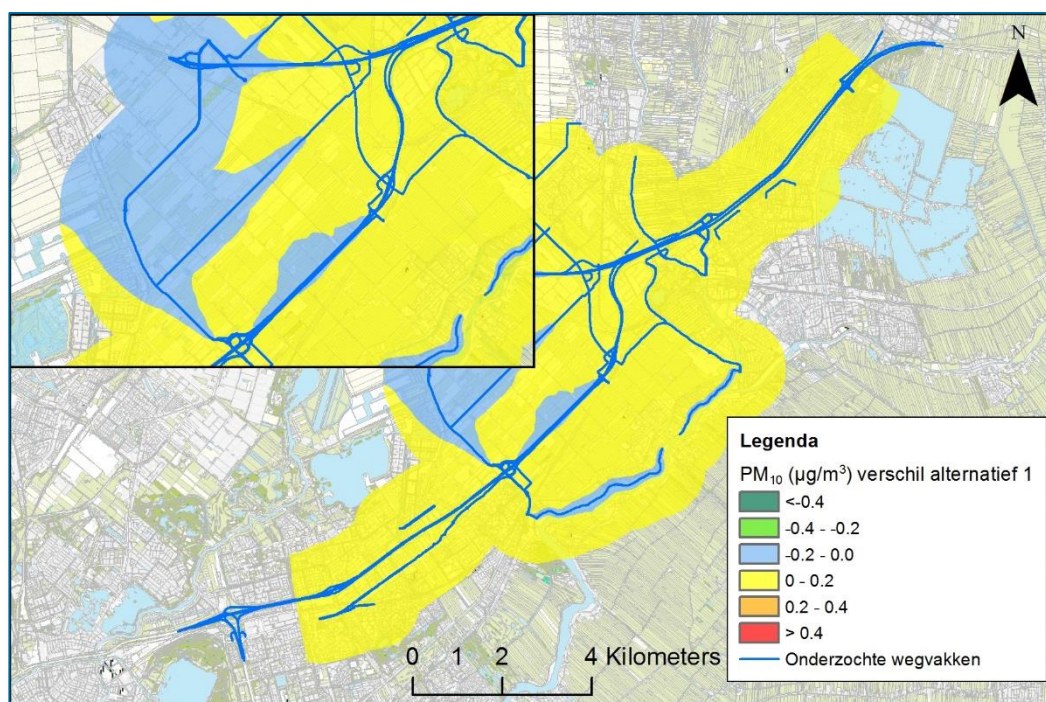
Figuur 4-14 Verschilcontouren \text{PM}_{10} alternatief 1 versus referentiesituatie
