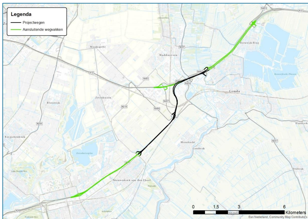
Figuur 2-1 Projectwegen en aansluitende wegvakken
