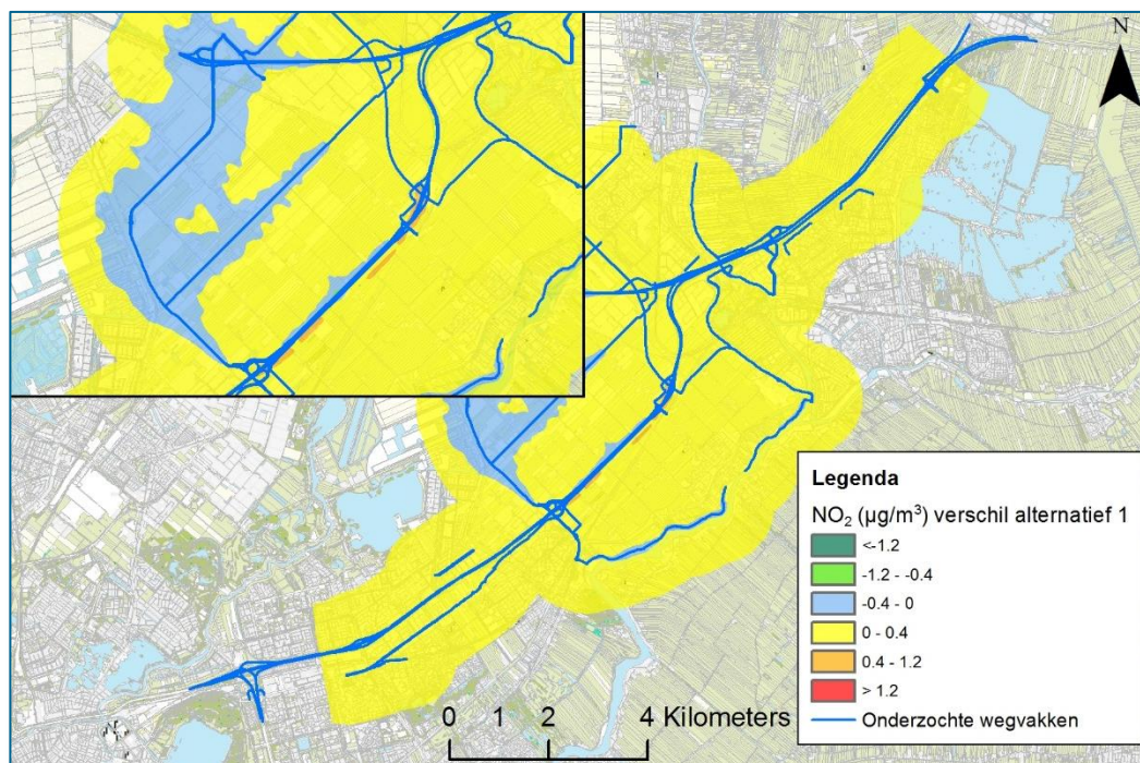
Figuur 4-13 Verschilcontouren \text{NO}_2 alternatief 1 versus referentiesituatie
