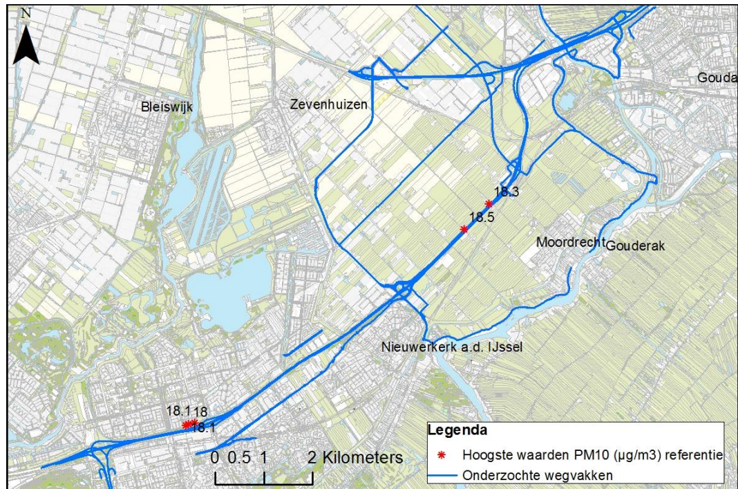
Figuur 4-4 Ligging rekenpunten 5 hoogst berekende concentraties PM 10 referentiesituatie
