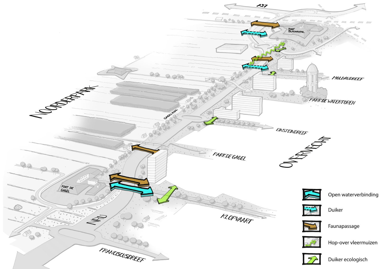
Figuur 4.5 Locatie waterlopen, faunapas-sages, hop-over Vleer-muizen en ecologisch duikers
