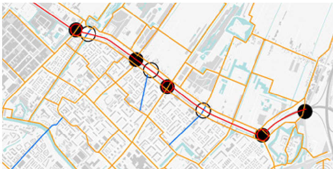
Figuur 2.4: De huidige (zwarte gevulde cirkels) en gewenste (zwarte lege cirkels) oversteken voor langzaam verkeer bij de NRU, het fietsnetwerk (oranje/blauw) en de NRU (rood)
