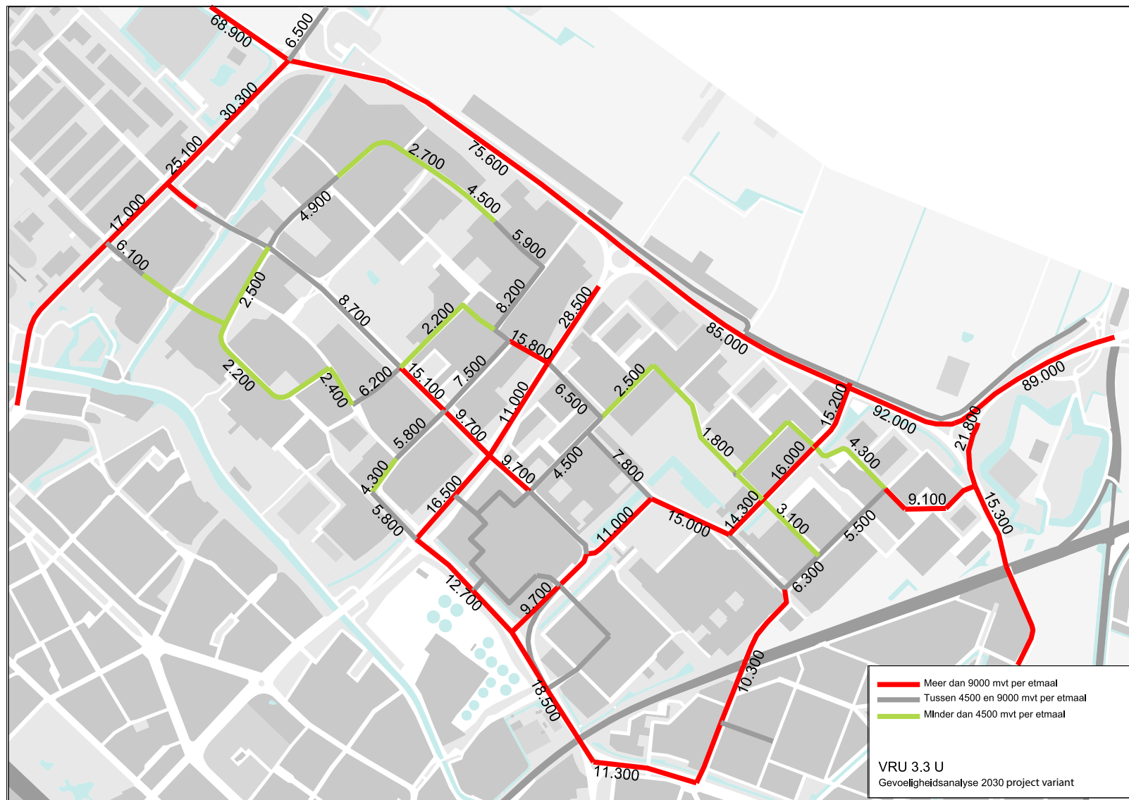
Figuur 6.7: Intensiteiten binnen Overvecht na vernieuwing NRU in 2030
