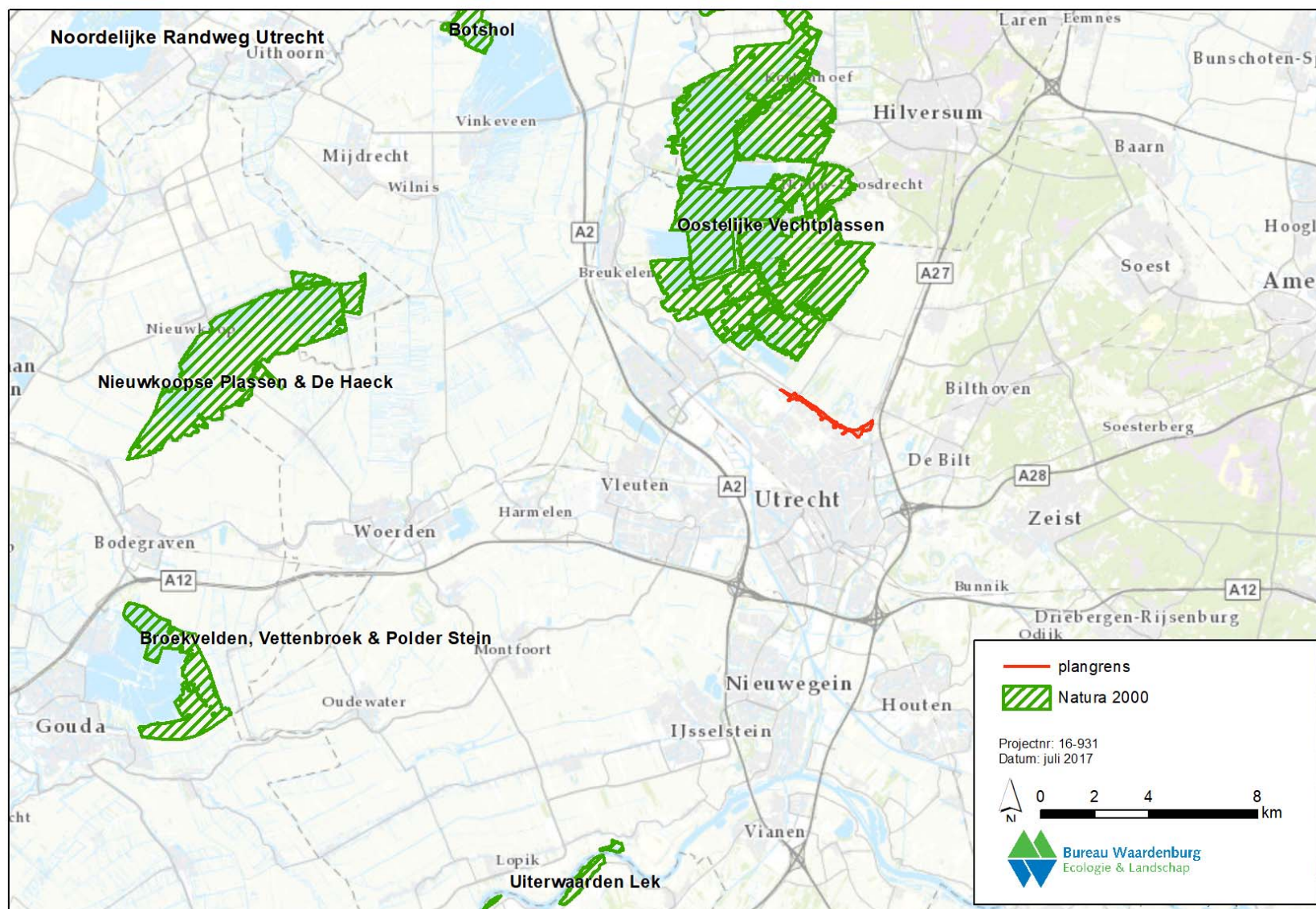
Figuur 3.13: Natura 2000-gebieden in omgeving van de NRU
