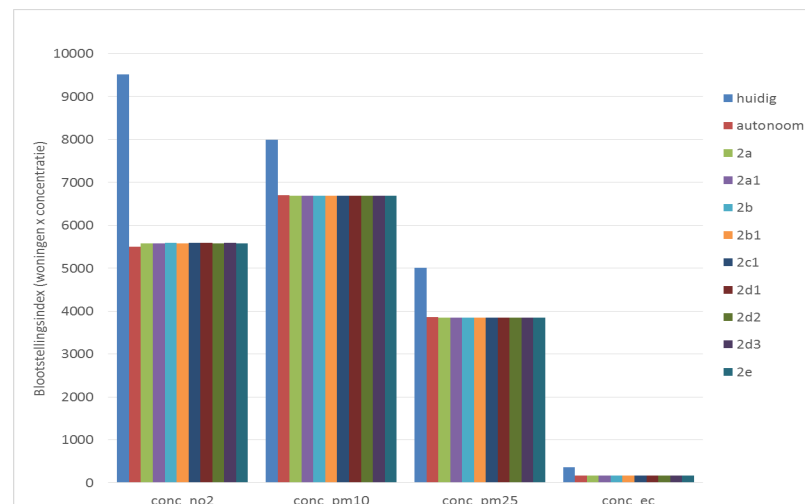
Figuur 6.20: Blootstellingsindex op de gevel van woningen langs de NRU. (Y-as is aantal bewoners * concentratie)
