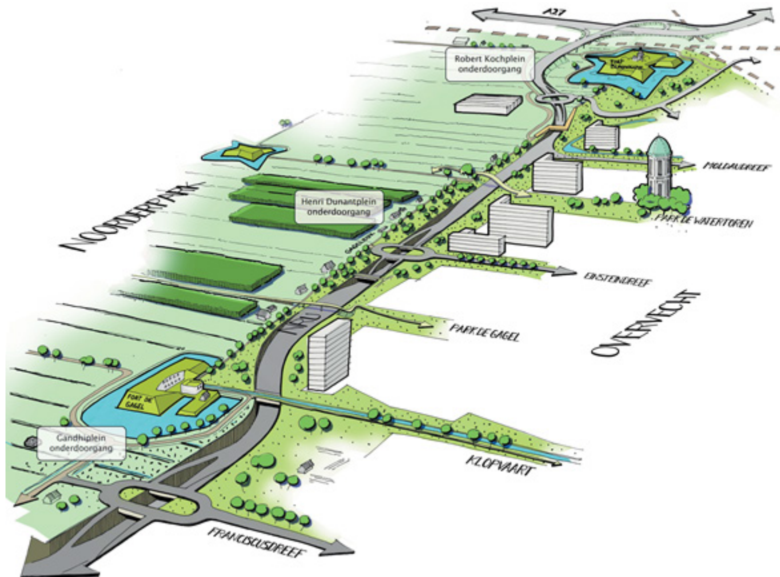
Figuur 4.1: Ontwerp NRU bij drie onderdoorgangen
