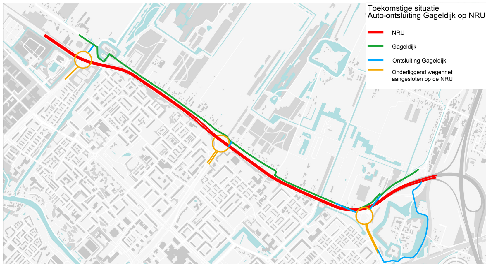
Figuur 4.3: Aansluitingen NRU op Gageldijk
