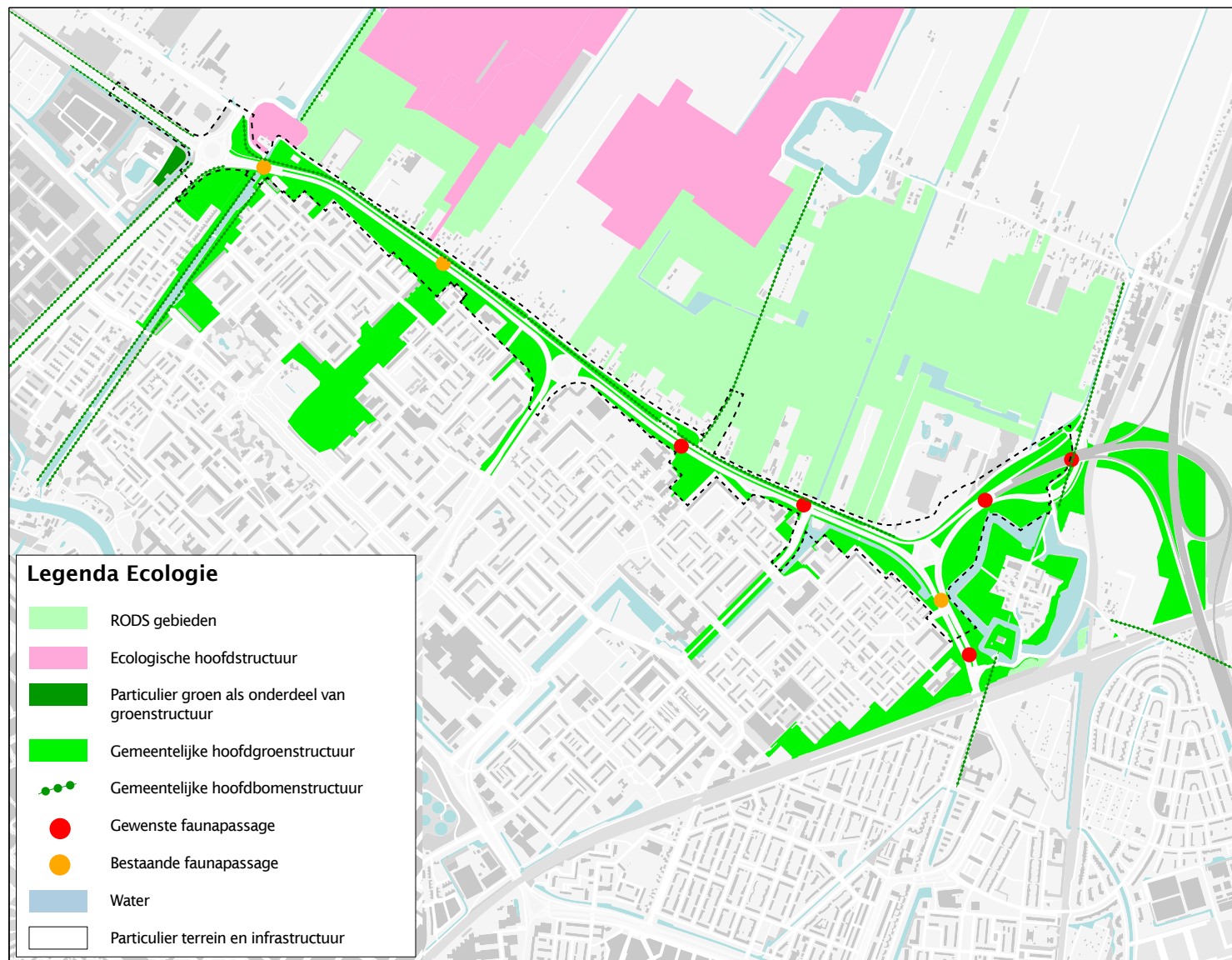
Figuur 3.14: RODS-gebieden, Natuurnetwerk Nederland (NNN)/Ecologische hoofdstructuur, gemeentelijke hoofdgroenstructuur, faunapassages (huidige situatie)
