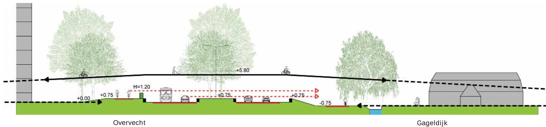
Principe dwarsprofiel voorkeursvariant
