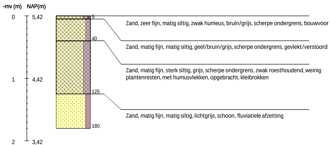
Boring 140 RD-coördinaten: 231063/503956 -
