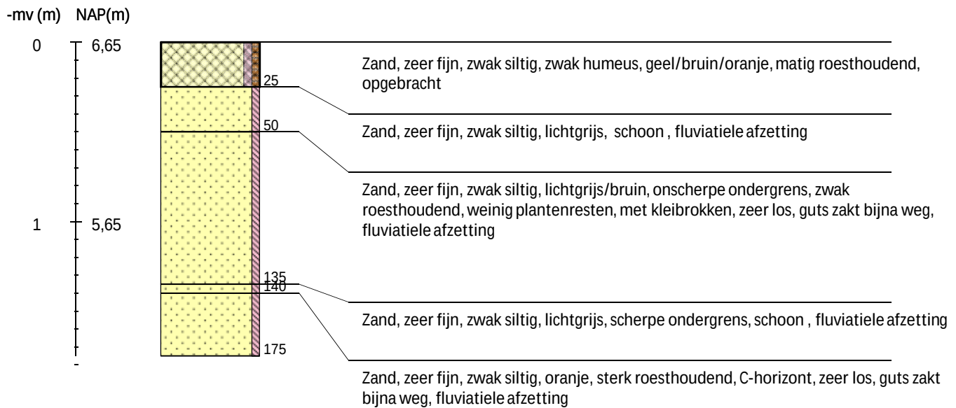
Boring 66 RD-coördinaten: 237269/507587
