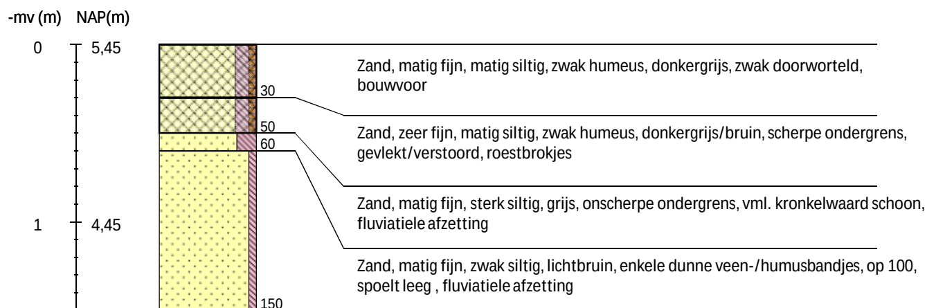
Boring 126 RD-coördinaten: 231037/504242 -
