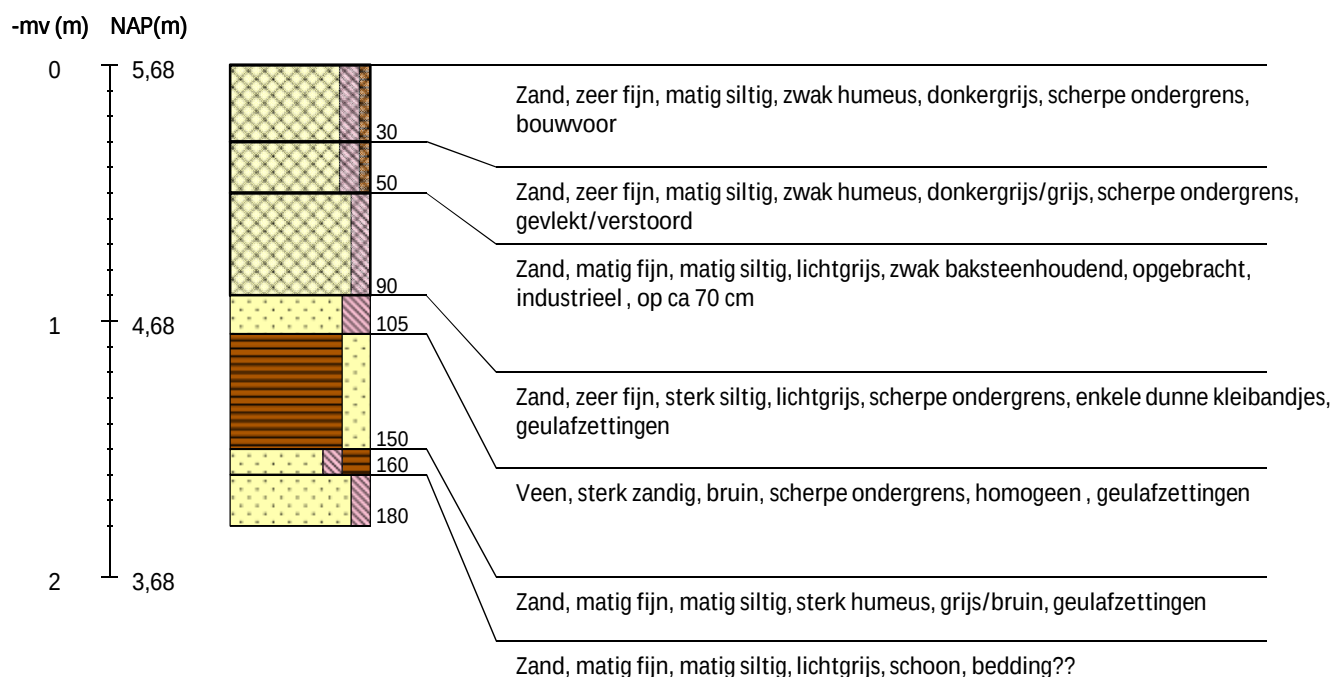
Boring 134 RD-coördinaten: 231225/504124 -
