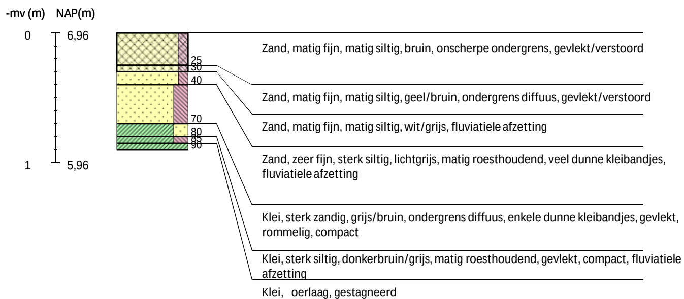
Boring 210 RD-coördinaten: 236594/506868 -
