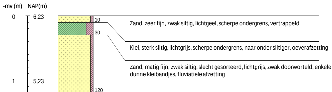
Boring 83 RD-coördinaten: 237392/508005
