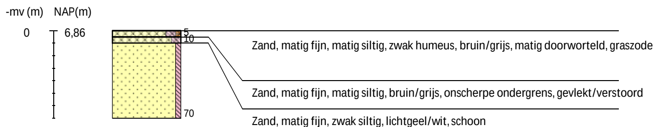
Boring 219 RD-coördinaten: 237291/507735 -
