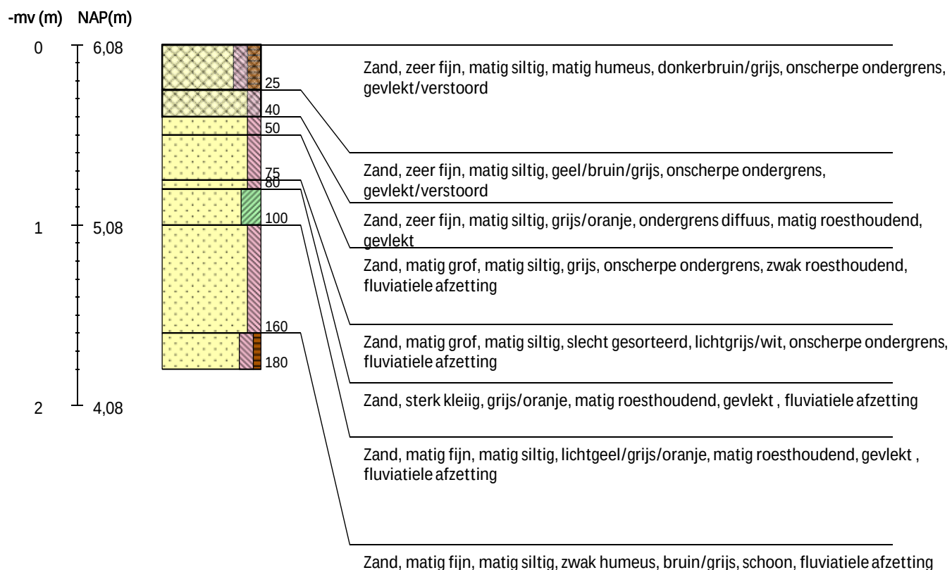
Boring 204 RD-coördinaten: 233411/504726 -
