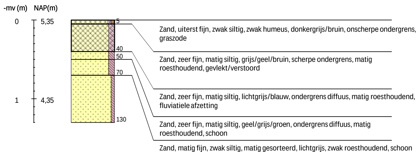
Boring 22 RD-coördinaten: 231816/503825
