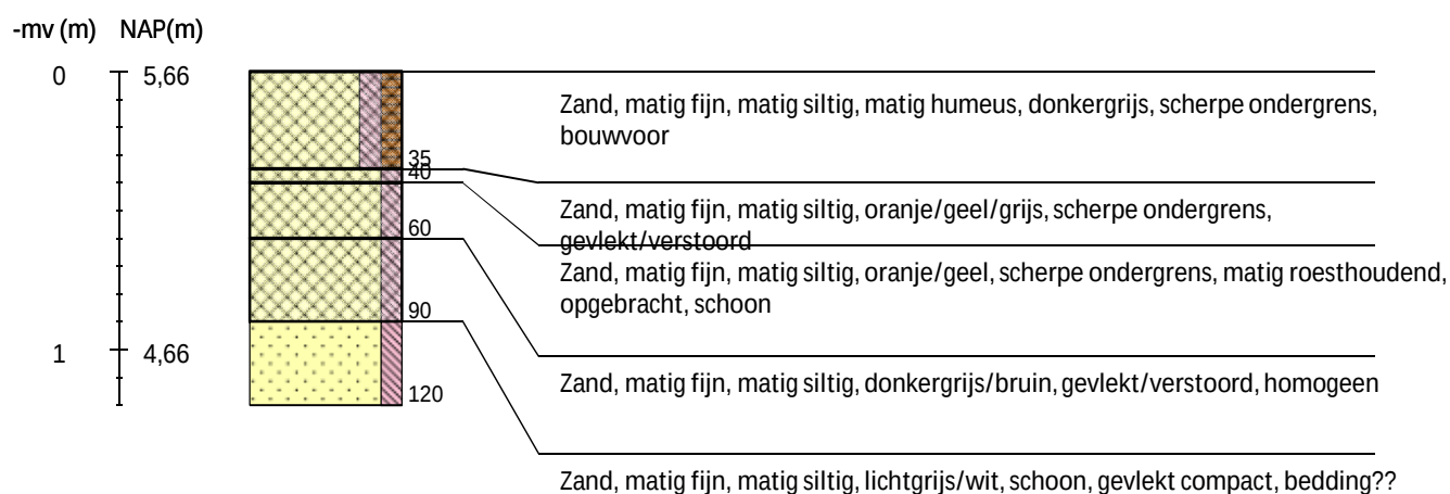
Boring 135 RD-coördinaten: 231209/504088 -
