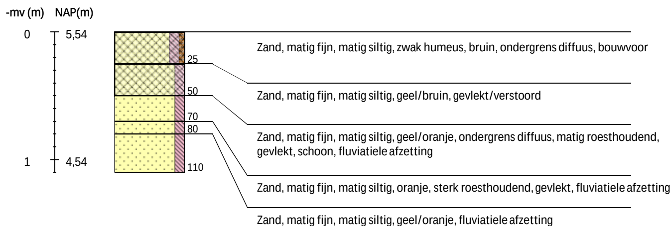
Boring 120 RD-coördinaten: 230857/504347 -
