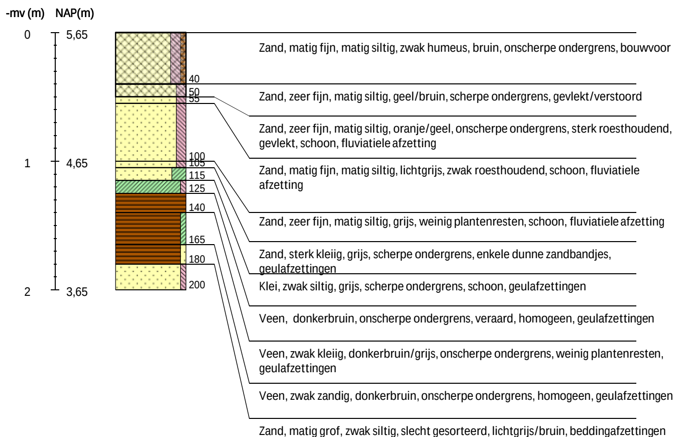
Boring 122 RD-coördinaten: 230890/504275 -
