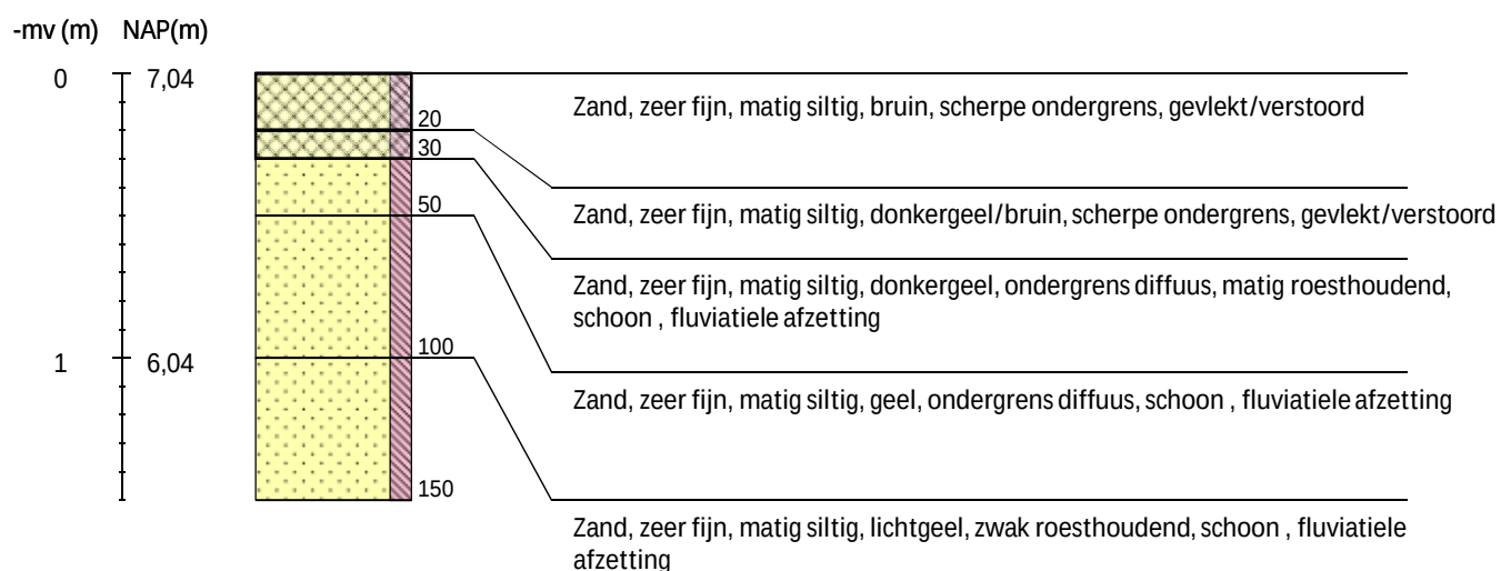
Boring 207 RD-coördinaten: 236441/506783 -
