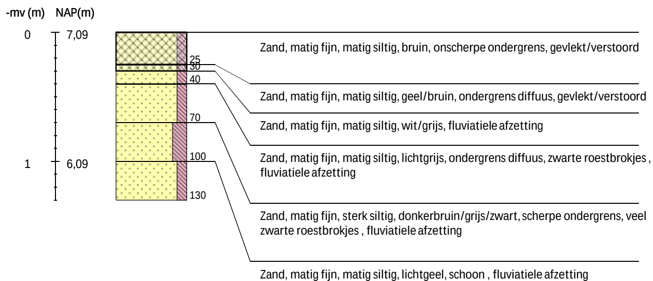
Boring 209 RD-coördinaten: 236567/506848 -
