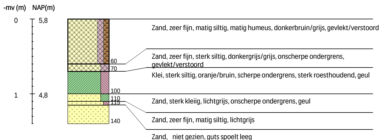
Boring 26 RD-coördinaten: 231720/503935
