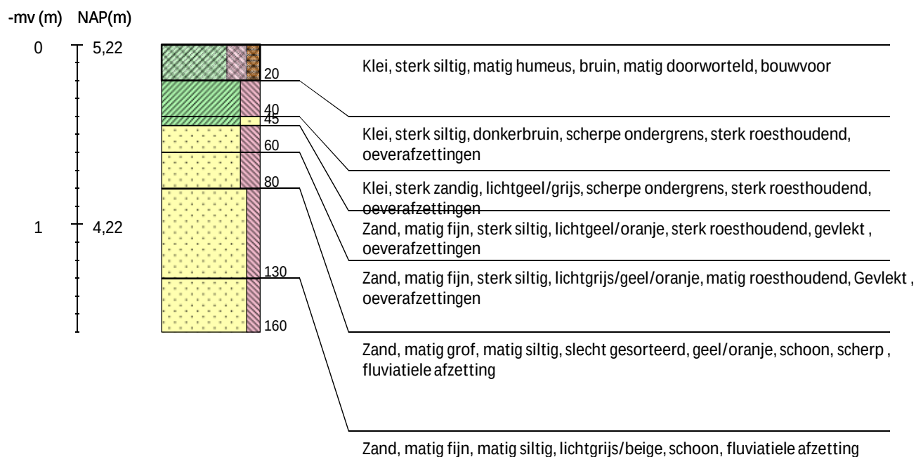
Boring 141 RD-coördinaten: 231053/503919 -
