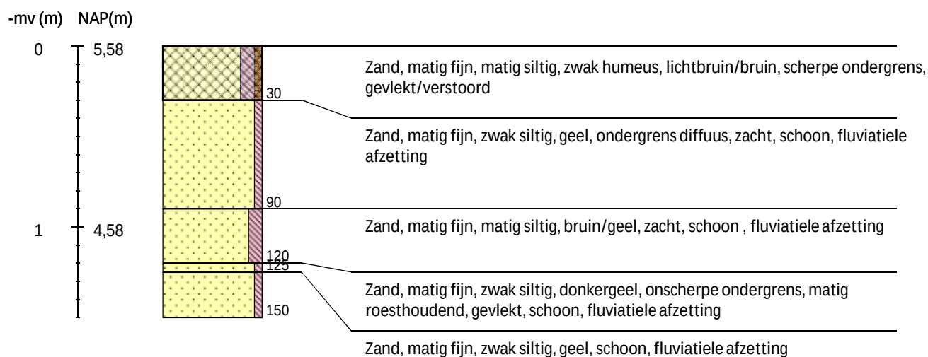
Boring 109 RD-coördinaten: 230676/504732 -
