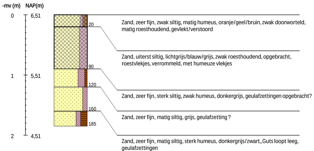
Boring 62 RD-coördinaten: 237140/507506
