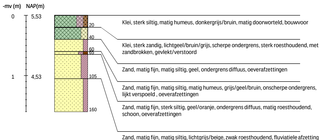
Boring 142 RD-coördinaten: 231046/503877 -
