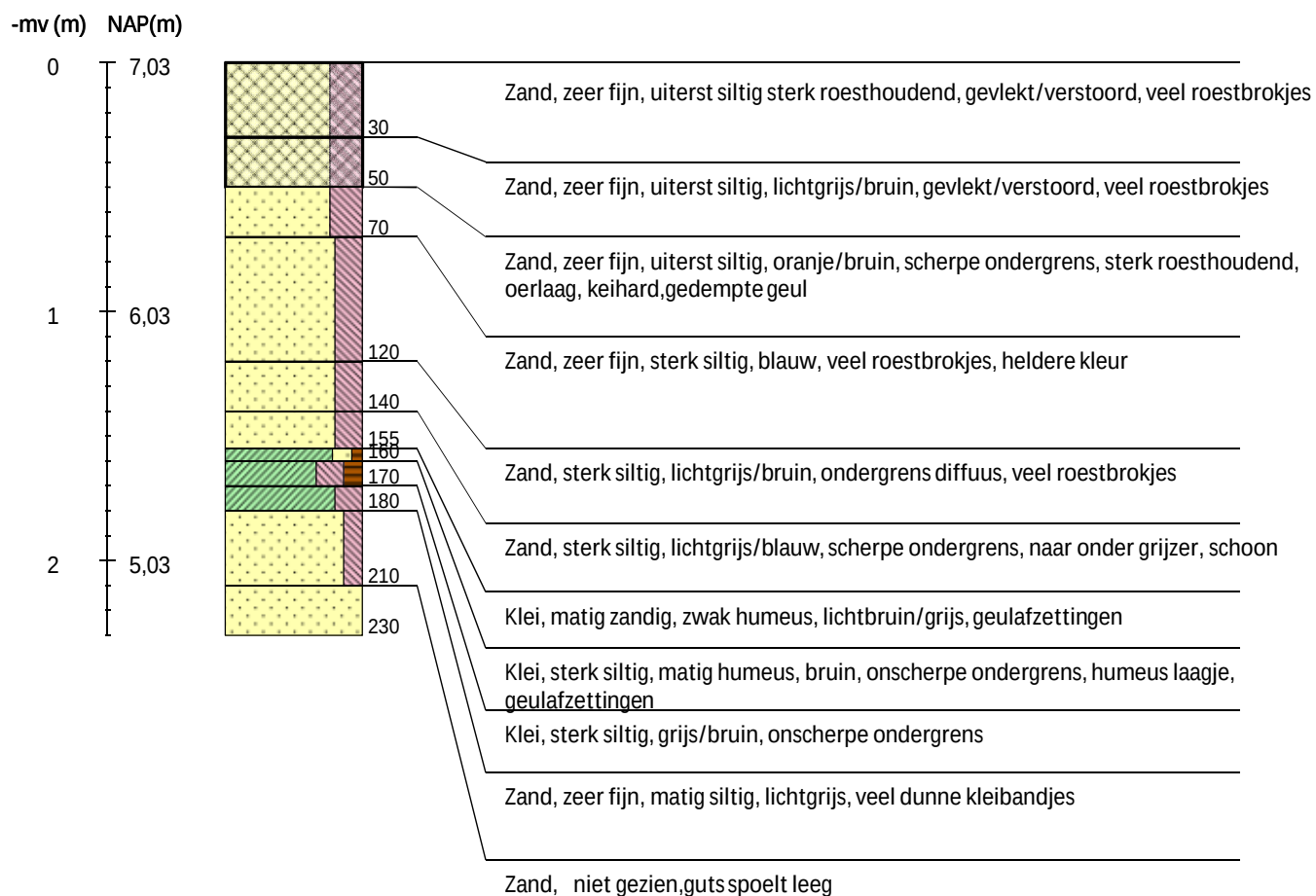
Boring 87 RD-coördinaten: 237948/508412
