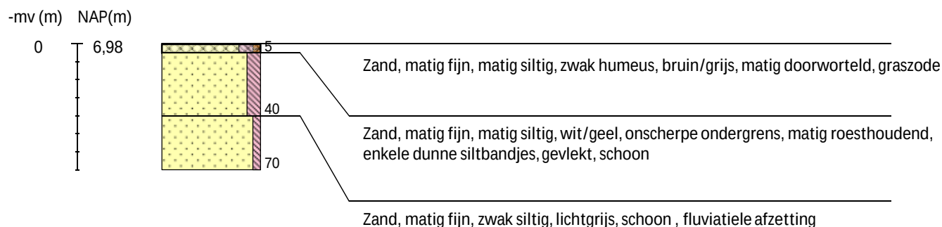
Boring 220 RD-coördinaten: 237302/507755 -
