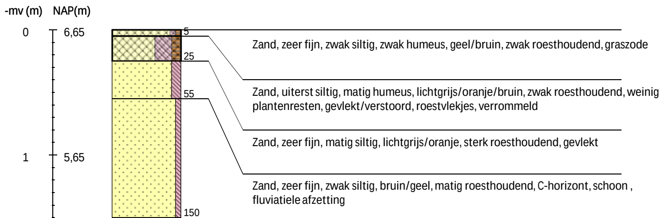
Boring 65 RD-coördinaten: 237255/507549
