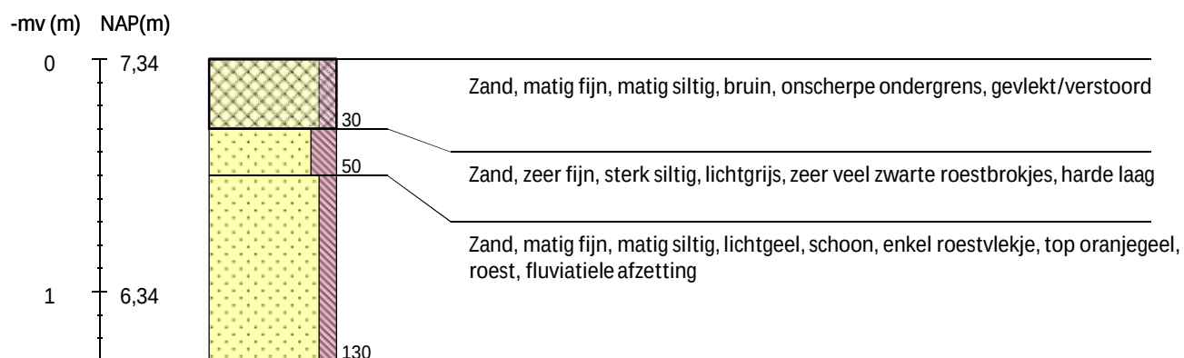
Boring 212 RD-coördinaten: 236701/506940 -
