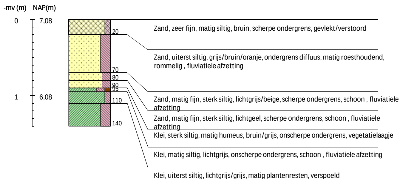
Boring 208 RD-coördinaten: 236478/506800 -
