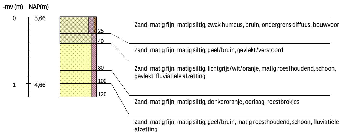
Boring 121 RD-coördinaten: 230874/504311 -
