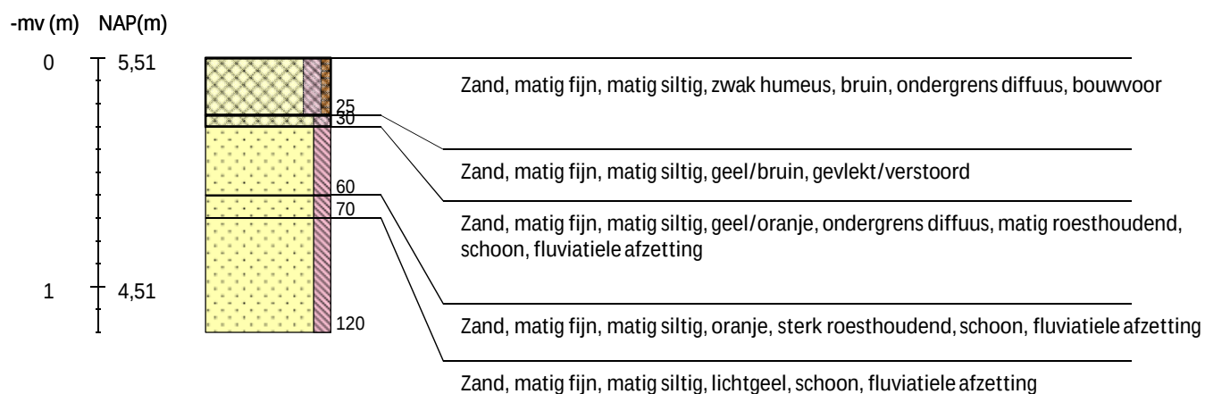
Boring 119 RD-coördinaten: 230842/504385 -
