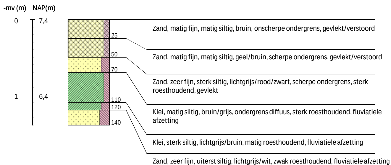
Boring 211 RD-coördinaten: 236685/506931 -
