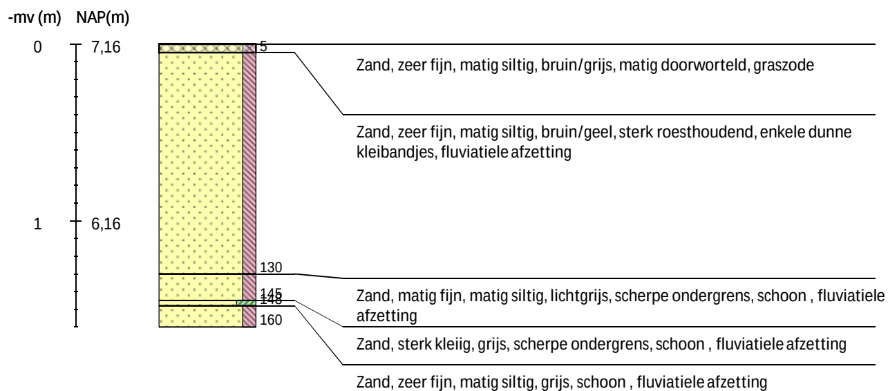
Boring 213 RD-coördinaten: 236944/507719 -
