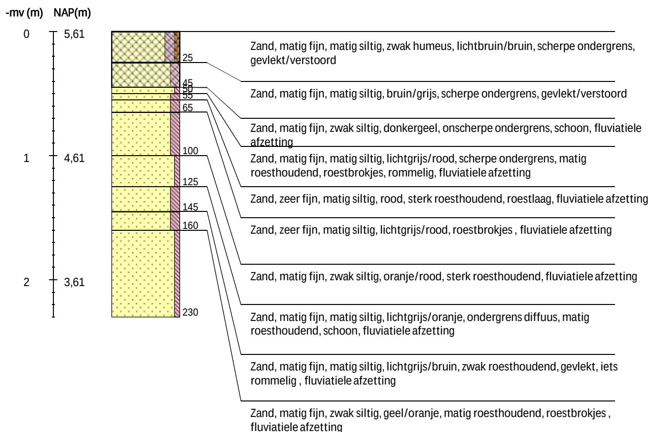
Boring 110 RD-coördinaten: 230696/504697 -
