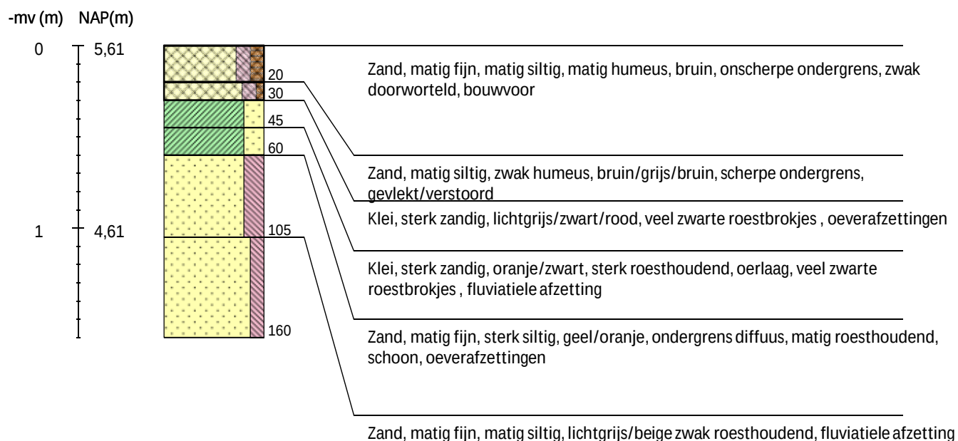
Boring 143 RD-coördinaten: 231048/503840 -
