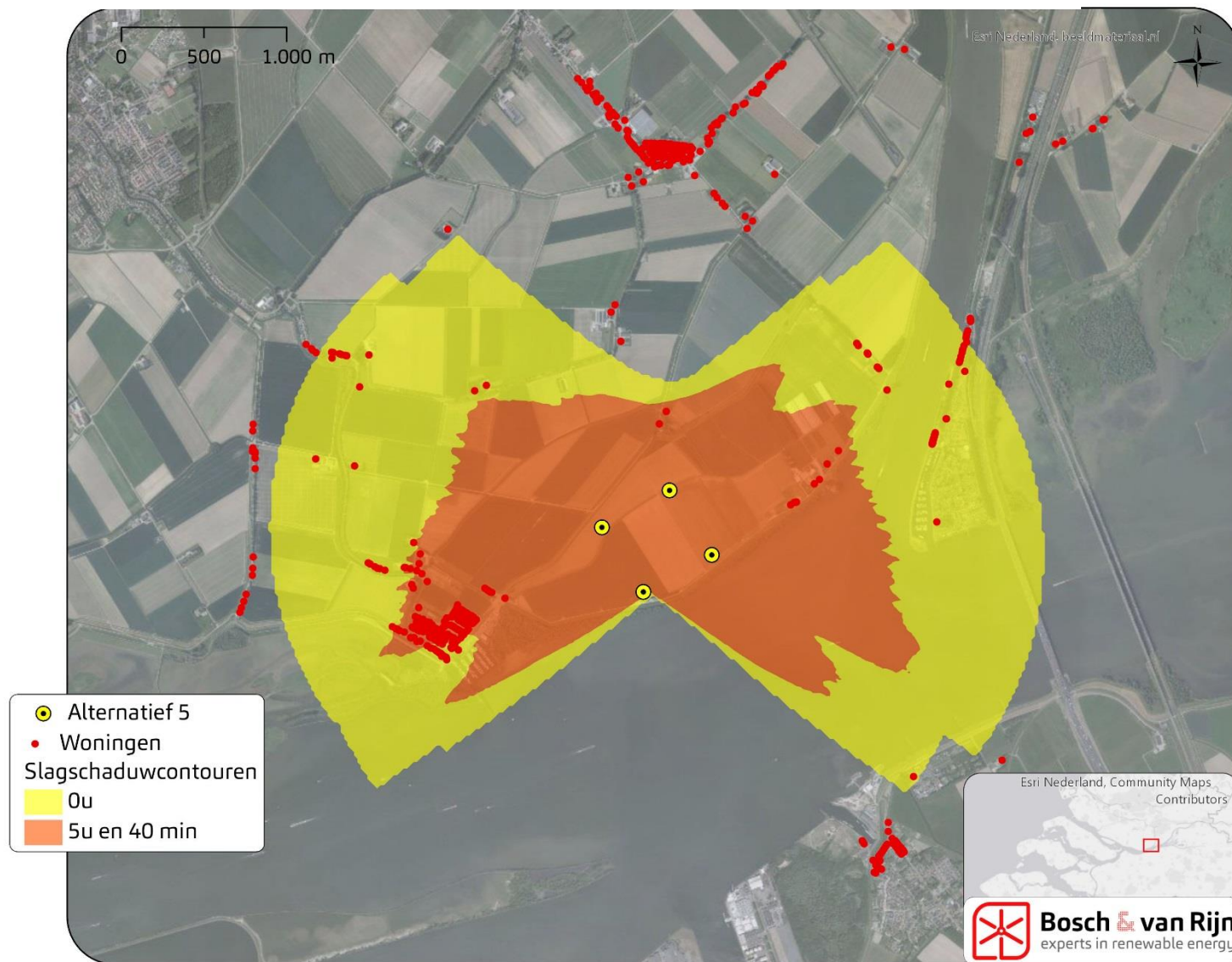
Figuur 14 Slagschaduwcontour Alternatief 5
