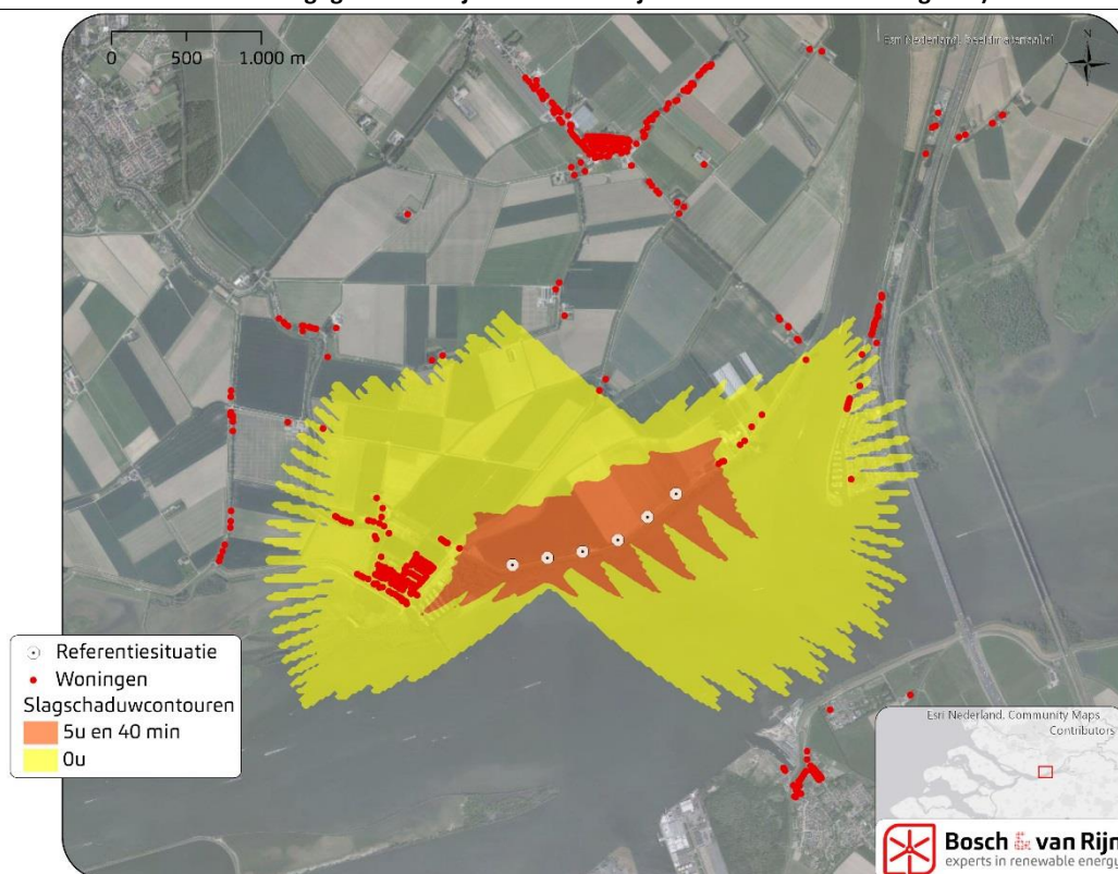
Figuur 6 5:40u en 0:00u slagschaduwcontouren van de alternatieven (volgorde: referentiesituatie, alternatief 1, alternatief 2, alternatief 3, alternatief 4 en alternatief 5). Hierbij zijn ook de gevoelige objecten van derden weergegeven. Dit zijn immers de objecten waarvoor de norm geldt.)
