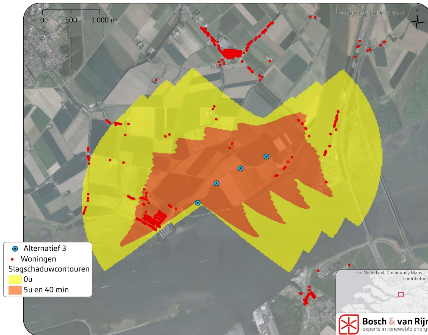
Figuur 12 Slagschaduwcontour Alternatief 3
