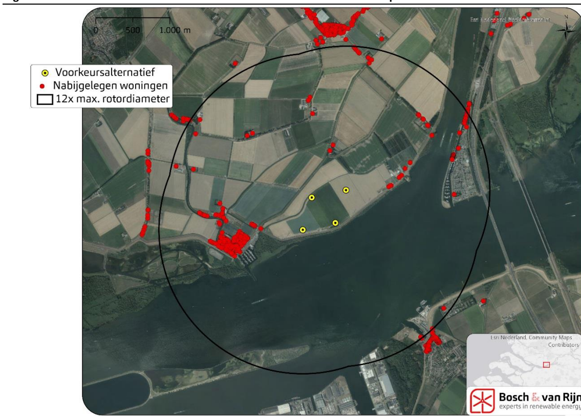
Figuur 7 Windturbinelocaties van het voorkeursalternatief van Windpark Oude Mol
