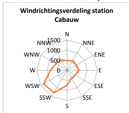
Figuur 5 Windroos van meteorostation Cabauw op 140 meter hoogte.
