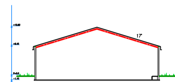
DOORSNEDE STAL 3
