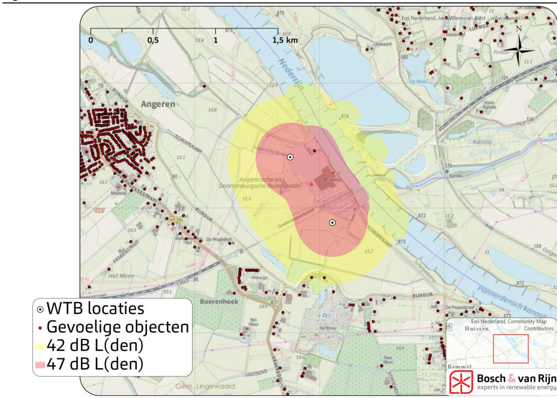
Figuur 8 L den 47- en 42 dB-contour van Alternatief 2.
