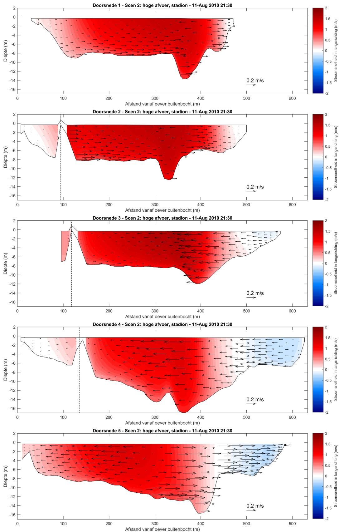
Figuur 3.9: Dwarsdoorsneden op vijf locaties (zie Figuur 3.1) met de snelheid langs de as van de rivier in de kleurschaal, waarbij de rode kleur een snelheid in benedenstroomse richting (richting de Noordzee) weergeeft. De snelheid dwars op de as van de rivier is weergegeven met de pijlen.
