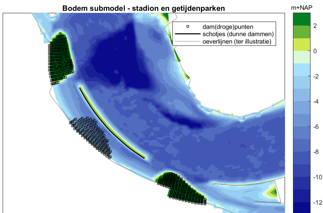
Figuur 2.4: Bodem en dampunten in het model van de variant met het stadion, de langsdam en de getijdenparken.
