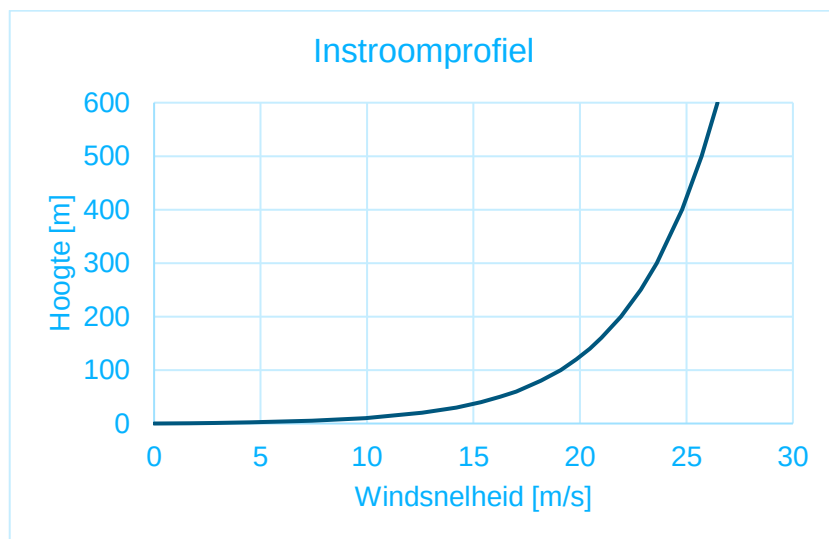
Afbeelding 2-6: Instroomprofiel wind
