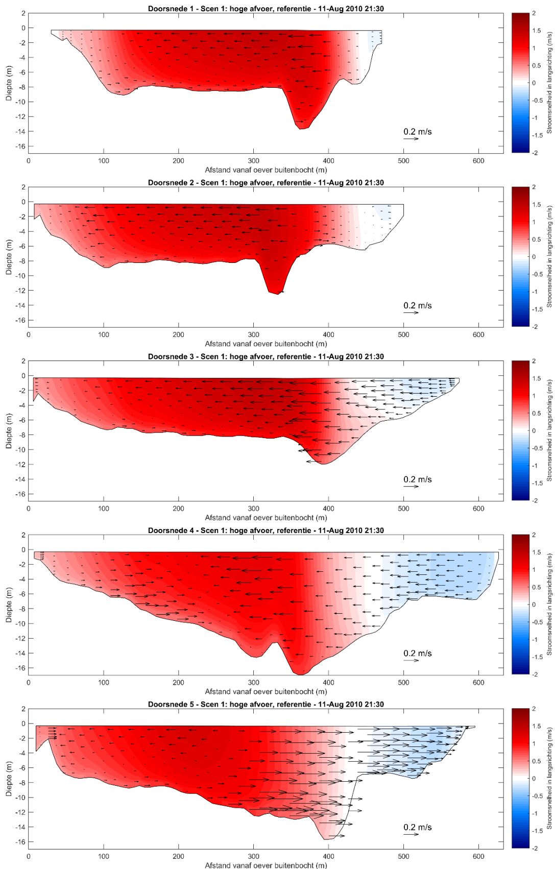
Figuur 3.4: Dwarsdoorsnedes op vijf locaties (zie Figuur 3.1) met de snelheid langs de as van de rivier in de kleurschaal, waarbij de rode kleur een snelheid in benedenstroomse richting (richting de Noordzee) weergeeft. De snelheid dwars op de as van de rivier is weergegeven met de pijlen.
