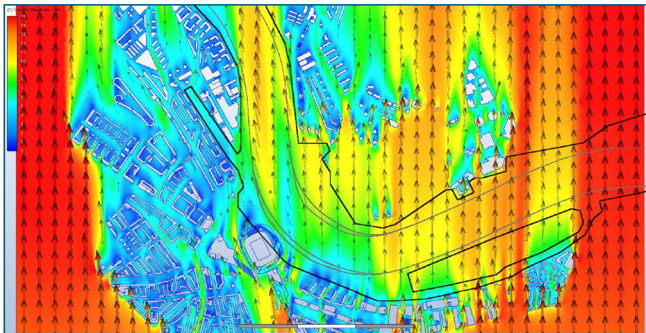
Figuur 4-12 Toekomstige situatie Z wind op 6 m hoogte
