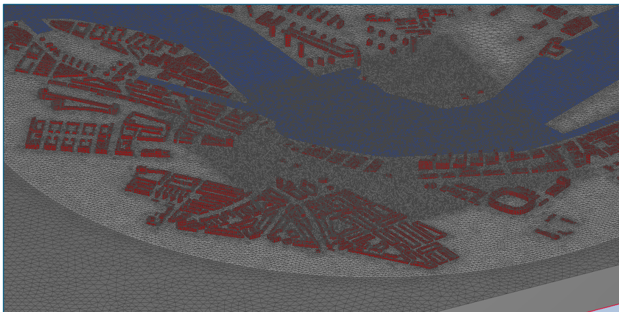
Afbeelding 3-1: Overzicht rekenrooster
