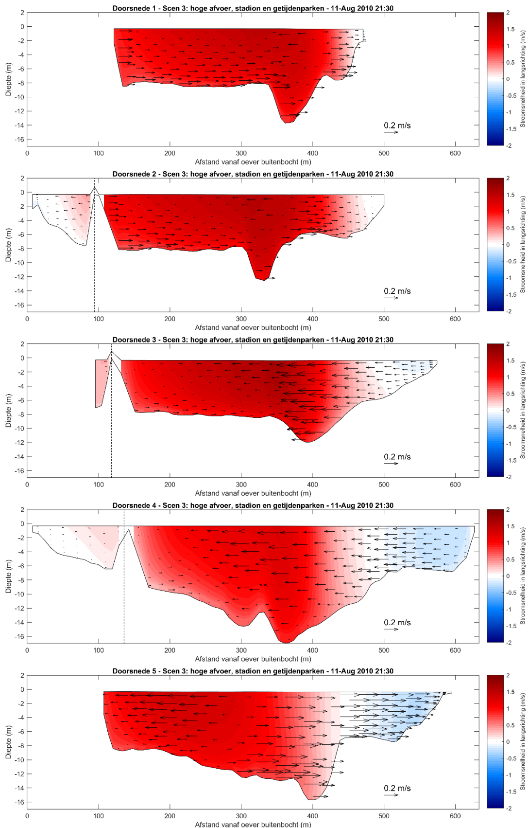
Figuur 3.17: Dwarsdoorsnedes op vijf locaties (zie Figuur 3.1) met de snelheid langs de as van de rivier in de kleurschaal, waarbij de rode kleur een snelheid in benedenstroomse richting (richting de Noordzee) weergeeft. De snelheid dwars op de as van de rivier is weergegeven met de pijlen.
