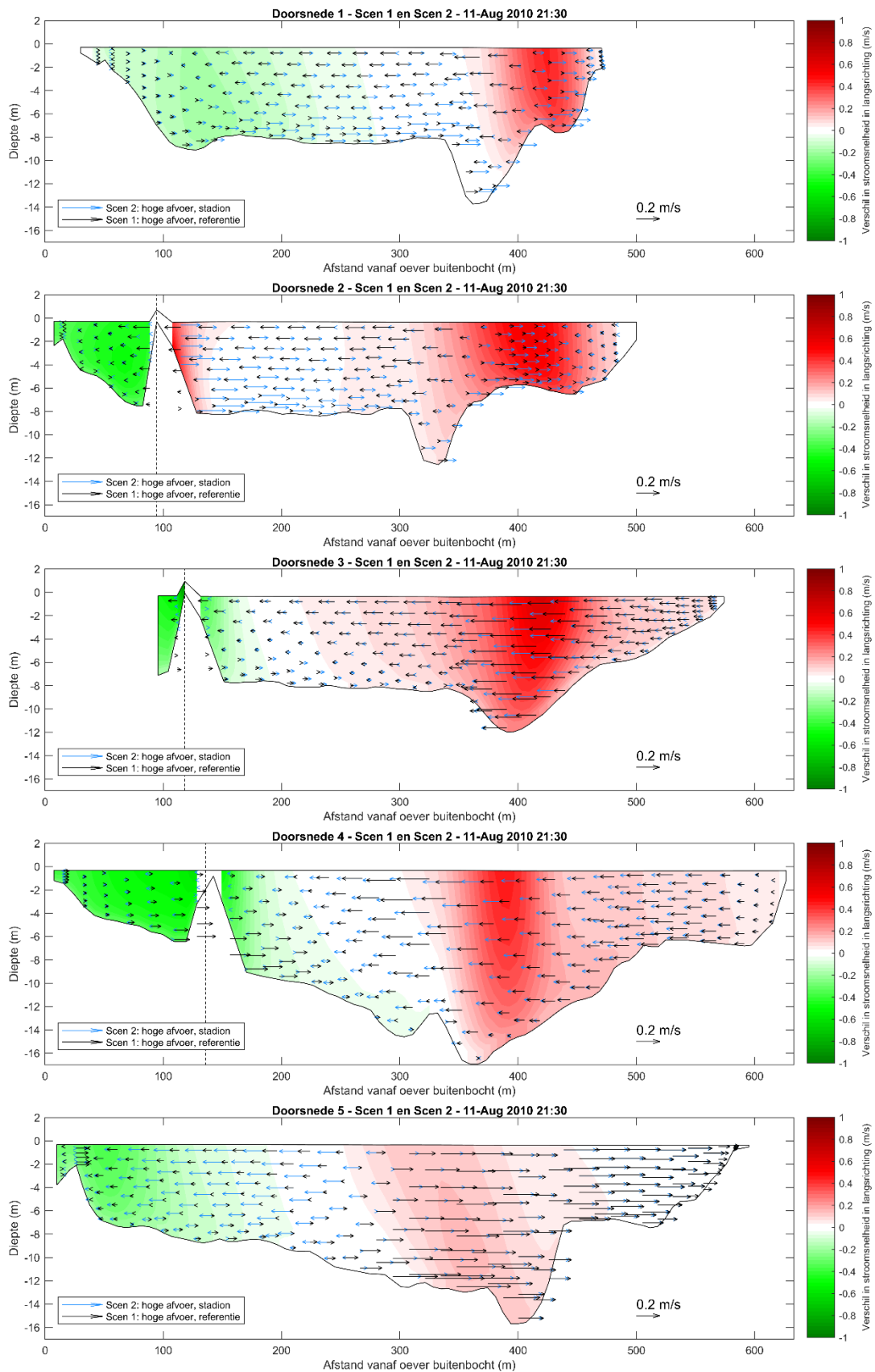
Figuur 3.10: Dwarsdoorsneden op vijf locaties (zie Figuur 3.1) met het verschil in snelheid langs de as van de rivier in de kleurschaal tussen het referentie scenario en het scenario met het stadion en de langsdam. De snelheid dwars op de as van de rivier is weergegeven met de pijlen.
