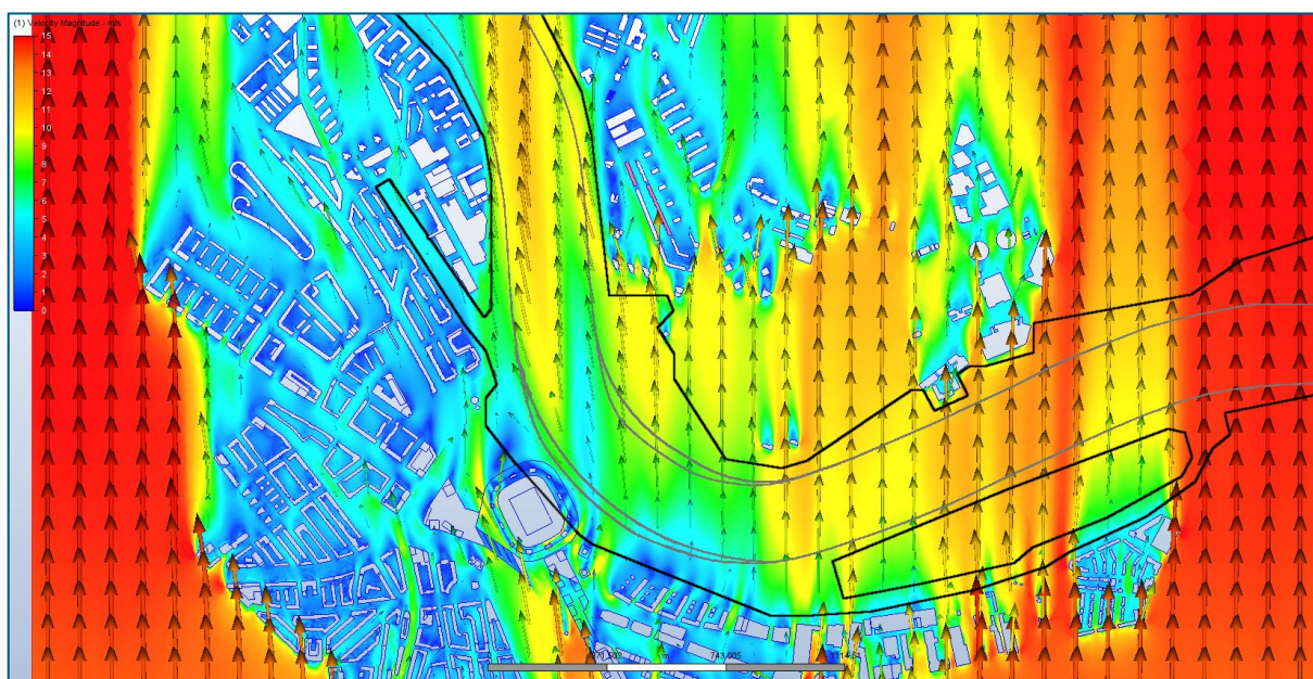
Afbeelding 4-4: overzicht windvector 6m hoogte, situatie nieuw, S.
