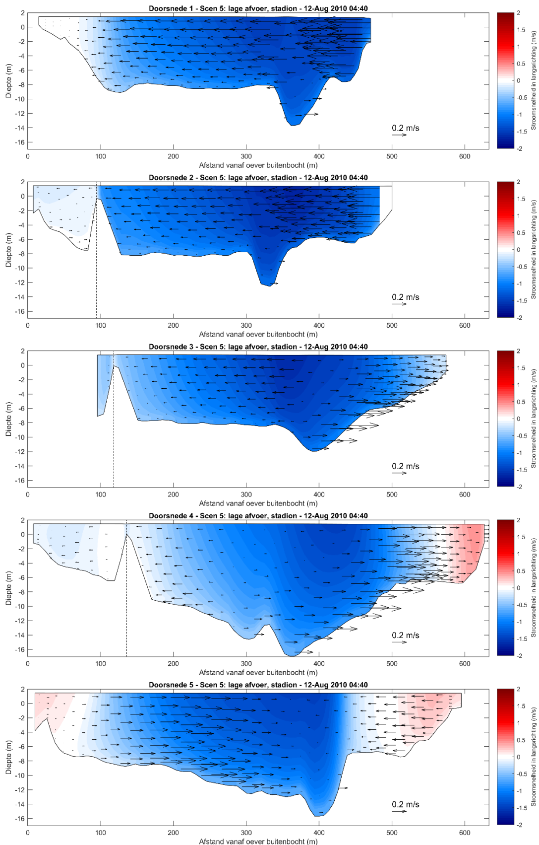
Figuur 3.26: Dwarsdoorsnedes op vijf locaties (zie Figuur 3.1) met de snelheid langs de as van de rivier in de kleurschaal, waarbij de rode kleur een snelheid in benedenstroomse richting (richting de Noordzee) weergeeft. De snelheid dwars op de as van de rivier is weergegeven met de pijlen.
