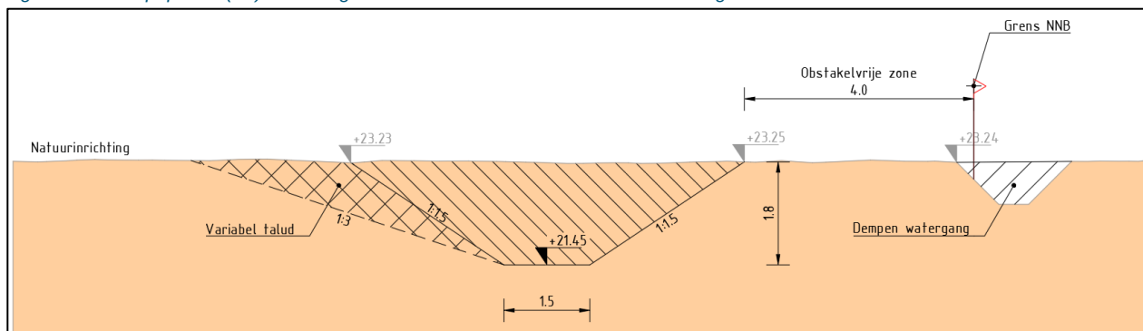
Figuur 24: Principeprofiel (P2) omleiding BZ42 & BZ57 tussen bestaande BZ42 en te dempen BERE-0329
