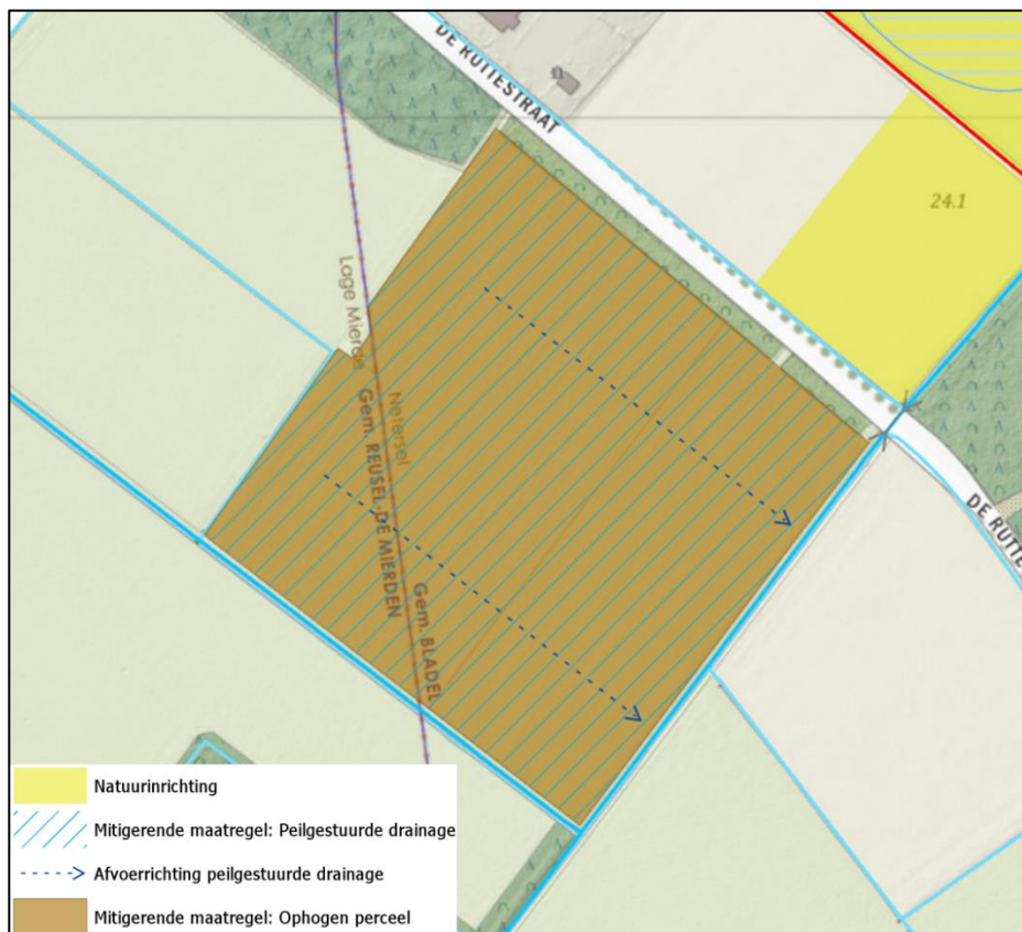
Figuur 42: Overzicht en afwateringsrichting peilgestuurde drainage MDE02-K- 101, MDE02-K-100, BDL01-L-25 en BDL01-L-24
