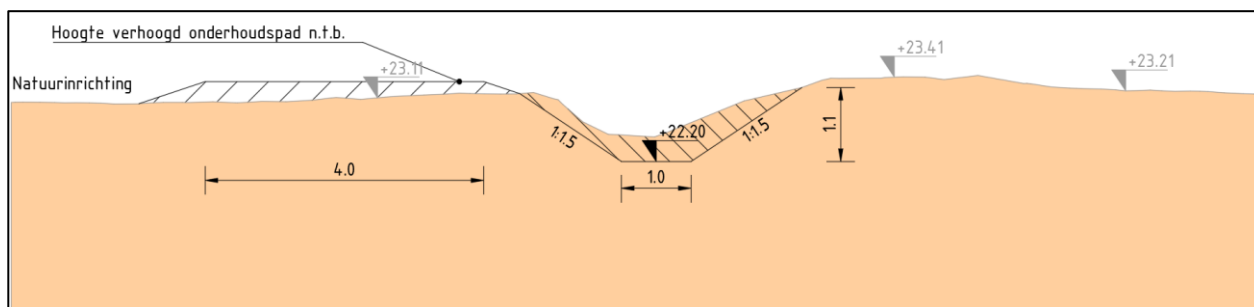
Figuur 23: Principeprofiel (P1) omleiding BZ42 & BZ57 tussen uitstroom overkluizing en bestaande BZ42
