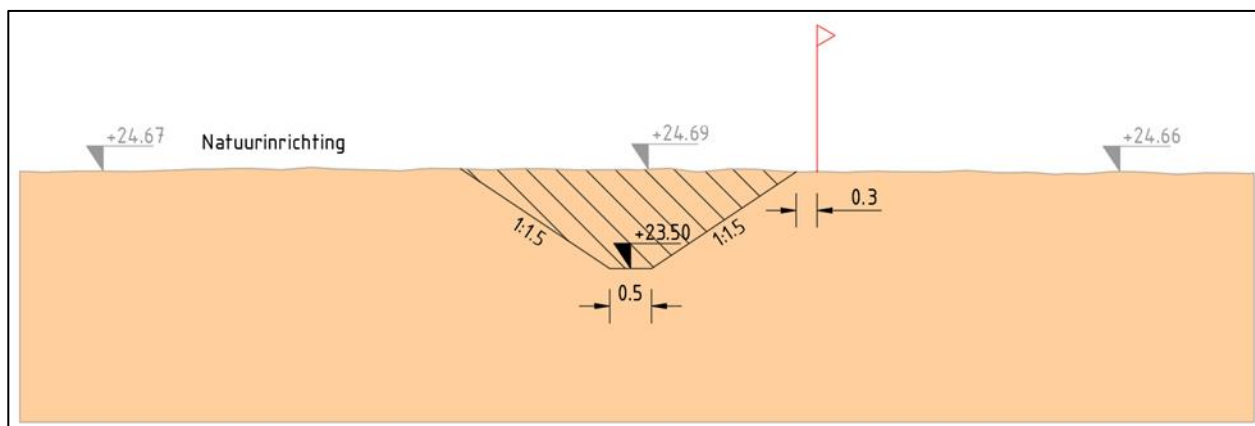
Figuur 20: Principeprofiel P1 omleiding ten zuiden van de Mispelindse Heide ter hoogte van de Beersdijk
