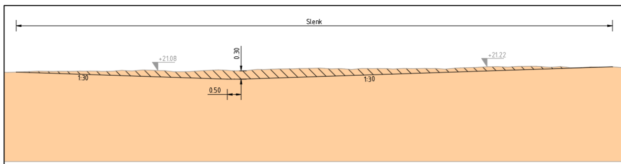
Figuur 46: Principeprofiel aan te brengen slenk op zuidelijk perceel
