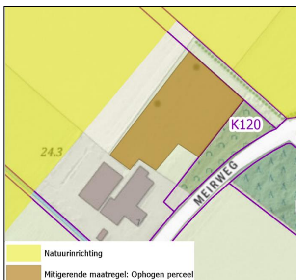
Figuur 38: Gedeeltelijke ophoging perceel MDE-K-116
