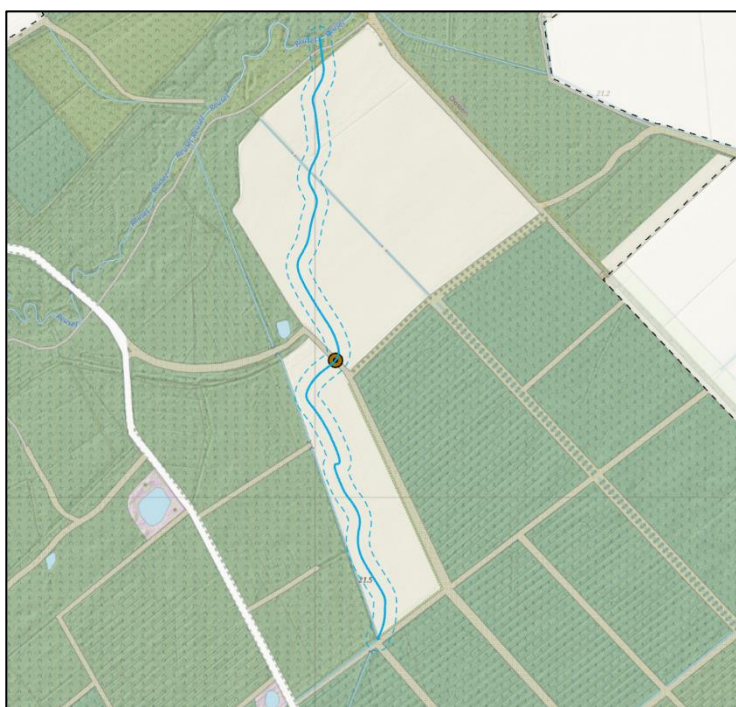
Figuur 45: Overzicht indicatieve locatie aan te brengen slenk met voorde
