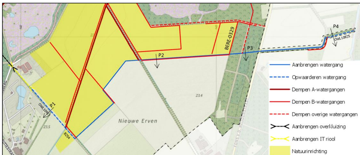
Figuur 22: Overzicht benodigde maatregelen t.b.v. aan te brengen omleiding BZ42 en BZ57
