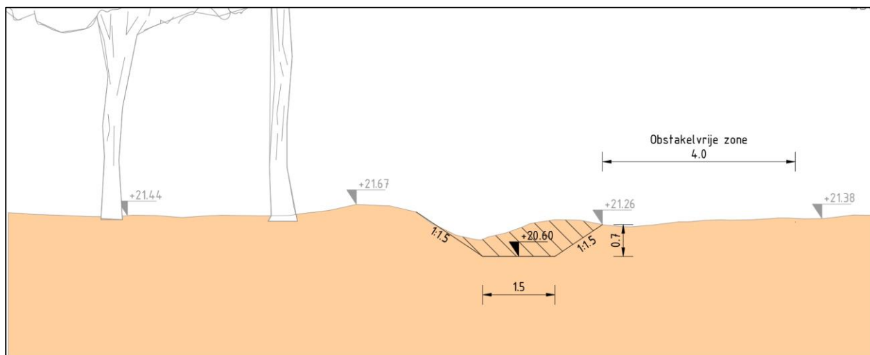
Figuur 26: Principeprofiel (P4) omleiding BZ42 & BZ57 ter hoogte van de op te waardenen OWL10825
