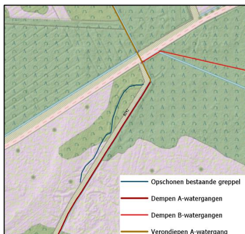
Figuur 57: Op te schonen greppel
