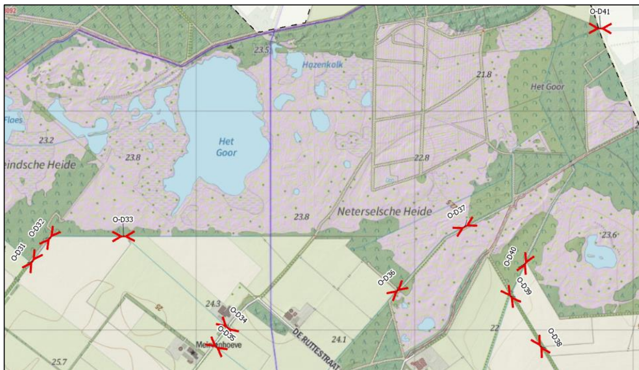
Figuur 34: Overzicht te verwijderen duikers
