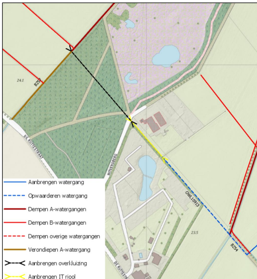
Figuur 27: Overzicht maatregelen rondom overkluizing
