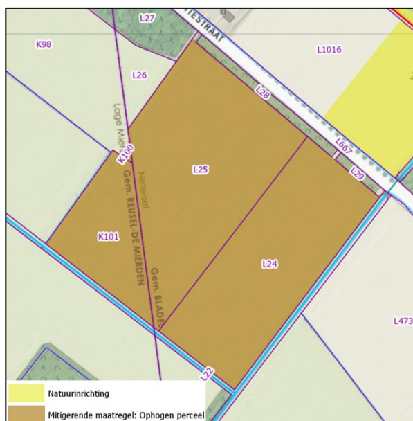
Figuur 41: Ophoging percelen MDE02-K- 101, MDE02-K-100, BDL01-L-25 en BDL01-L-24
