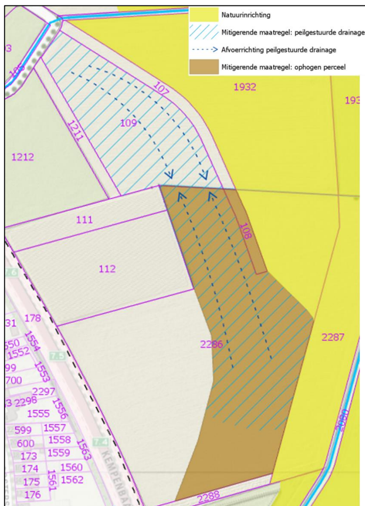
Figuur 18: Overzicht peilgestuurde drainage incl. afwateringrichting t.b.v. mitigatie effecten
