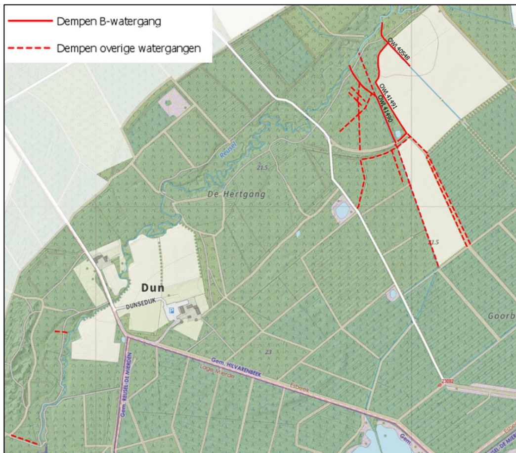
Figuur 43: Overzicht te dempen watergangen
