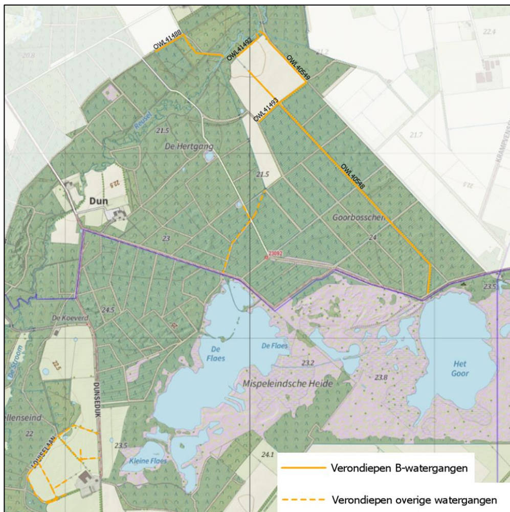
Figuur 44: Overzicht te verondiepen watergangen
