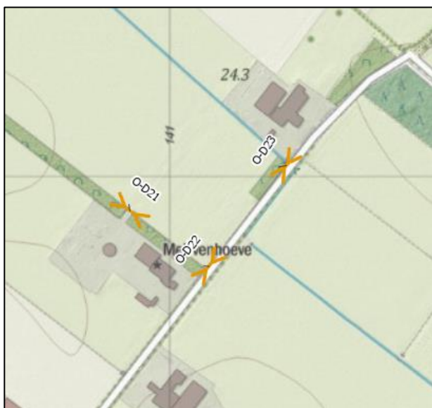
Figuur 33: Overzicht te vervangen duikers
