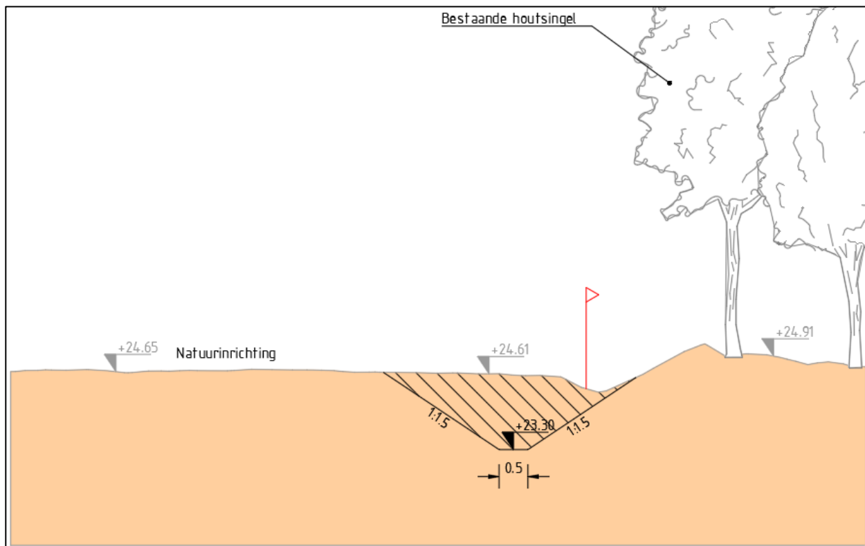
Figuur 21: Principeprofiel P2 omleiding ten zuiden van Mispelindse Heide
