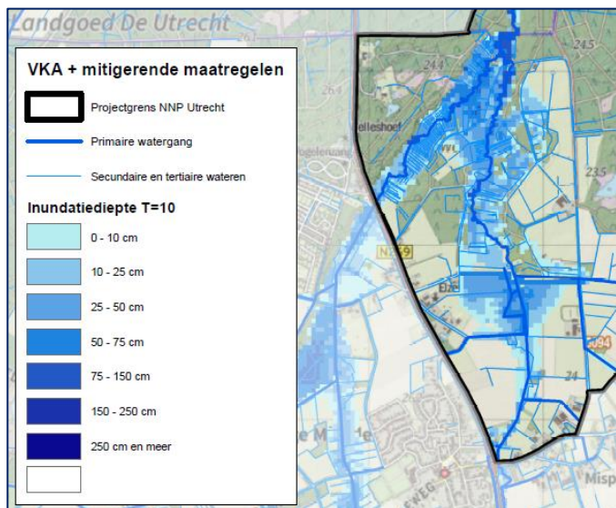
Figuur 63: Uitsnede deelgebied Raamsloop uit Bijlage A8-8. Inundatiediepte Voorkeursalternatief bij piekafvoer die 1x per 10 jaar voorkomt (T=10)
