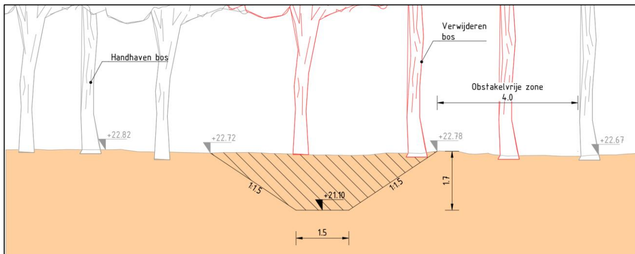
Figuur 25: Principeprofiel (P3) omleiding BZ42 & BZ57 tussen BERE-0329 en Fons van der Heijdenstraat
