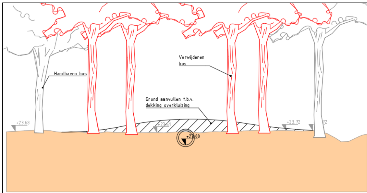
Figuur 28: Principeprofiel aan te brengen overkluizing t.h.v. instroom
