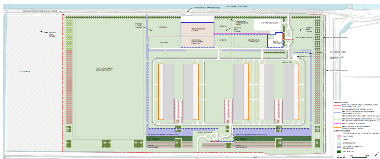
Figuur 3-6 Inrichting van de campus met datacenter, de afbeelding is tevens voor de leesbaarheid opgenomen in Bijlage 1
