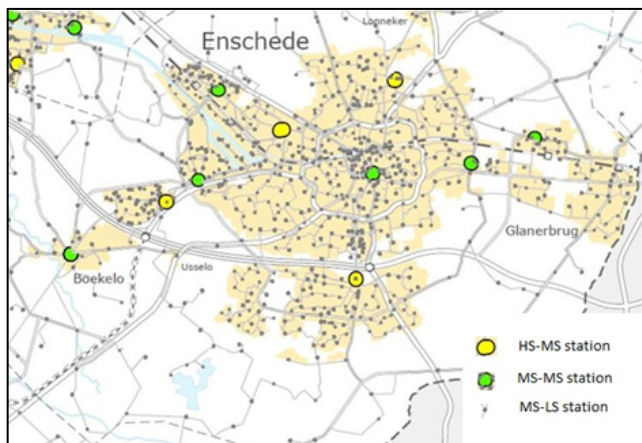
Fig. 3 Netwerkstations Enexis
