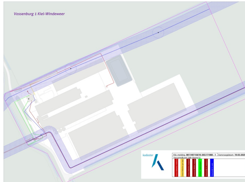
overzicht kabels&leidingen
