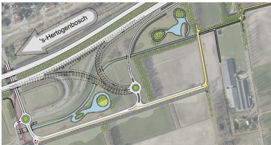
Figuur 3.4 Aansluiting Rekken op aansluiting Nuland zoals in MER / VOBP juni 2019: via huidige wegenstructuur of via een nieuwe rotonde.
