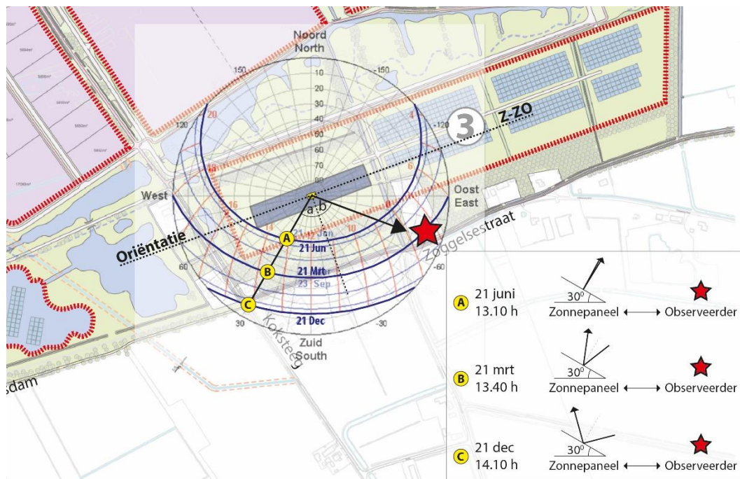
Figuur 10-2 Illustratieve uitwerking mogelijke reflectie op drie momenten (A, B en C (niet gecorrigeerd naar zomer- en wintertijd)) van de zon op een zonnepaneel richting een observeerder (rode ster)
