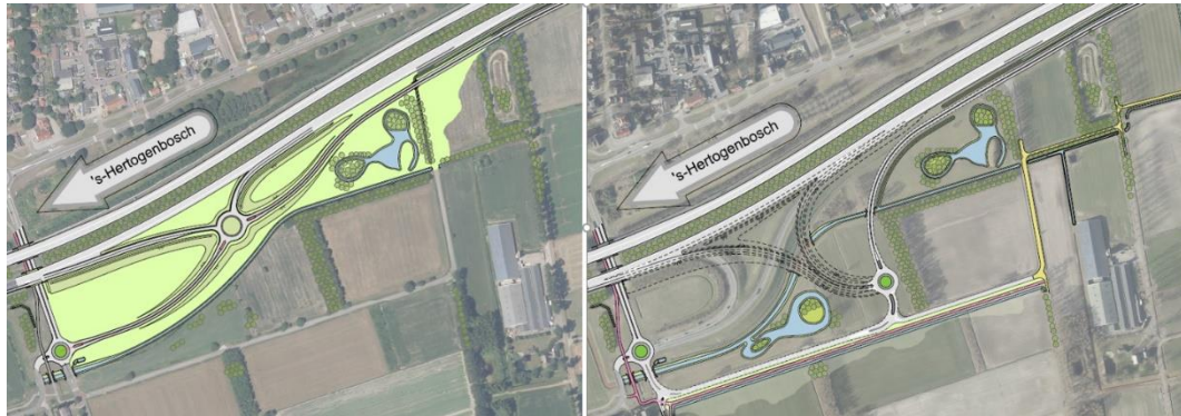
Figuur 15.3 Geoptimaliseerde aansluiting Nuland (links) en het ontwerp uit 2019 (rechts)
