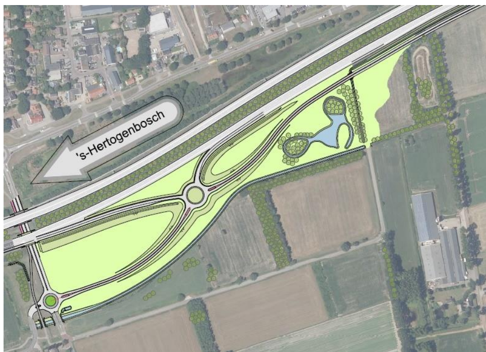
Figuur 3.6 Optimalisatie aansluiting Rekken op aansluiting Nuland in nieuw stedenbouwkundig ontwerp
