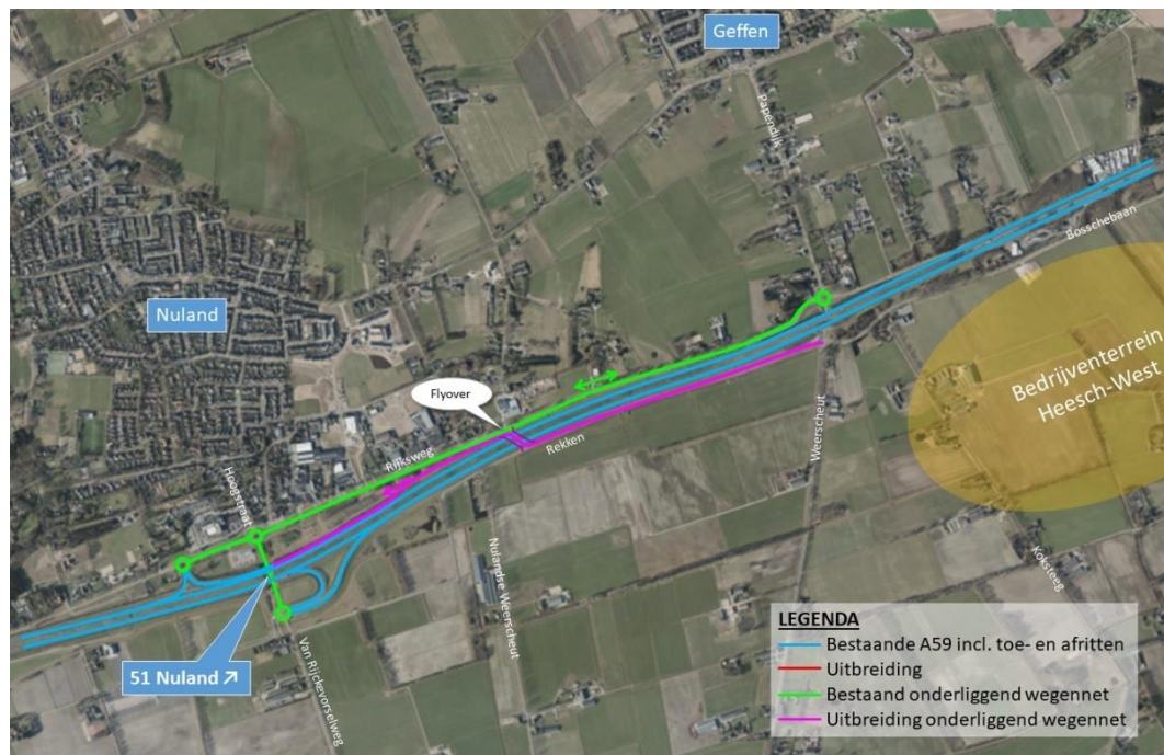
Figuur 3.9 Alternatief 2a Leefbaar Nuland voor aansluiting Rekken op aansluiting Nuland (bron: gemeente Den Bosch)
