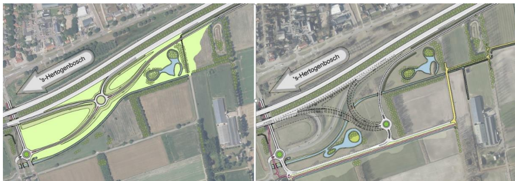
Figuur 14.1 Geoptimaliseerde aansluiting Nuland (links) en het ontwerp uit 2019 (rechts)
