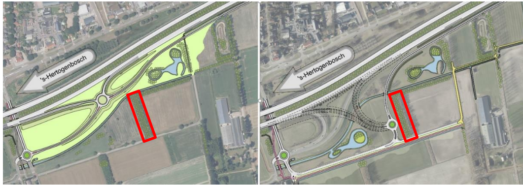
Figuur 17.3 Geoptimaliseerde aansluiting Nuland (links) en het ontwerp uit 2019 (rechts), het nabijgelegen NNB gebied ligt binnen de rode contour.
