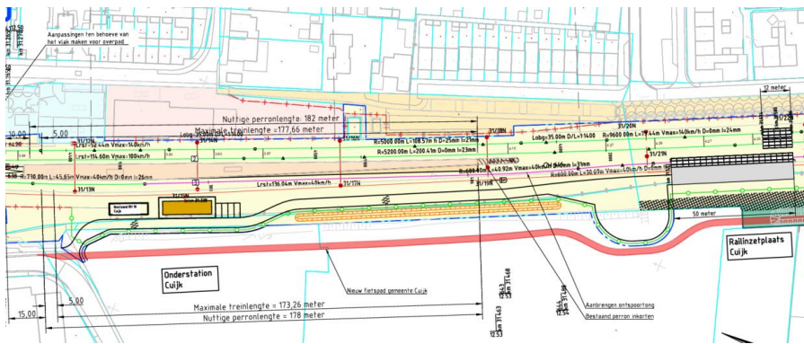
Figuur 3 Ontwerp onderstation en railinzetplaats Cuijk (FIS 3.0)
