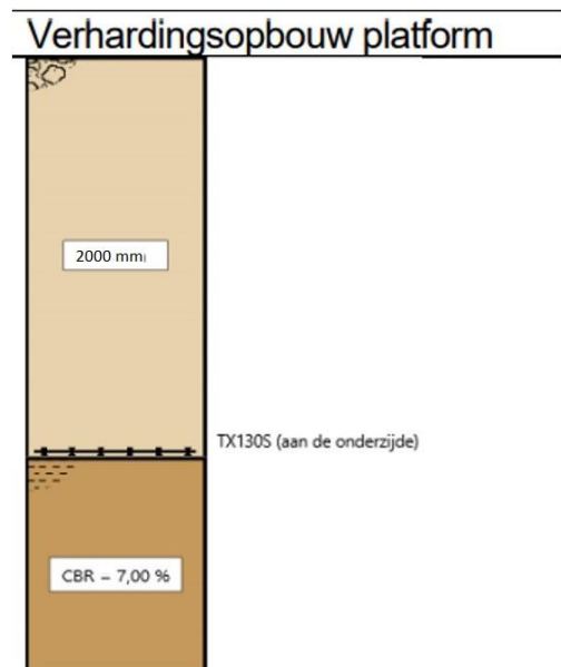
Figuur 3.6 Indicatie opbouw kraanopstelplaatsen
