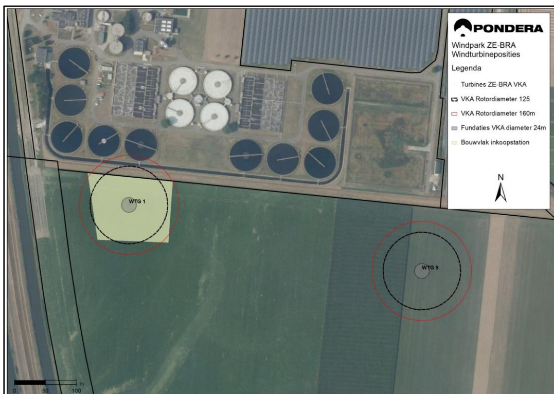
Figuur 3.12 Bouwvlak inkoopstation WT1
