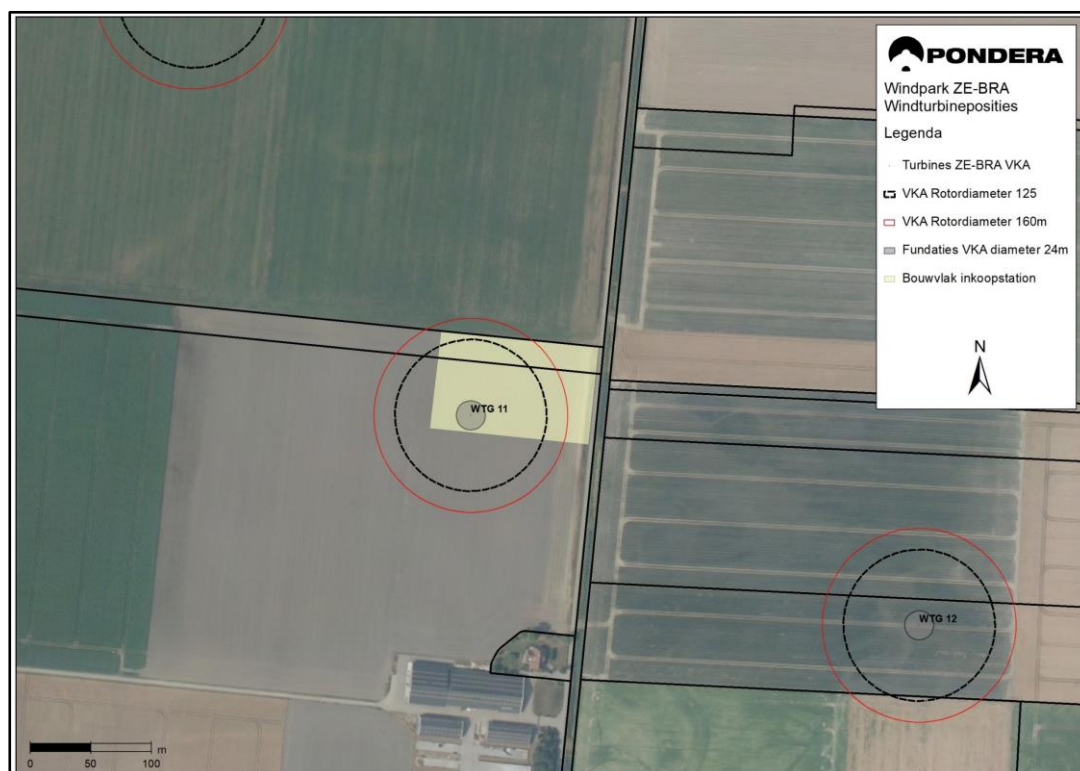
Figuur 3.13 Bouwvlak inkoopstation WT11
