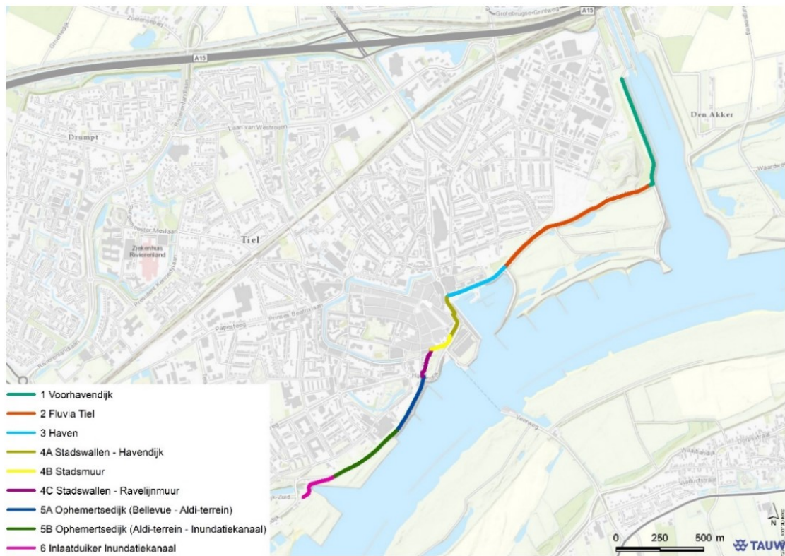
Figuur 1 Ligging dijkversterking Stad Tiel met een kleuraanduiding van de deeltrajecten.
