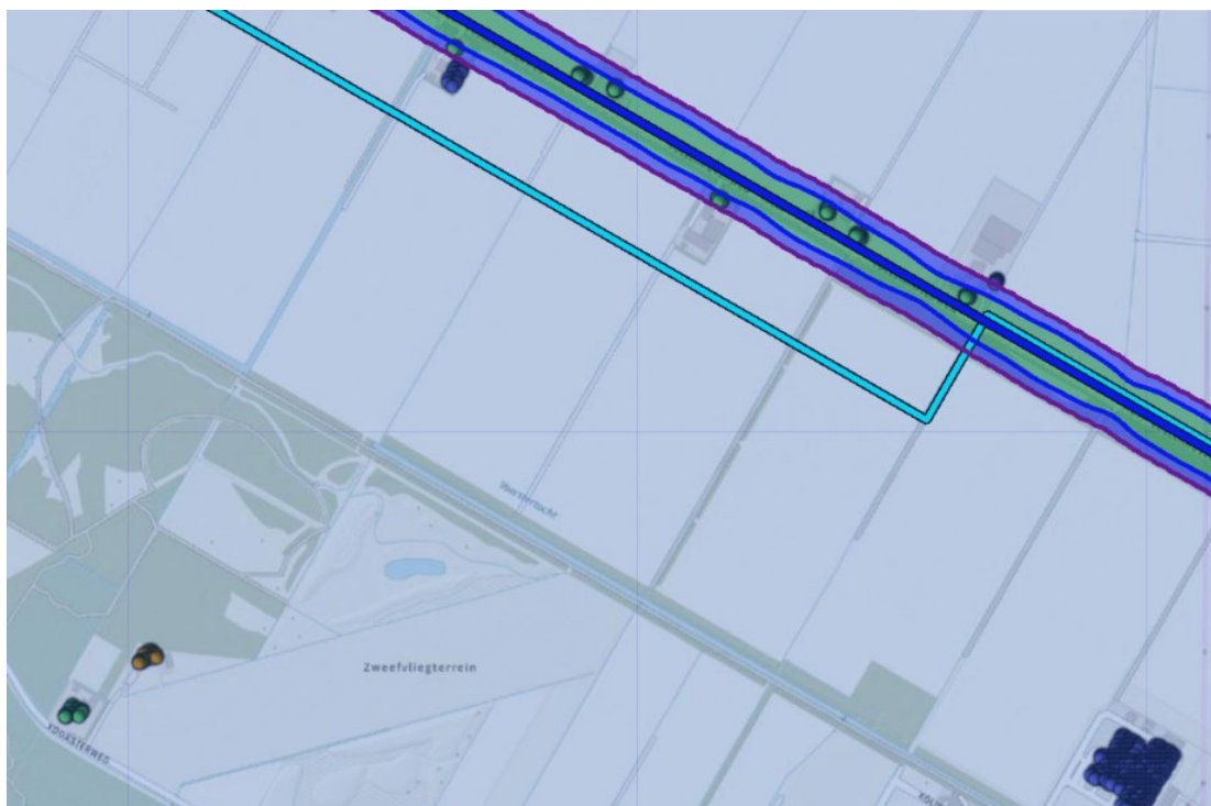
Figuur 4.3 Plaatsgebonden risico voor 6975_leiding-N-500-50-deel-1 excl. verl. (groene gebied = alles binnen PR 10^{-7} contour, blauwe gebied = alles binnen PR 10^{-8} contour)
