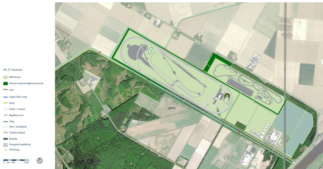
Figuur 2. Inrichtingstekening van het MITC-terrein. Bron: Landschappelijke inpassing MITC Marknesse. VISTA, 4 oktober 2021
