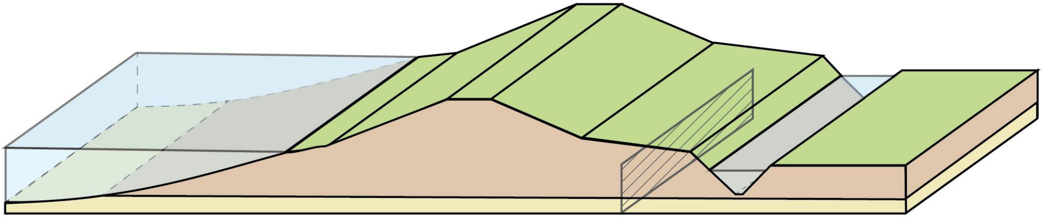
Filbertechniek: verticaal filterscherm
