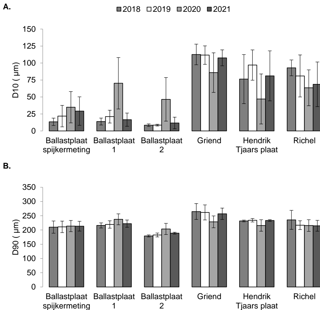
Figuur 3-3 Overzicht veranderingen in A) gemiddelde korrelgrootte D_{10} ( \mu\text{m} ) en B) gemiddelde korrelgrootte D_{90} ( \mu\text{m} ) en bijbehorende standaarddeviaties voor 2018, 2019, 2020 op de Ballastplaat Spijkermeting (spijkermeting locaties), Ballastplaat 1 (bodemdalingengebied 1), Ballastplaat 2 (referentiegebied 2), Griend (referentiegebied B), Hendrik Tjaarsplaat (referentiegebied 3) en Richel (referentiegebied A).
