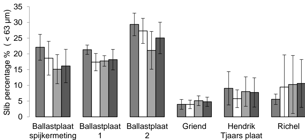
Figuur 3-1 Overzicht veranderingen in A) gemiddelde korrelgrootte (µm) en B) gemiddeld slib percentage (% < 63 µm) en bijbehorende standaarddeviaties voor 2018, 2019, 2020 en 2021 op de Ballastplaat Spijkermeting (spijkermeting locaties), Ballastplaat 1 (bodemdalingsgebied 1), Ballastplaat 2 (referentiegebied 2), Griend (referentiegebied B), Hendrik Tjaarsplaat (referentiegebied 3) en Richel (referentiegebied A).
