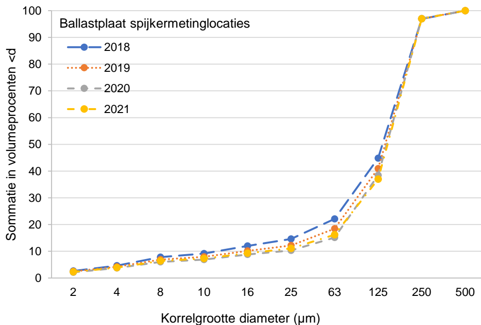
Figuur 3-2 Gemiddelde cumulatieve korrelgrootteverdeling voor 2018, 2019, 2020 en 2021 op de Ballastplaat voor de spijkermeting locaties. Op de x-as is de korrelgrootte (diameter in \mu\text{m} ) weergegeven. Op de y-as is het cumulatieve volume-percentage van de gevonden volumes weergegeven, beginnend bij de kleinste korrelafmeting.
