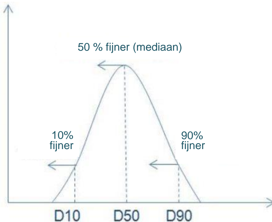
Figuur 2-4 Overzichtsfiguur cumulatieve percentielwaarden: 90% van de korrelgrootteverdeling van een sedimentmonster ligt onder D 90 , 50% ligt onder de D 50 (mediaan), en 10% ligt onder de D 10 . Figuur gebaseerd op Azom, Palani D.
