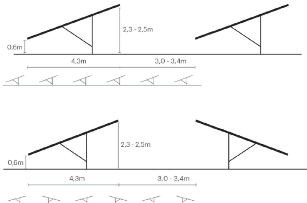
Figuur 4.4: Twee voorbeeld opstellingen zonnepanelen
