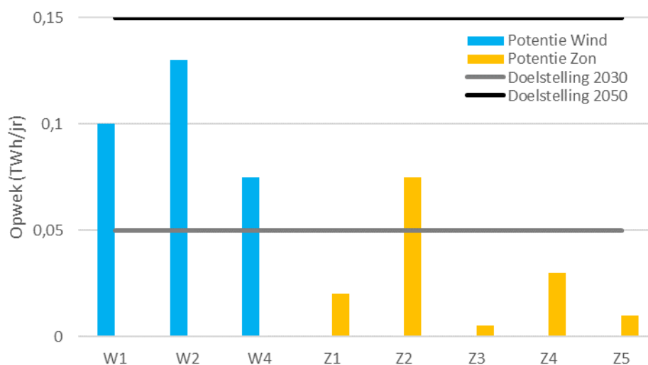
Figuur 6 Opwekpotentie per zoekgebied. Gegevens op basis van het planMER.
