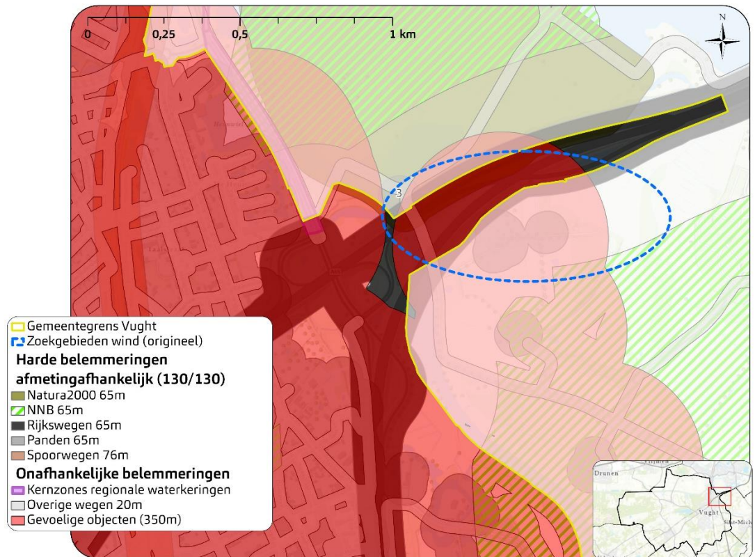
Figuur 4 Harde belemmeringen rond en in windzoekgebied 3
