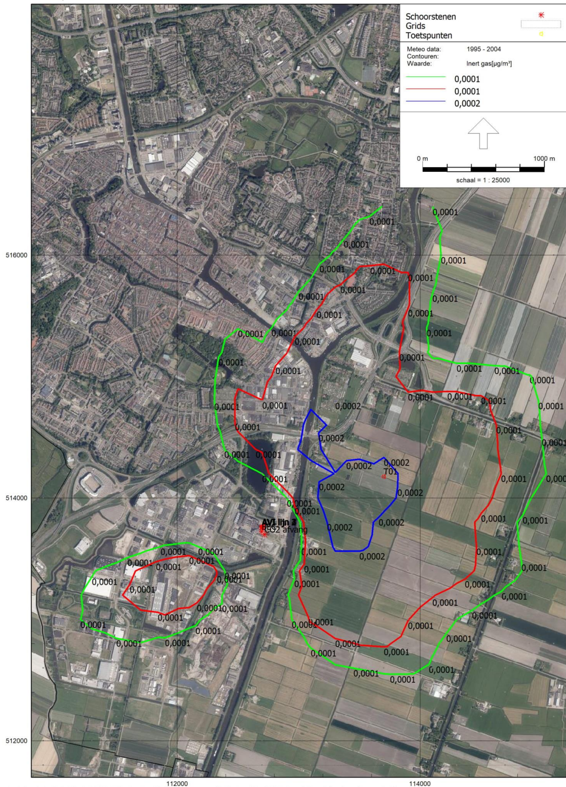
Figuur w Jaargemiddelde concentraties \Sigma zware metalen (0,00010; 0,00012 en 0,00020 \mu\text{g}/\text{m}^3 ): BEC -> CO 2 -afvanginstallatie
