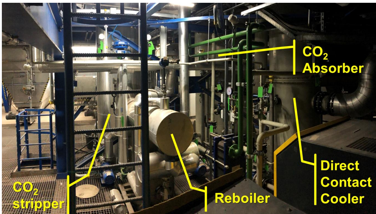
Figuur 10, Afvang installatie (1e verdieping RGR gebouw BEC)
