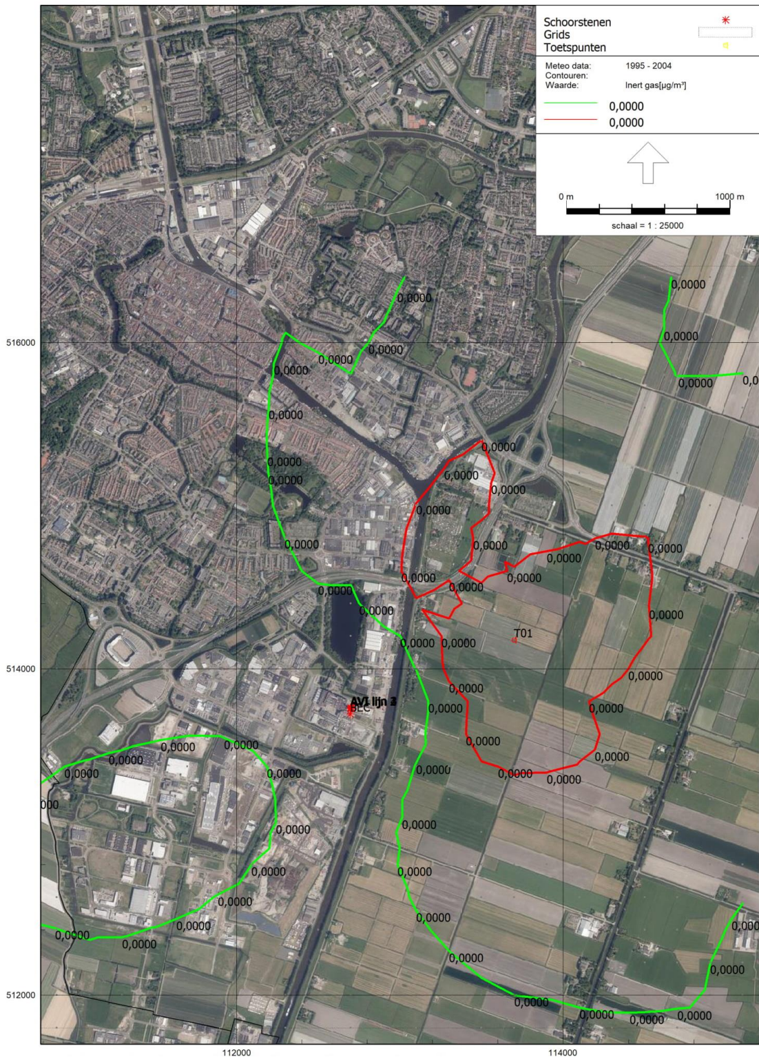
Figuur p Jaargemiddelde concentraties Hg (0,00001 en 0,00002 µg/m 3 ) in de vergunde situatie
