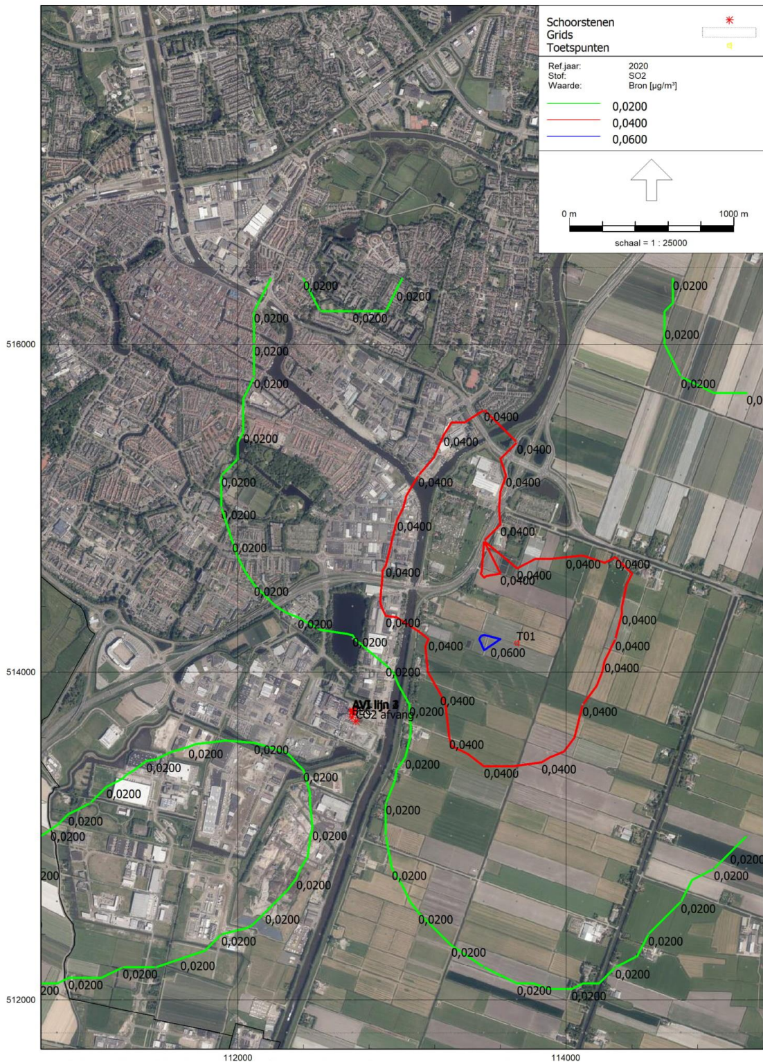
Figuur I Jaargemiddelde concentraties \text{SO}_x ( \mu\text{g}/\text{m}^3 ): Lijn 4 -> \text{CO}_2 -afvanginstallatie
