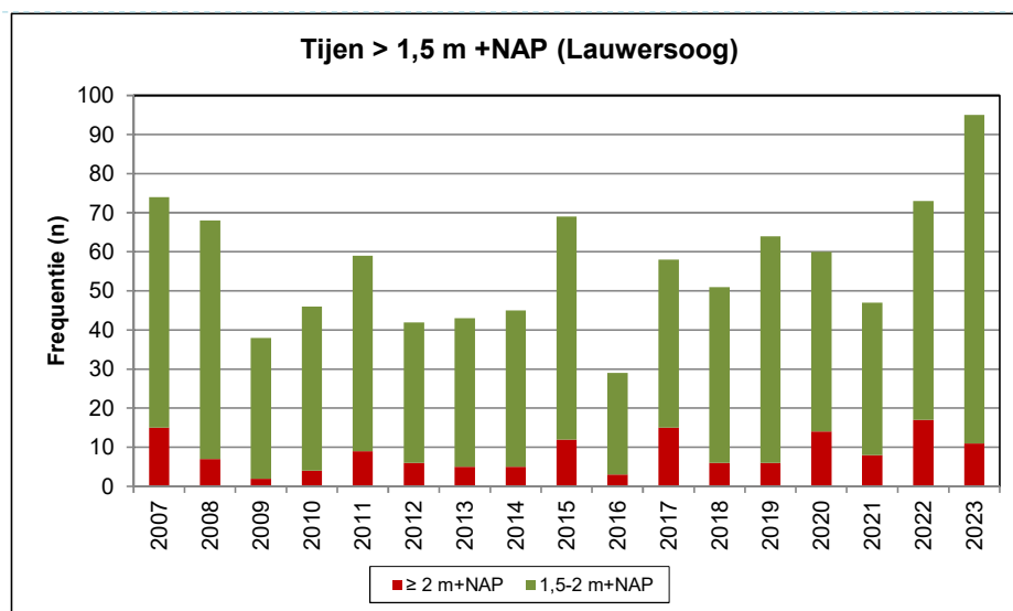
Figuur 3.15 Aantal tijen >1,5 m +NAP voor Lauwersoog van 2007-2023 op basis van RWS-data.
