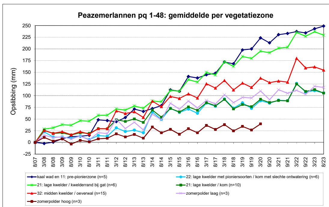
Figuur 3.1 Gemiddelde cumulatieve netto-opslibbing (mm) per vegetatiezone (met SALT97 code) in de kwelder en deelgebied in de zomerpolder op basis van SEB-metingen in de Peazemerlannen van 2007-2023. Data betreffende de zomerpolder-hoog vanaf 9/20 ontbreken wegens het afmaaien van de SEB-palen.
