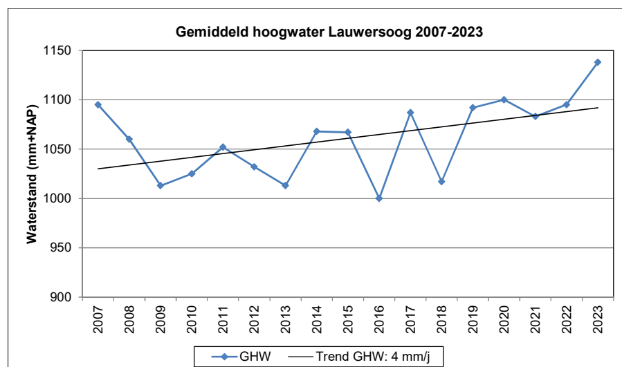
Figuur 3.14 Jaargemiddelde hoogwater en trendlijn van 1988-2023 en van 2007-2023 op basis van hoogwater-data van Rijkswaterstaat voor Lauwersoog.
