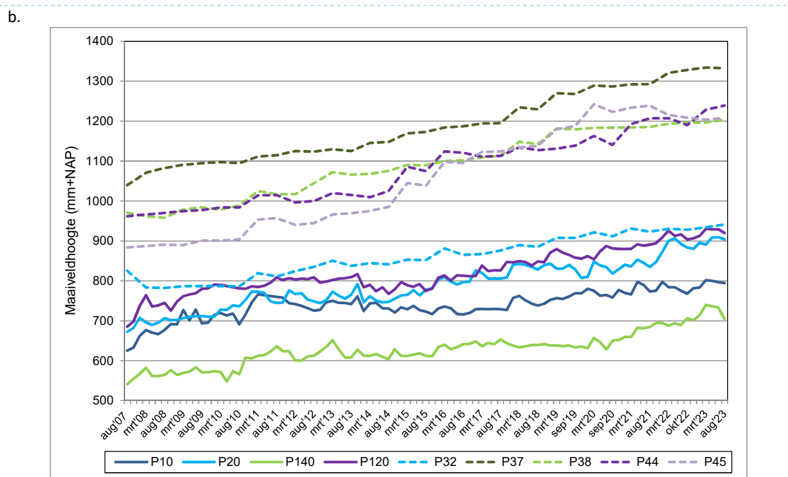
Figuur 3.4a Vergelijking van de opslibingsmetingen van NCA en Artemisia op de overgang van wad naar kwelder bij de Peazemerlannen over de periode aug. 2007- aug. 2023. De P met nummer betreft het meetpunt en het getal achter de stip de opslibing in mm/j (Kaart gemaakt door NCA; zie ook Krol et al., 2024); b. De ontwikkeling van de maaiveldhoogte (mm+NAP) bij de meetpunten van ca. aug. 2007-aug. 2023. De doorgetrokken lijnen betreffen de NCA-meetpunten en de gestippelde lijnen de Artemisia-meetpunten. De meetpunten die bij elkaar in de buurt liggen hebben vergelijkbare kleuren.
