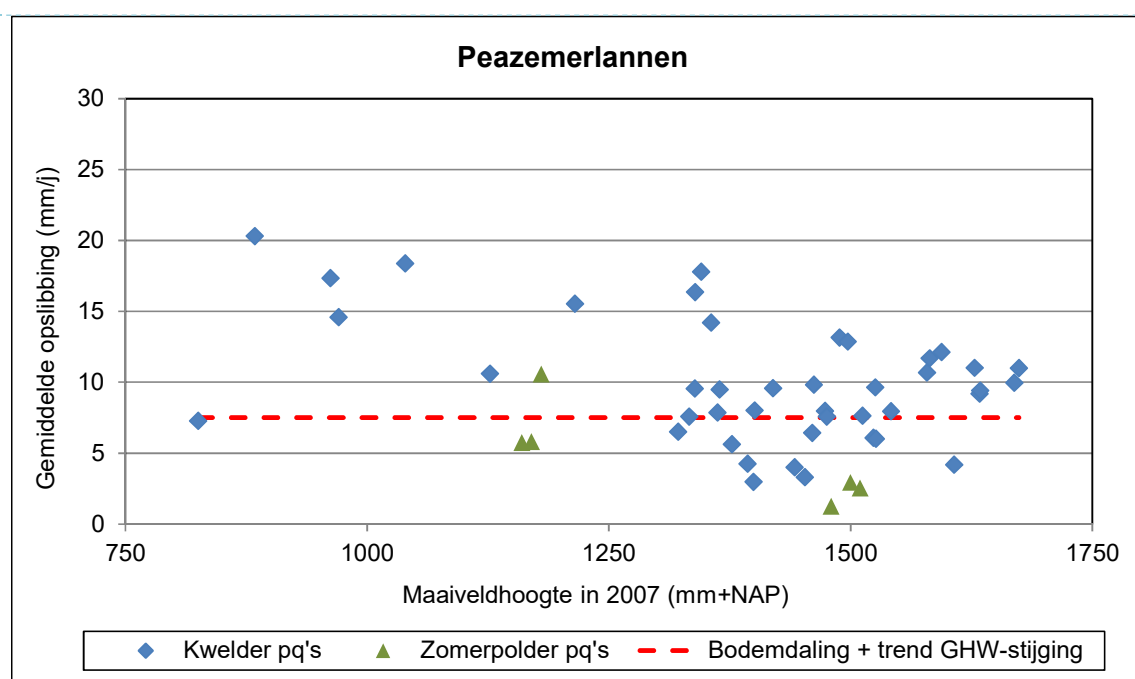
Figuur 3.2 Gemiddelde netto-opslibbing in mm/j per pq over de periode 2007-2023 in de Peazemerlannen. De rode stippellijn geeft de gemiddelde jaarlijkse bodemdaling over de periode 2007 t/m 2023 van 3,5 mm/j (zie ook Figuur 1.3) + de trend in GHW-stijging van 4 mm berekend voor Lauwersoog over de periode 2007 t/m 2023 (zie Figuur 3.14).
