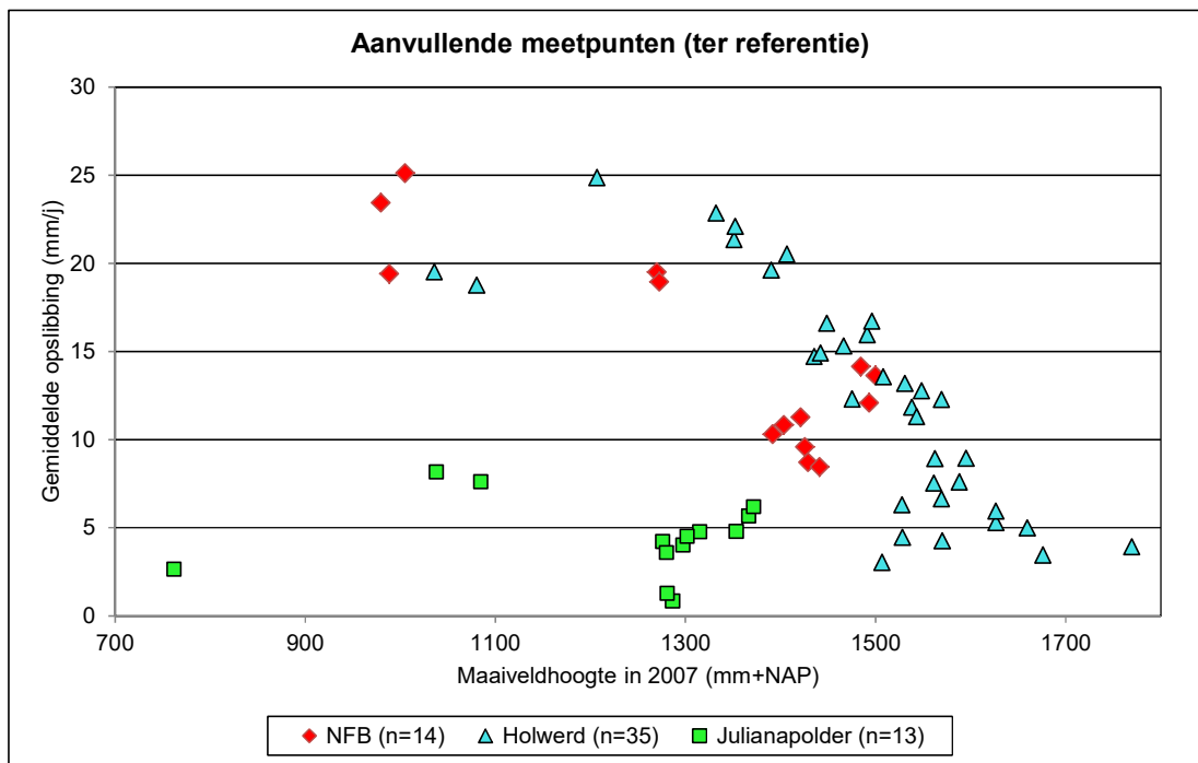
Figuur 3.8 Gemiddelde netto-opslibbing in mm/j per kwelder-pq (inclusief pq's in de pionierzone) over de periode 2007-2023 in de aanvullende meetpunten ter referentie in de deelgebieden Noord-Friesland Buitendijks (NFB), Holwerd (Fr.) en Julianapolder (Gr.).
