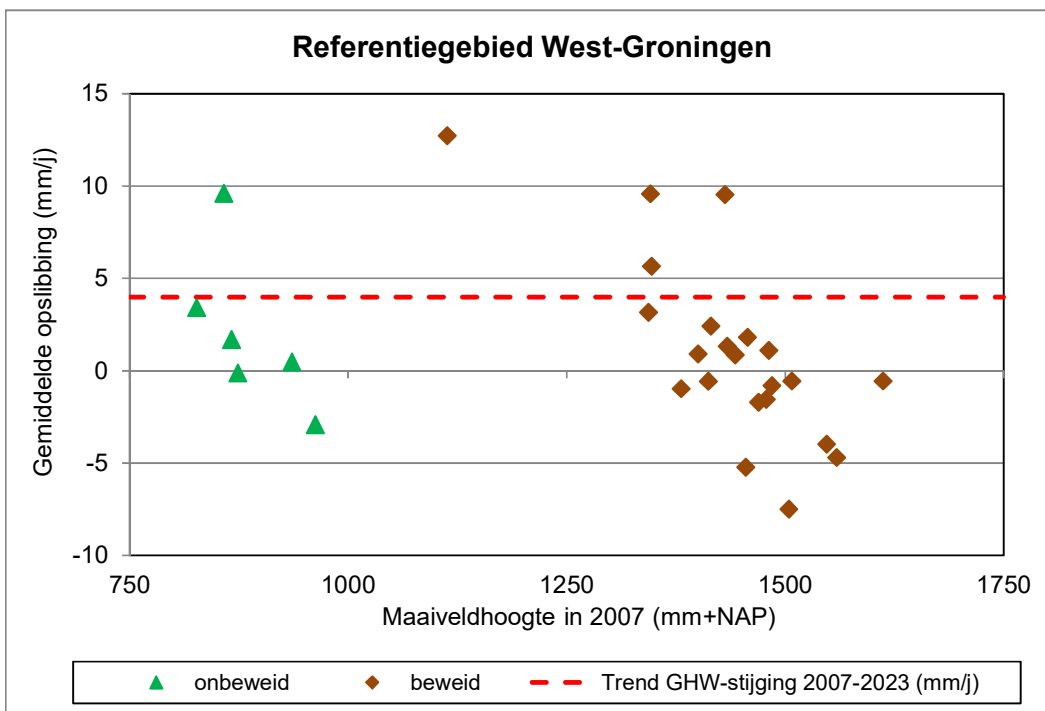
Figuur 3.7 Gemiddelde netto-opslibbing in mm/j per kwelder-pq (inclusief pq's in de pionierzone) over de periode 2007-2023 in het referentiegebied West-Groningen. De rode stippellijn geeft de gemiddelde trend in GHW-stijging van 4 mm berekend voor Lauwersoog over de periode 2007 t/m 2023 (zie Figuur 3.14). Alleen de onbegroeide pq's op het wad zijn nog onbeweid.
