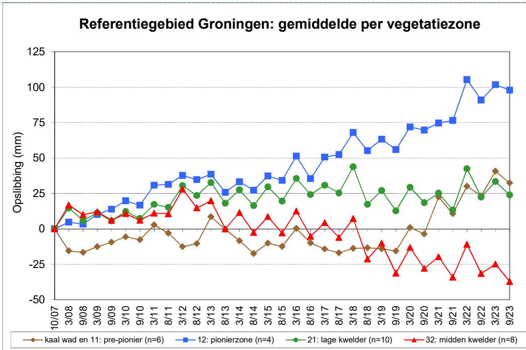
Figuur 3.6 Gemiddelde cumulatieve netto-opslibbing (mm) per vegetatiezone (met SALT97 code) op basis van de SEB-metingen in het referentiegebied West-Groningen van 2007-2023.
