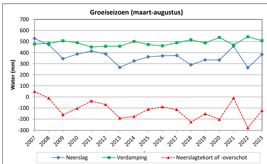
Figuur 3.16 Neerslag, verdamping en neerslagtekort in het groeiseizoen (maart t/m augustus) voor Lauwersoog (station 277) van 2007-2023 op basis van KNMI-gegevens.
