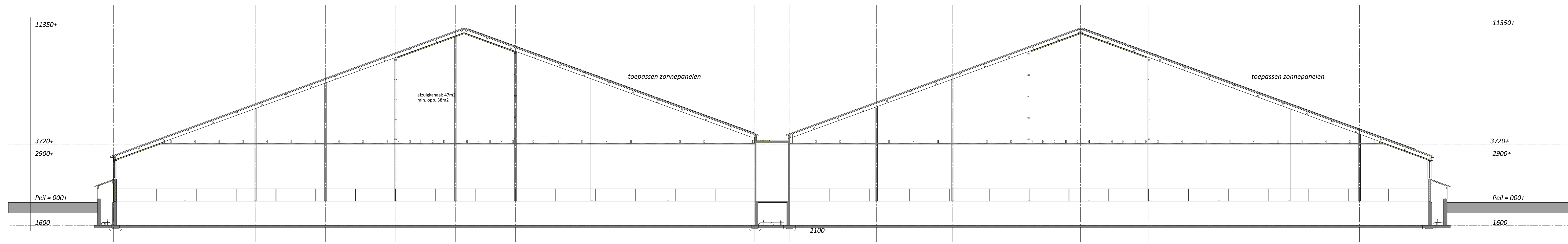
Doorsnede B-B
