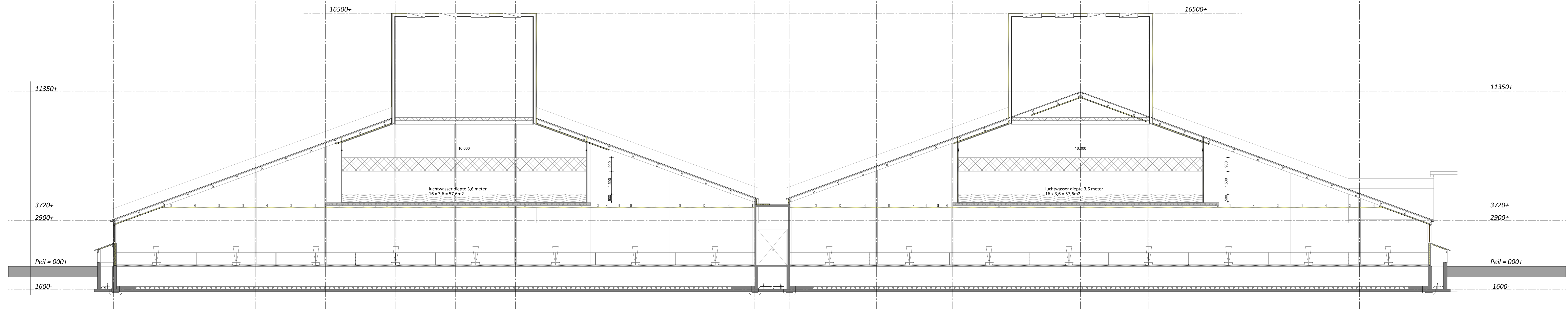
Doorsnede C-C
