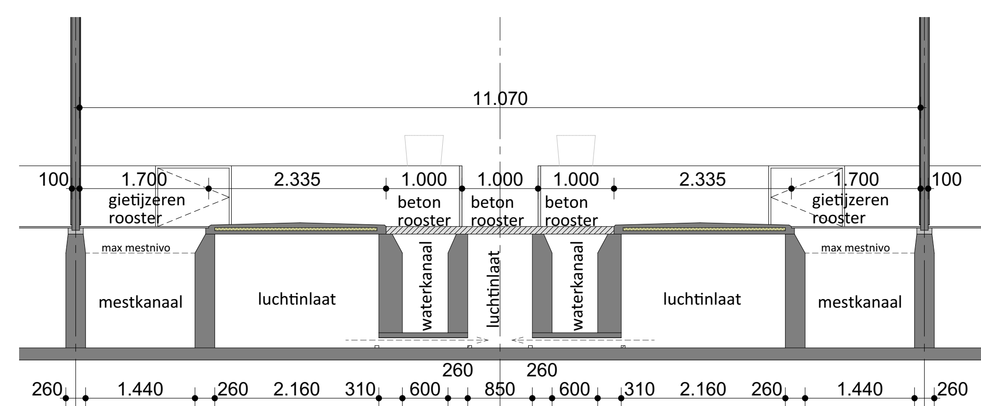
Doorsnede D-D afdeling
