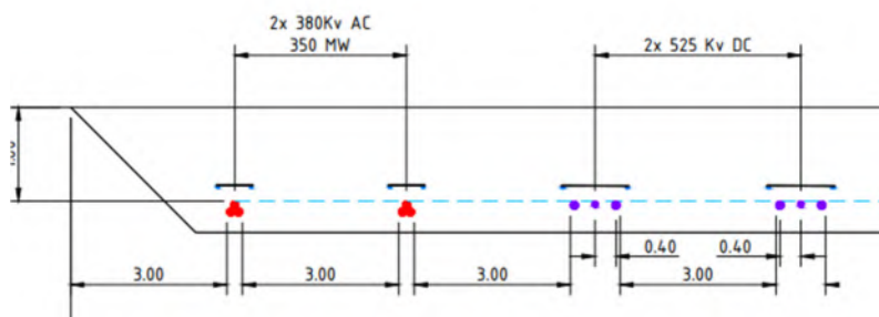
Figuur 7 - Kabelcorridor cross section 3 voor 4,7 GW scenario.
