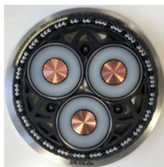
AC-kabelsysteem op zee
