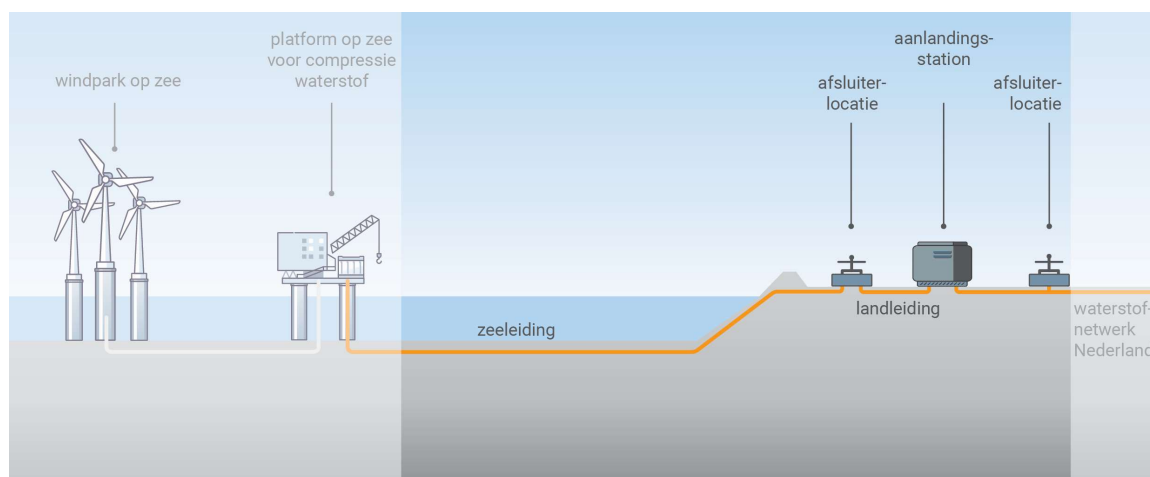
Afbeelding 4.2 Schematische weergave van een waterstofverbinding
