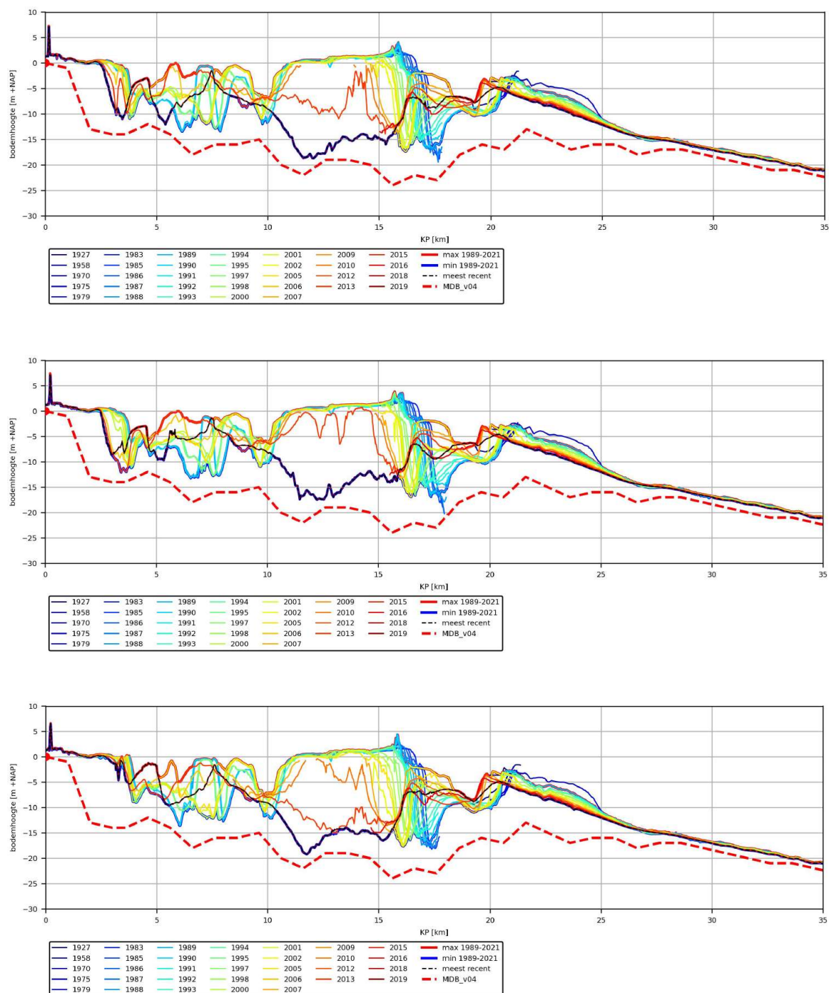
Afbeelding 3.117 Morfologisch ontwerp-profiel (rood gestippelde lijn) en waargenomen bodemligging langs route A2 door de jaren van 1927 t/m 2020. Van boven naar beneden: middenlijn, zijlijn oost en zijlijn west
