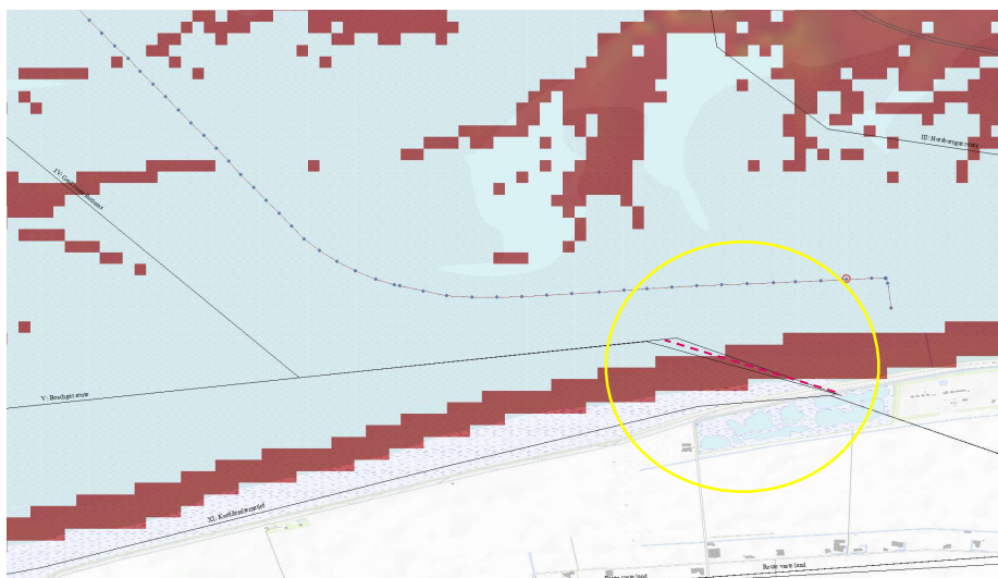
De leiding kan vanaf de kruising van de zeewering met een legschip verder richting offshore gelegd worden. Om installatie met legschip mogelijk te maken voor deze route is veel baggerwerk noodzakelijk in de delen met geringe waterdiepte voor de toegang van het legschip en aanvullend baggerwerk om de leiding op voldoende diepte te brengen, ten aanzien van dit aspect is de route vergelijkbaar met Route III.
