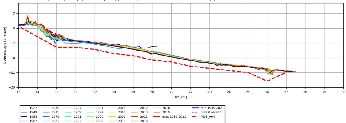
Afbeelding 3.143 Waargenomen bodemligging langs zijlijn west (1500 m) van route VII variant A door de jaren van 1927 t/m 2019 (KP 13,0-30,0). Rode gestippelde lijn: het morfologisch ontwerpprofiel
