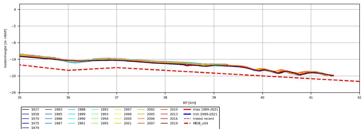
Afbeelding 3.106 Waargenomen bodemligging langs zijlijn west van route V variant A1 door de jaren van 1927 t/m 2019 (KP 35,0-42,0). Rode gestippelde lijn: het morfologisch ontwerpprofiel
