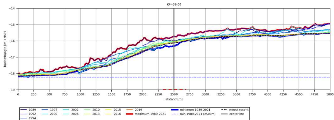
Afbeelding 3.107 Waargenomen bodemligging dwars op middenlijn van route V variant A1 door de jaren van 1989 t/m 2019 (KP 39,0). Rode gestippelde lijn: het morfologisch ontwerpprofiel
