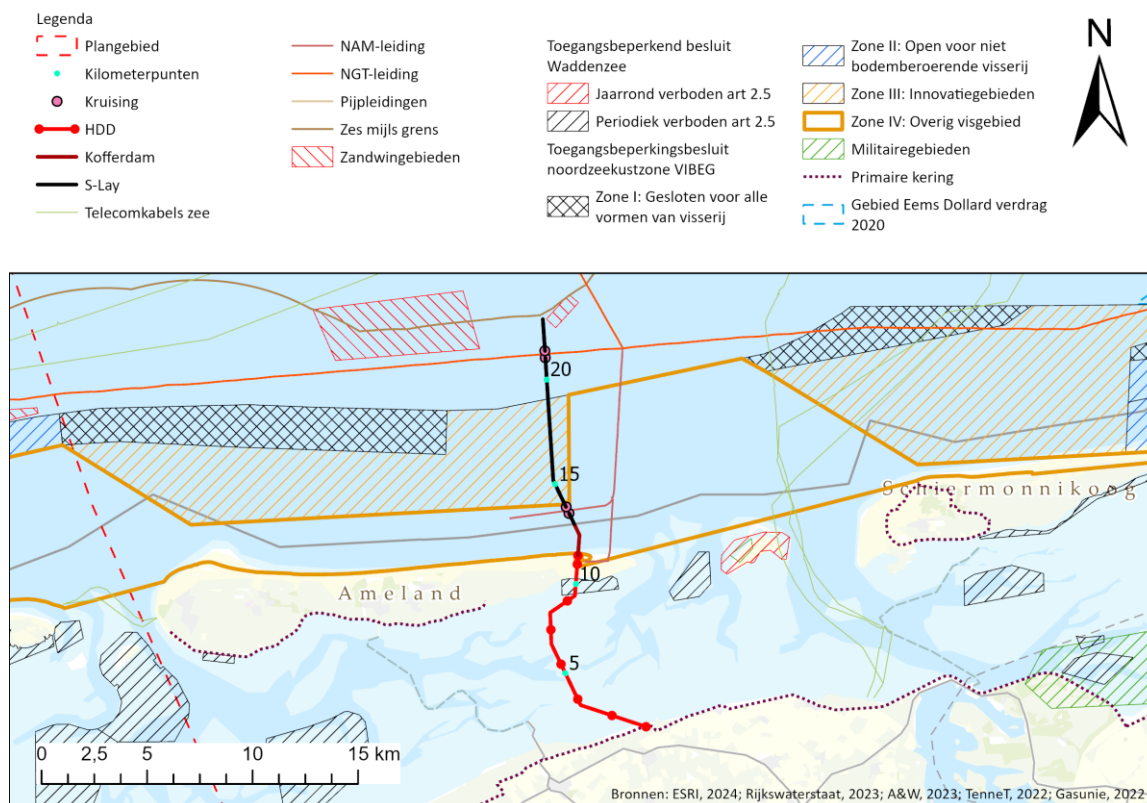
Abbeelding 12.3 Routeontwerp leiding (Baseline 3), serie HDD-boringen, VIII: Ameland Wantij route.
