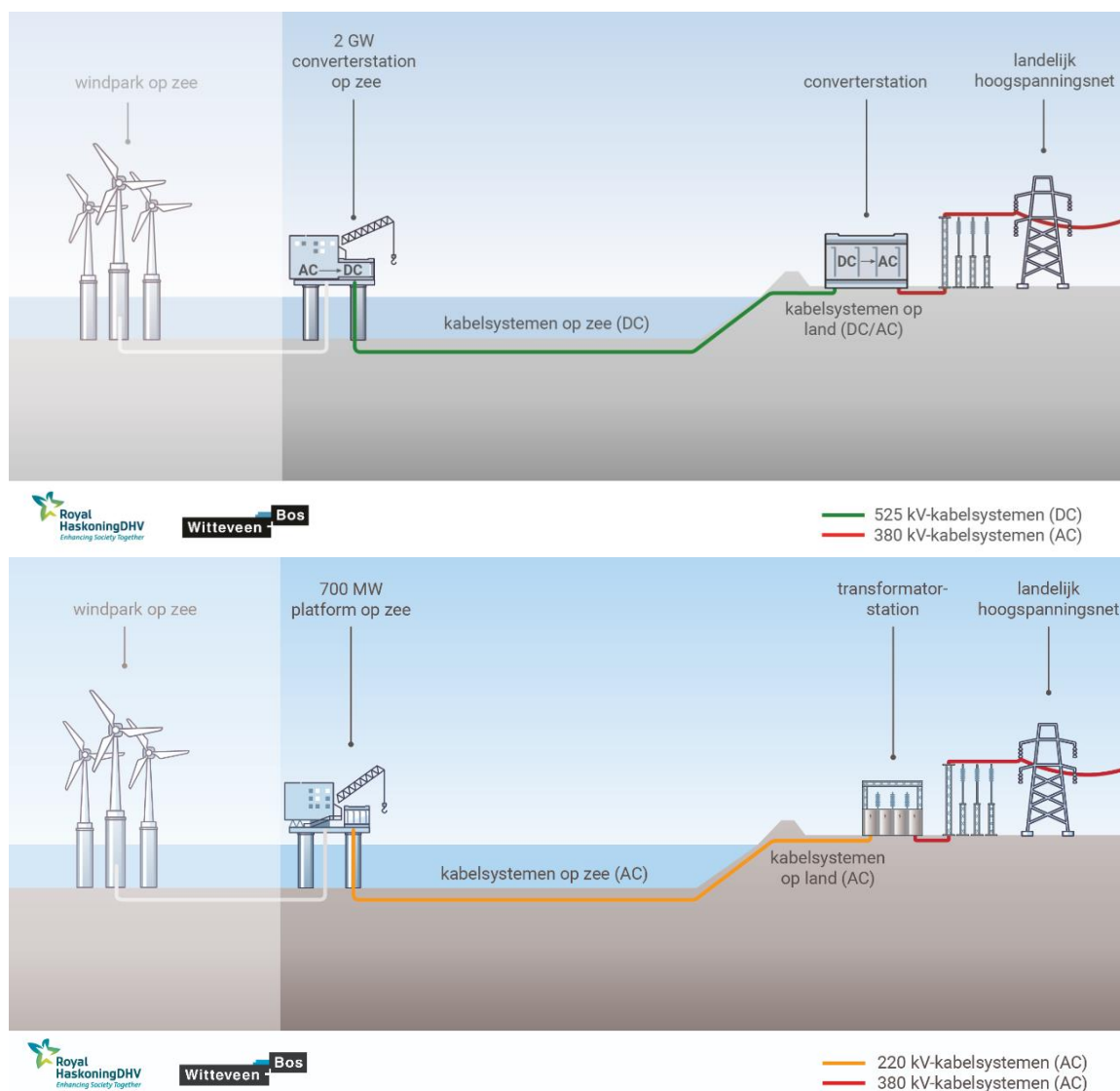
Afbeelding 3.1 Schematische weergave van het elektriciteitsnet (boven: gelijkstroom (DDW), onder: wisselstroom (TNW))
