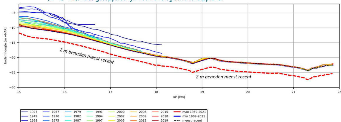
Afbeelding 3.218 Waargenomen bodemligging langs zijlijn oost van route IX variant 'A1' door de jaren van 1983 t/m 2020 (KP 15 - 22). Rode gestippelde lijn: het morfologisch ontwerpprofiel
