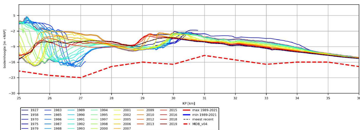
Afbeelding 3.94 Waargenomen bodemligging langs zijlijn west van route V variant A door de jaren van 1927 t/m 2019 (KP 25,0-36,0). Rode gestippelde lijn: het morfologisch ontwerpprofiel
