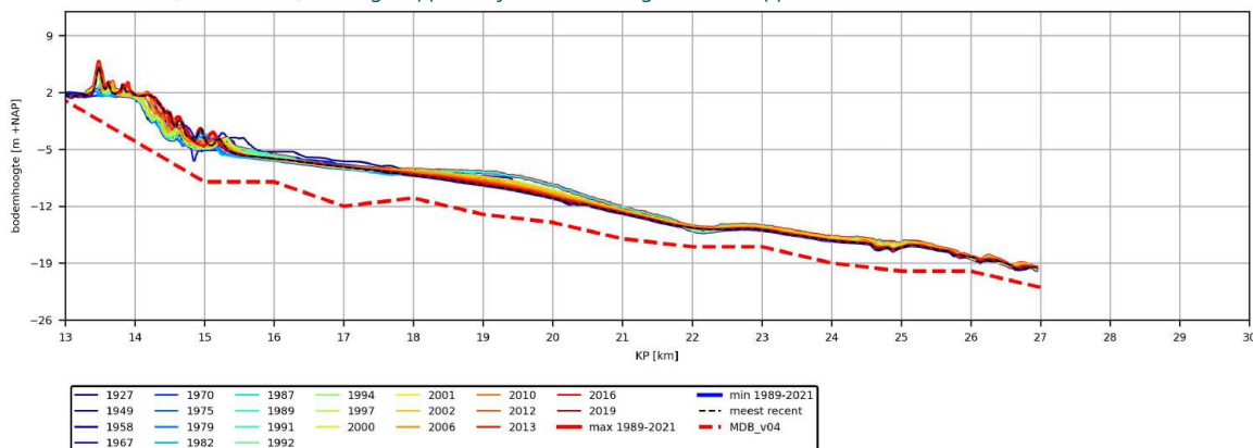
Afbeelding 3.148 Waargenomen bodemligging langs zijlijn west van route VII variant A1 door de jaren van 1927 t/m 2019 (KP 13,0-30,0). Rode gestippelde lijn: het morfologisch ontwerpprofiel
