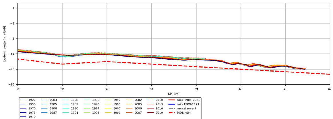
Afbeelding 3.104 Waargenomen bodemligging langs de middenlijn van route V variant A1 door de jaren van 1927 t/m 2019 (KP 35,0-42,0). Rode gestippelde lijn: het morfologisch ontwerpprofiel
