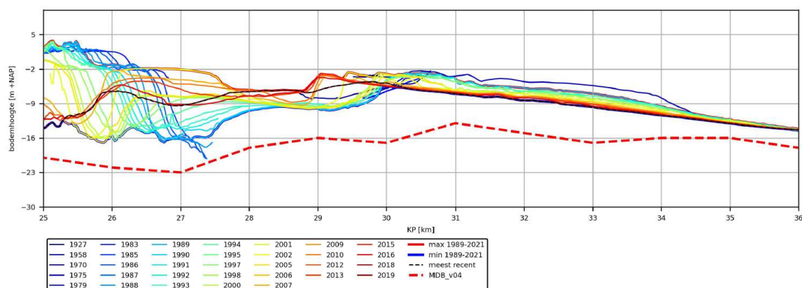
Afbeelding 3.93 Waargenomen bodemligging langs zijlijn oost van route V variant A door de jaren van 1927 t/m 2019 (KP 25,0-36,0). Rode gestippelde lijn: het morfologisch ontwerpprofiel
