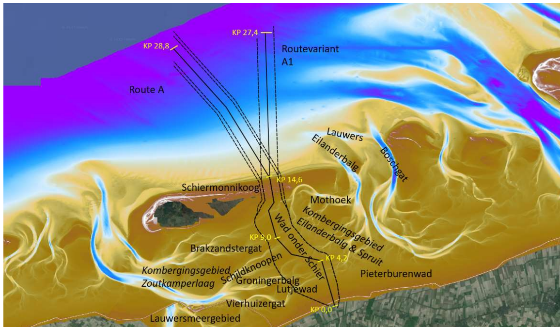
Afbeelding 3.118 Bovenaanzicht en langspiegel route VII (Schiermonnikoog wantij) incl. geulen, platen, kwelders langs route VII
