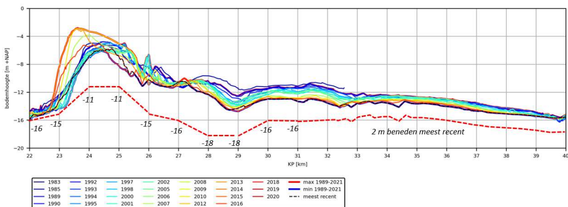
Afbeelding 3.48 Waargenomen bodemligging langs de middenlijn van route II variant TenneT-A door de jaren van 1983 t/m 2020 (KP 22 - 40). Rode gestippelde lijn: het morfologisch ontwerpprofiel
