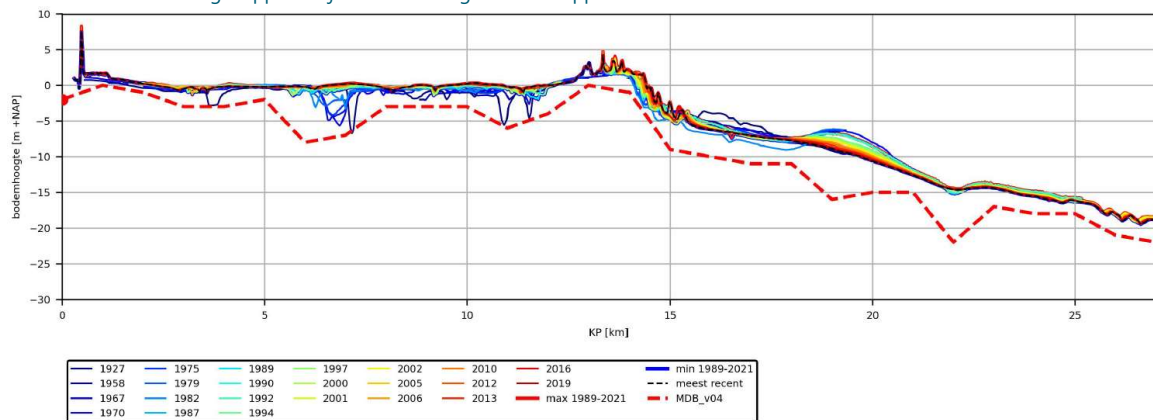
Afbeelding 3.157 Waargenomen bodemligging langs de middenlijn van route VII variant A1 door de jaren van 1927 t/m 2019. Rode gestippelde lijn: het morfologisch ontwerpprofiel
