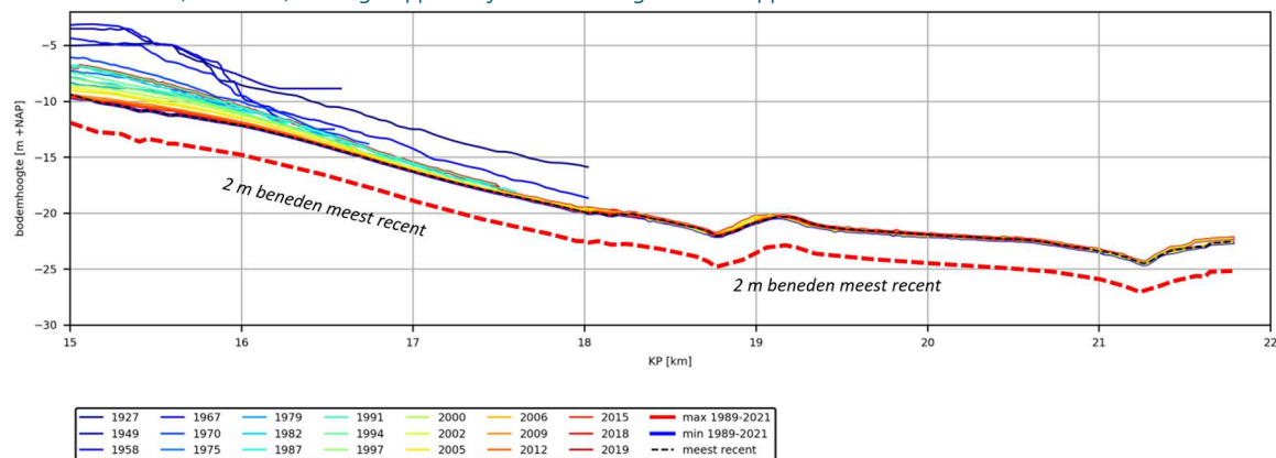
Afbeelding 3.217 Waargenomen bodemligging langs de middenlijn van route IX variant 'A1' door de jaren van 1983 t/m 2020 (KP 15 - 22). Rode gestippelde lijn: het morfologisch ontwerpprofiel
