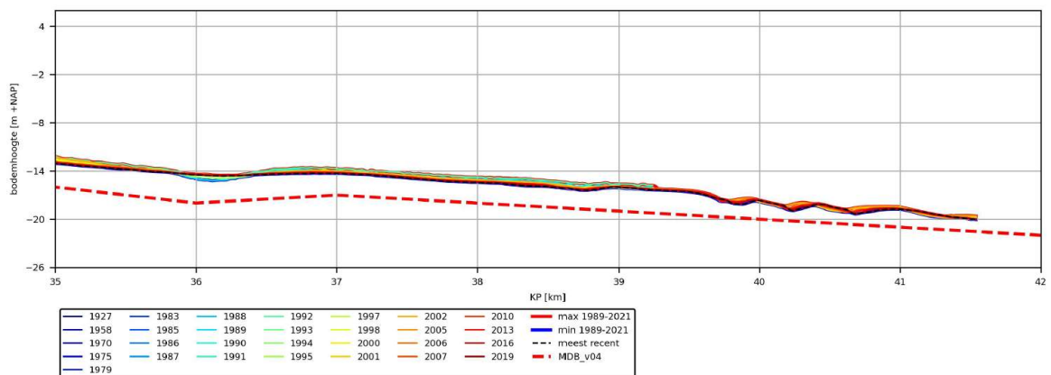
Afbeelding 3.105 Waargenomen bodemligging langs zijlijn oost van route V variant A1 door de jaren van 1927 t/m 2019 (KP 35,0-42,0). Rode gestippelde lijn: het morfologisch ontwerpprofiel
