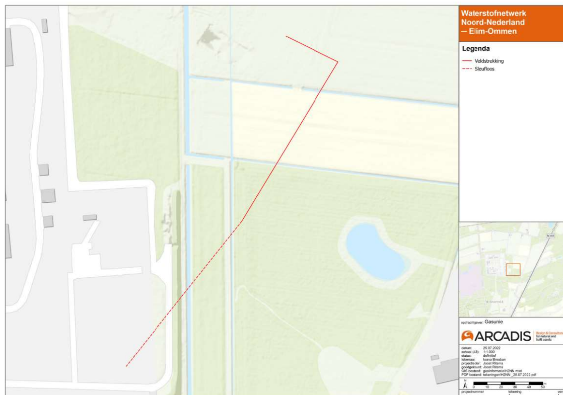
Figuur 2: Tracédeel Elim-Ommen, aanlegmethoden.
